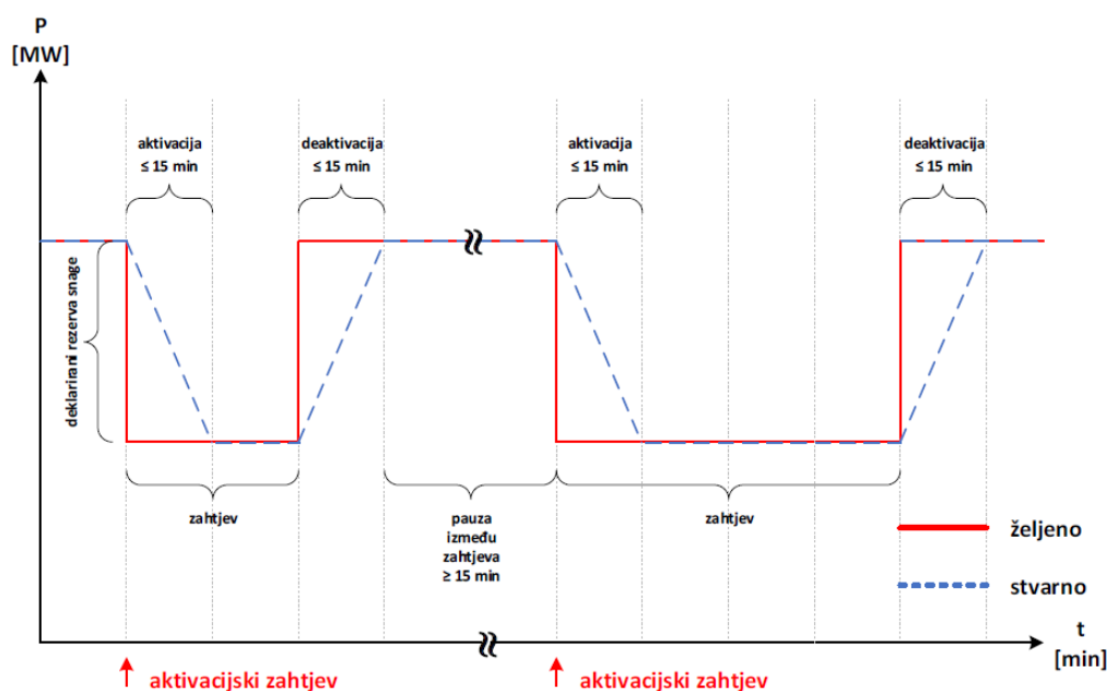
Slika 1 Procedura testiranja
