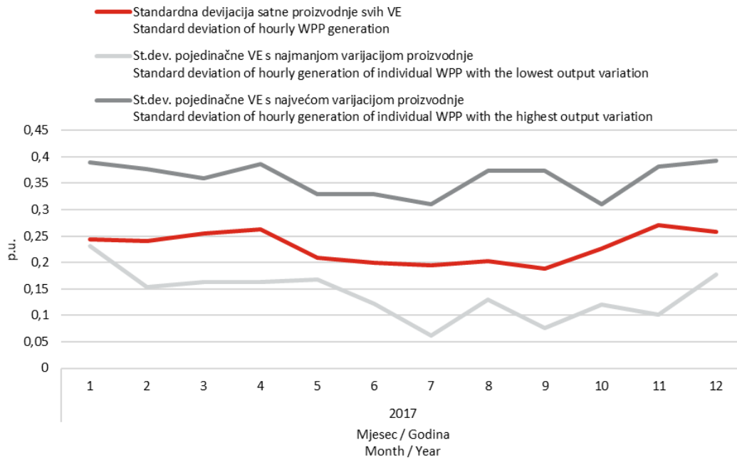
Slika 5 Standardna devijacija satne proizvodnje vjetroelektrana u jediničnim vrijednostima Figure 5 Standard deviation of hourly generation of all wind power plants in per unit
