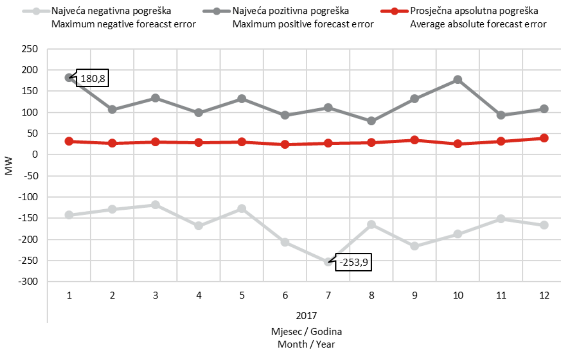
Slika 17 Maksimalna pozitivna, maksimalna negativna i prosječna apsolutna pogreška satne prognoze proizvodnje VE
