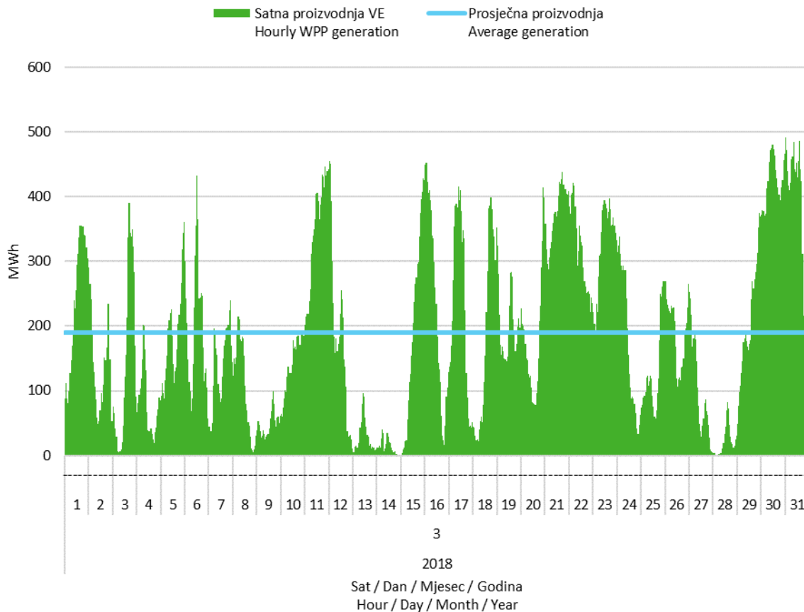
Slika 2 Satna proizvodnja svih vjetroelektrana u ožujku 2018. godine
