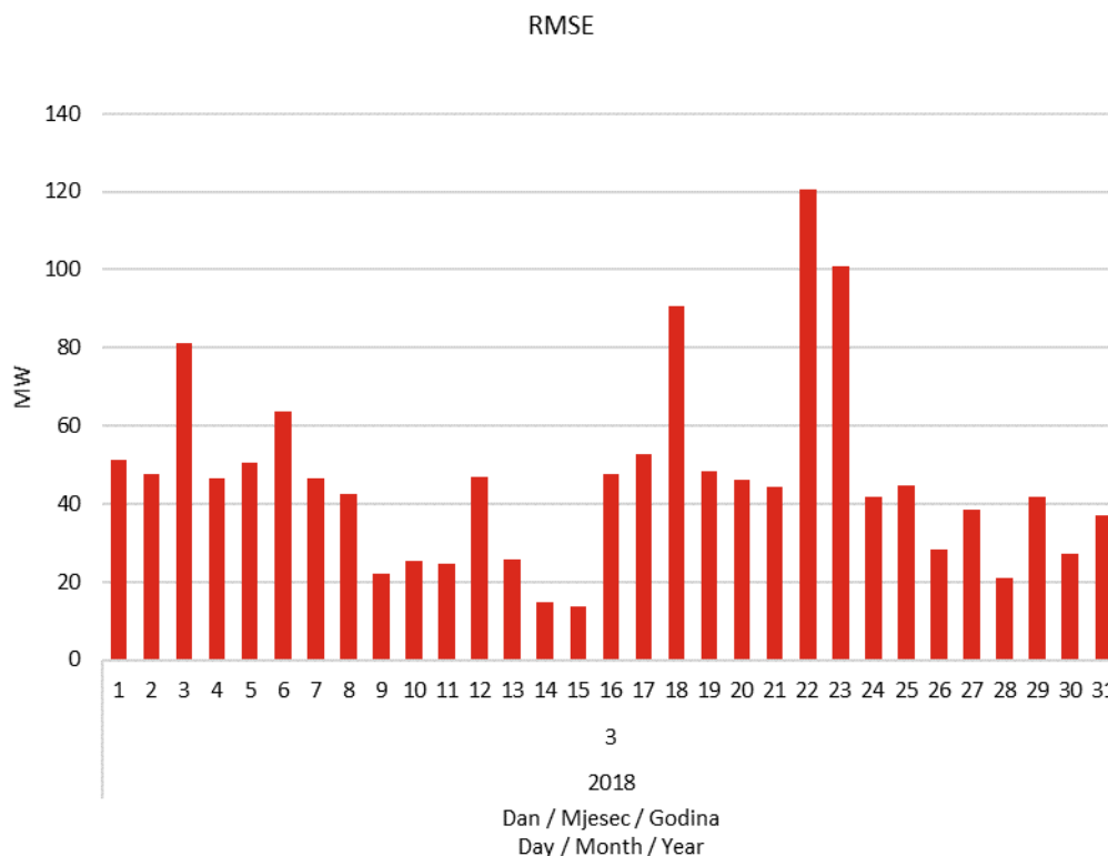
Slika 15 Korijen srednje kvadratne pogreške prognoze satne proizvodnje svih VE u ožujku 2018. godine
