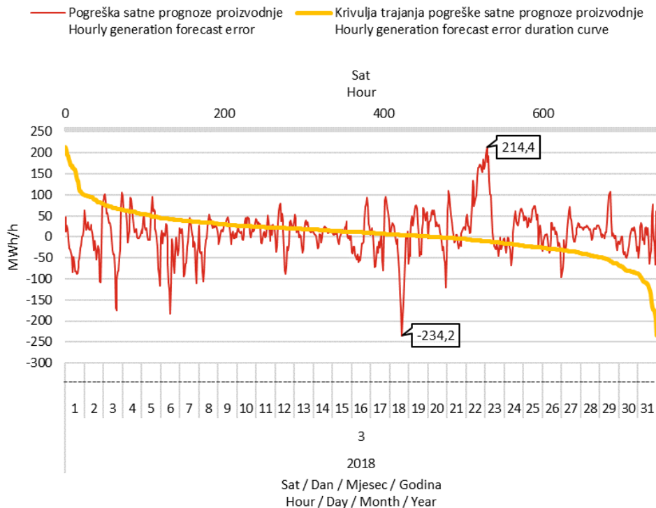
Slika 12 Razlika između prognozirane i ostvarene satne proizvodnje svih VE (pogreška prognoze) i pripadna krivulja trajanja u ožujku 2018. godine
