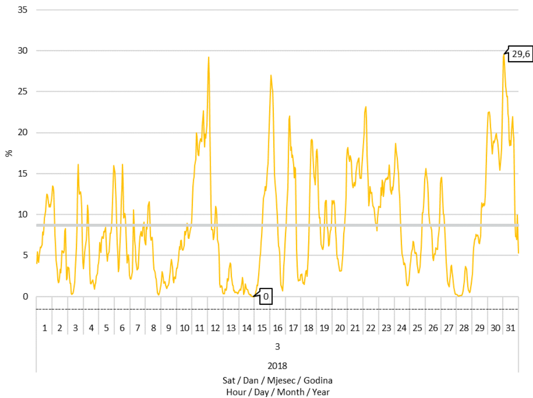
Slika 8 Udio proizvodnje vjetroelektrana u pokrivanju satnog opterećenja elektroenergetskog sustava u ožujku 2018. godine
