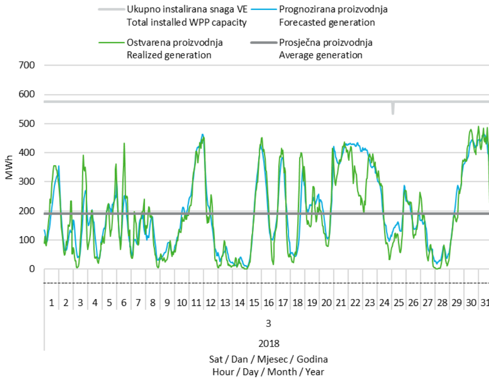
Slika 11 Prognozirana i ostvarena satna proizvodnja vjetroelektrana u ožujku 2018. godine
