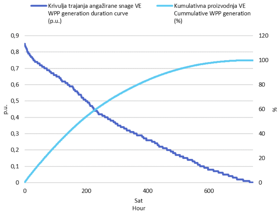
Slika 3 Krivulja trajanja angažirane snage svih VE i kumulativna proizvodnja VE u ožujku 2018. godine u jediničnim vrijednostima
