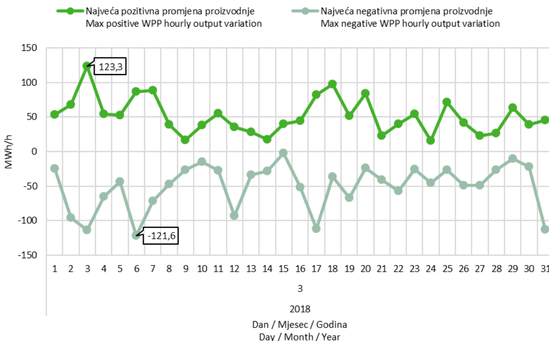
Slika 9 Maksimalna pozitivna i maksimalna negativna promjena satne proizvodnje VE u ožujku 2018. godine
