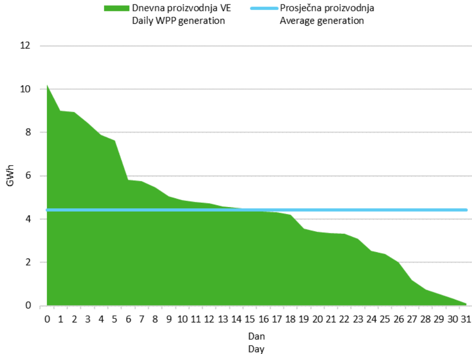
Slika 6 Krivulja trajanja dnevne proizvodnje vjetroelektrana u ožujku 2018. godine
