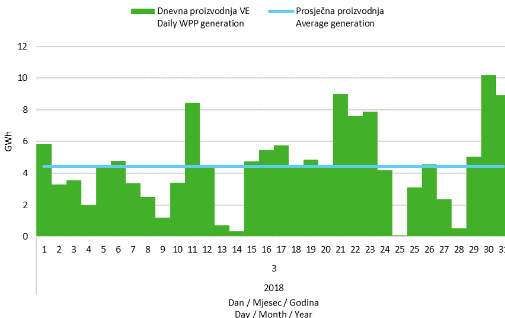
Slika 5 Dnevna proizvodnja svih vjetroelektrana u ožujku 2018. godine Figure 5 Daily generation of all wind power plants in March 2018
