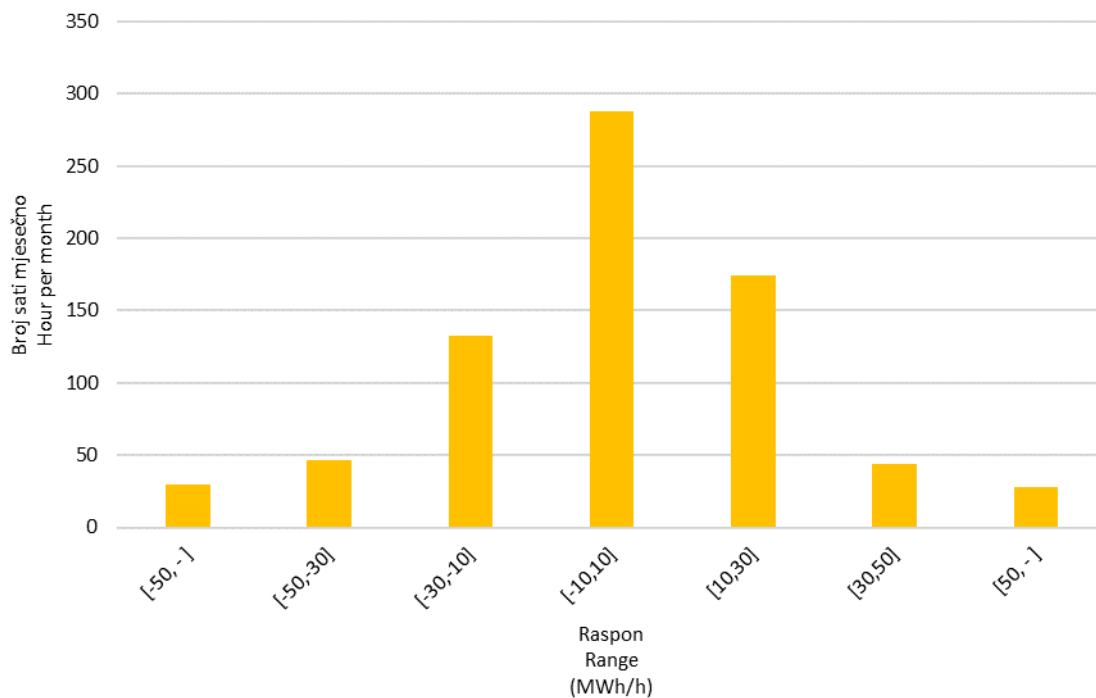
Slika 10 Statistička raspodjela satnih promjena proizvodnje VE u ožujku 2018. godine Figure 10 Statistical distribution of WPP hourly output variations in March 2018
