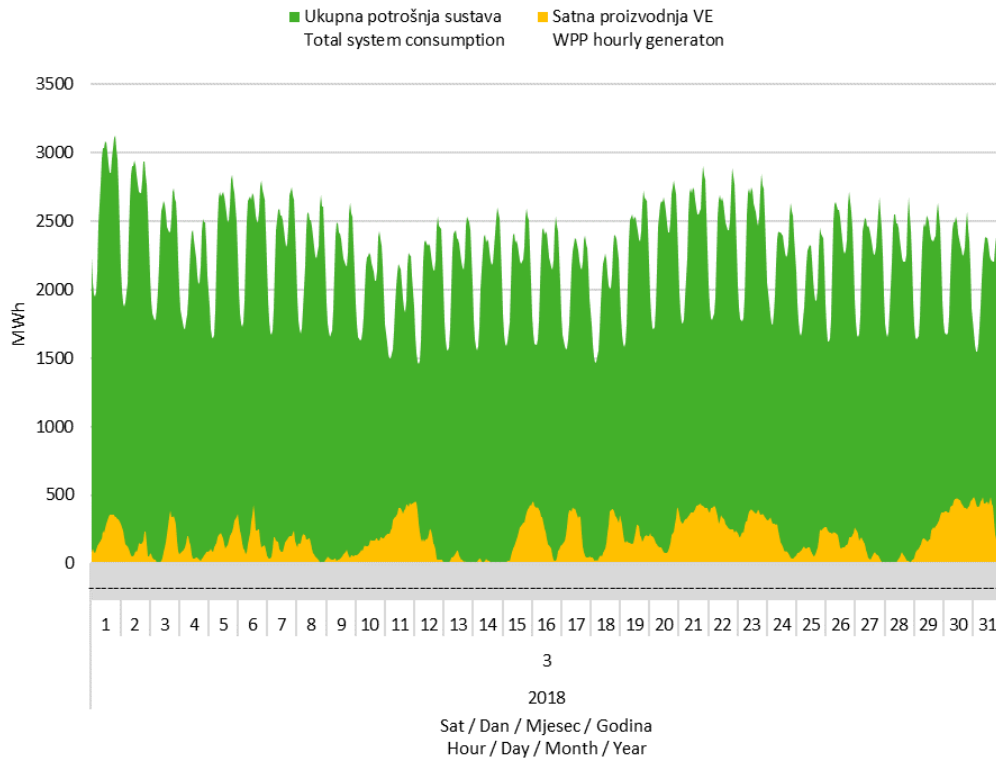
Slika 7 Usporedba satnog dijagrama opterećenja sustava i proizvodnje vjetroelektrana u ožujku 2018. godine
