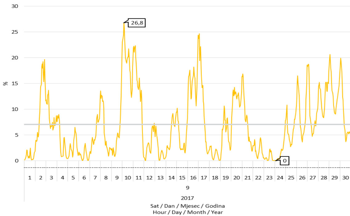
Slika 8 Udio proizvodnje vjetroelektrana u pokrivanju satnog opterećenja elektroenergetskog sustava u rujnu 2017. godine
