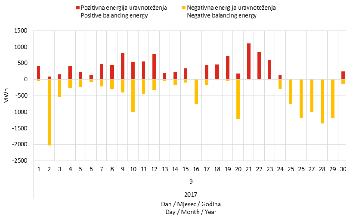
Slika 14 Suma pozitivnih pogreški prognoze satne proizvodnje VE (negativna energija uravnoteženja) i suma negativnih pogreški prognoze satne proizvodnje VE (pozitivna energija uravnoteženja) u rujnu 2017. godine
