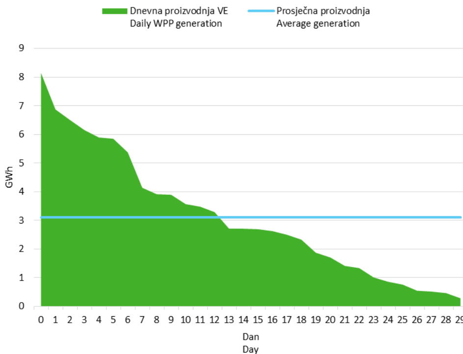
Slika 6 Krivulja trajanja dnevne proizvodnje vjetroelektrana u rujnu 2017. godine
