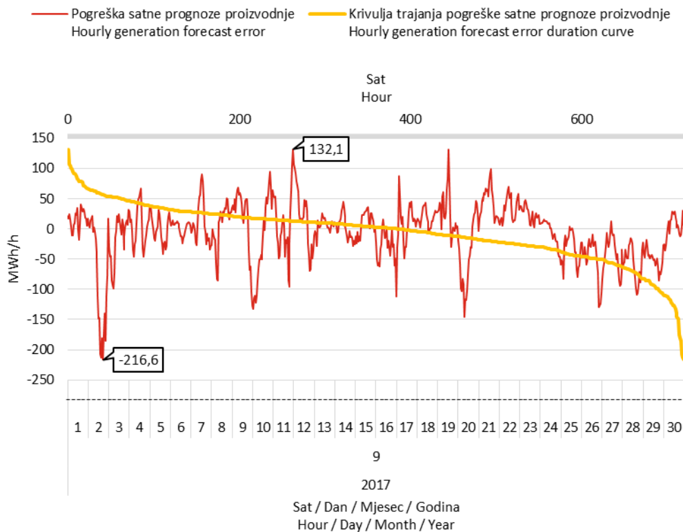
Slika 12 Razlika između prognozirane i ostvarene satne proizvodnje svih VE (pogreška prognoze) i pripadna krivulja trajanja u rujnu 2017. godine
