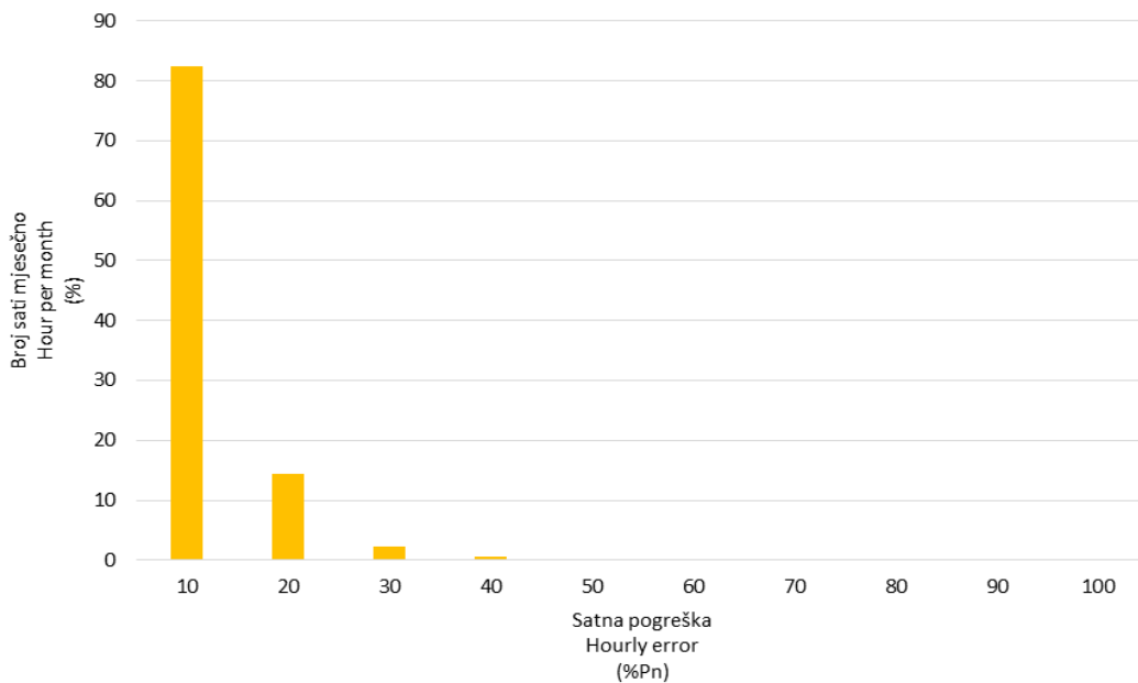
Slika 17 Frekvencija pojavljivanja pogreške prognoze satne proizvodnje svih VE u rujnu 2017. godine
