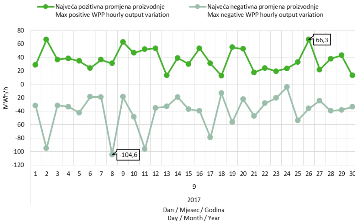
Slika 9 Maksimalna pozitivna i maksimalna negativna promjena satne proizvodnje VE u rujnu 2017. godine
