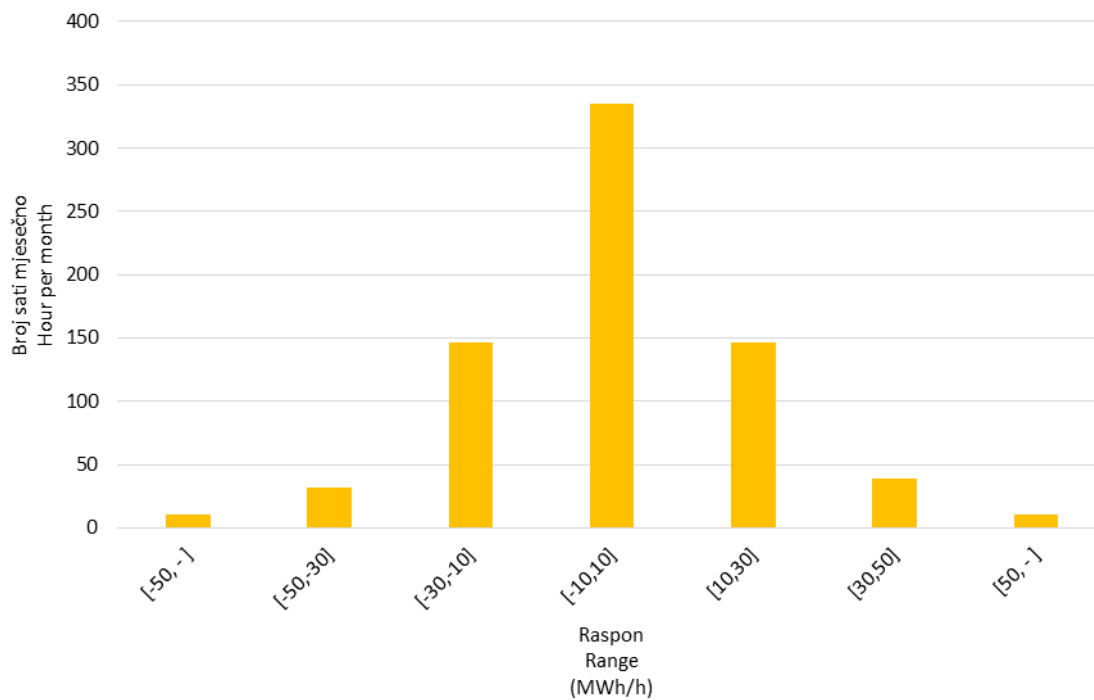
Slika 10 Statistička raspodjela satnih promjena proizvodnje VE u rujnu 2017. godine Figure 10 Statistical distribution of WPP hourly output variations in September 2017
