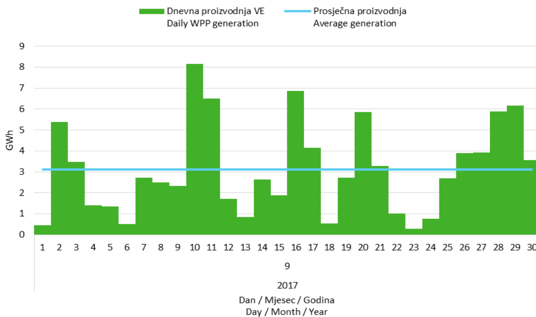
Slika 5 Dnevna proizvodnja svih vjetroelektrana u rujnu 2017. godine
