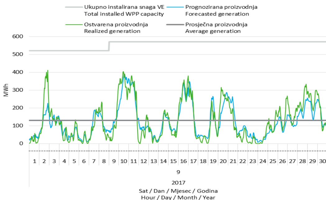
Slika 11 Prognozirana i ostvarena satna proizvodnja vjetroelektrana u rujnu 2017. godine
