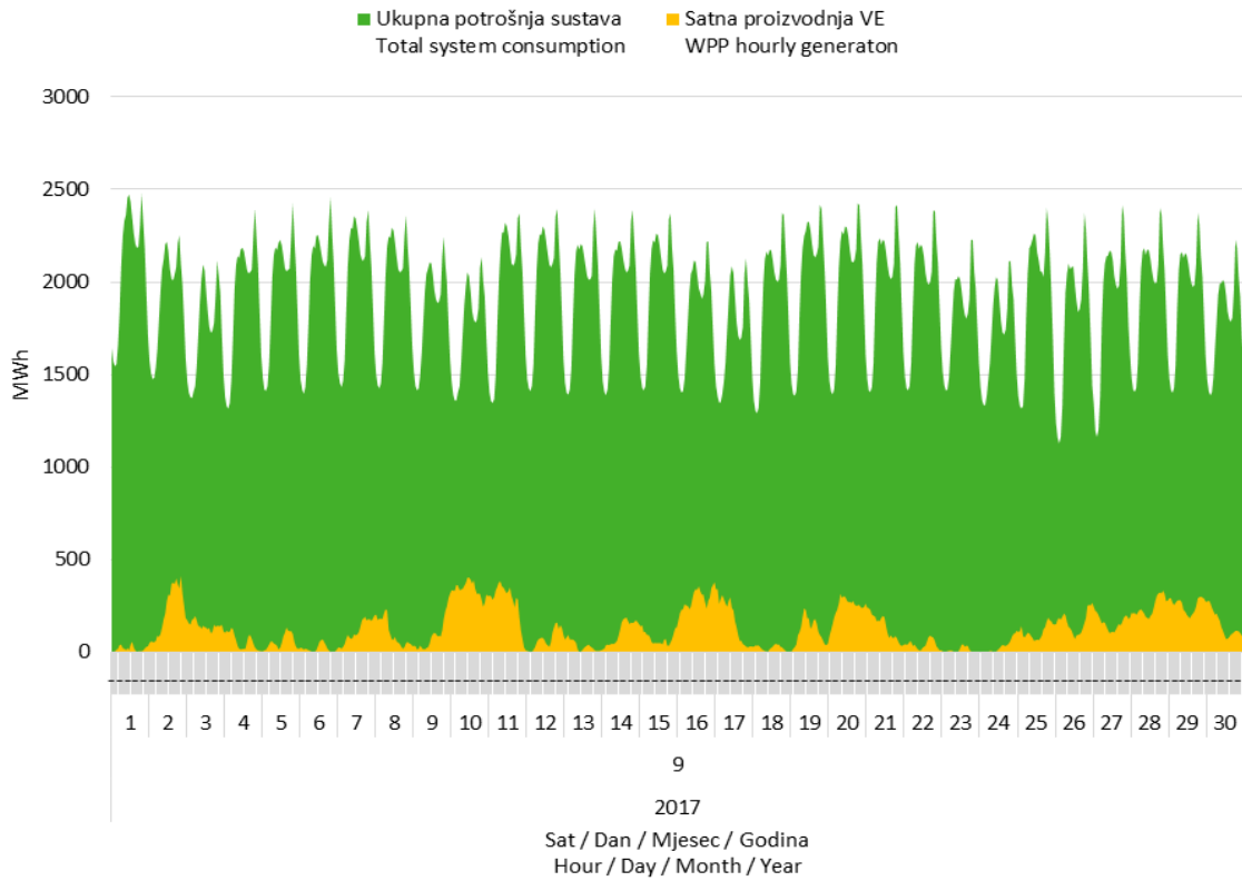
Slika 7 Usporedba satnog dijagrama opterećenja sustava i proizvodnje vjetroelektrana u rujnu 2017. godine
