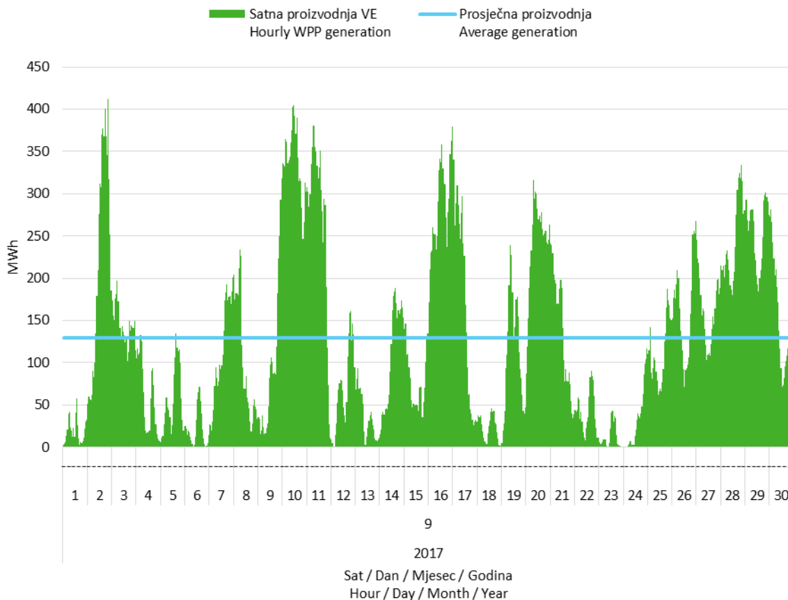
Slika 2 Satna proizvodnja svih vjetroelektrana u rujnu 2017. godine Figure 2 Hourly generation of all wind power plants in September 2017
