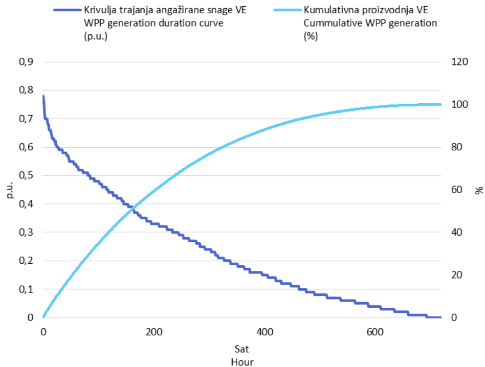
Slika 3 Krivulja trajanja angažirane snage svih VE i kumulativna proizvodnja VE u rujnu 2017. godine u jediničnim vrijednostima
