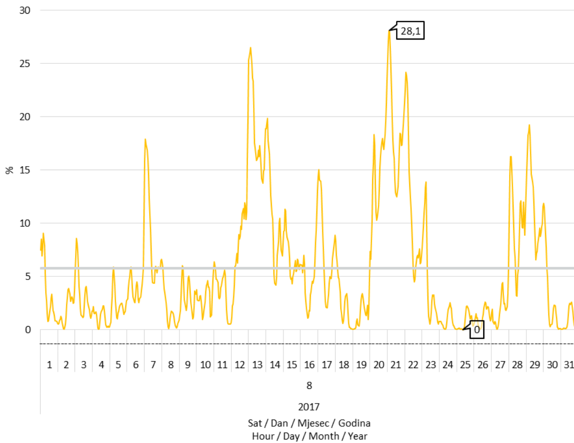
Slika 8 Udio proizvodnje vjetroelektrana u pokrivanju satnog opterećenja elektroenergetskog sustava u kolovozu 2017. godine
