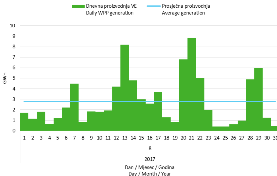
Slika 5 Dnevna proizvodnja svih vjetroelektrana u kolovozu 2017. godine
