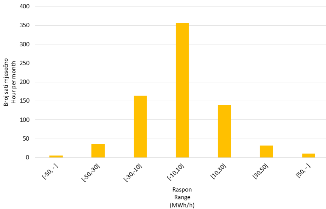
Slika 10 Statistička raspodjela satnih promjena proizvodnje VE u kolovozu 2017. godine
