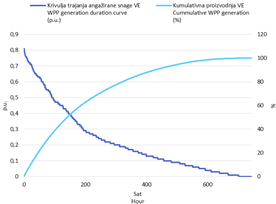
Slika 3 Krivulja trajanja angažirane snage svih VE i kumulativna proizvodnja VE u kolovozu 2017. godine u jediničnim vrijednostima
