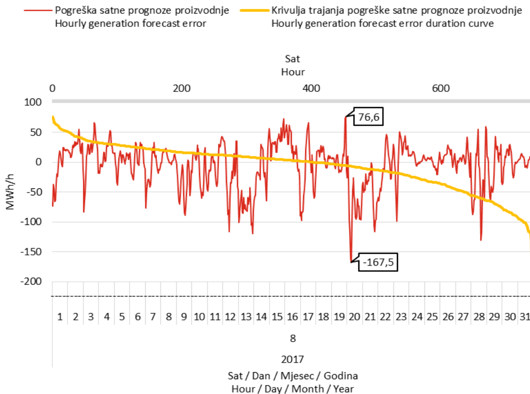
Slika 12 Razlika između prognozirane i ostvarene satne proizvodnje svih VE (pogreška prognoze) i pripadna krivulja trajanja u kolovozu 2017. godine
