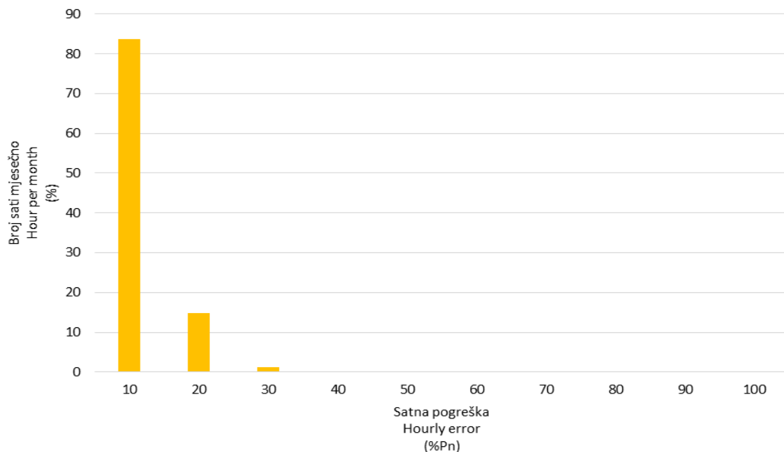
Slika 17 Frekvencija pojavljivanja pogreške prognoze satne proizvodnje svih VE u kolovozu 2017. godine
