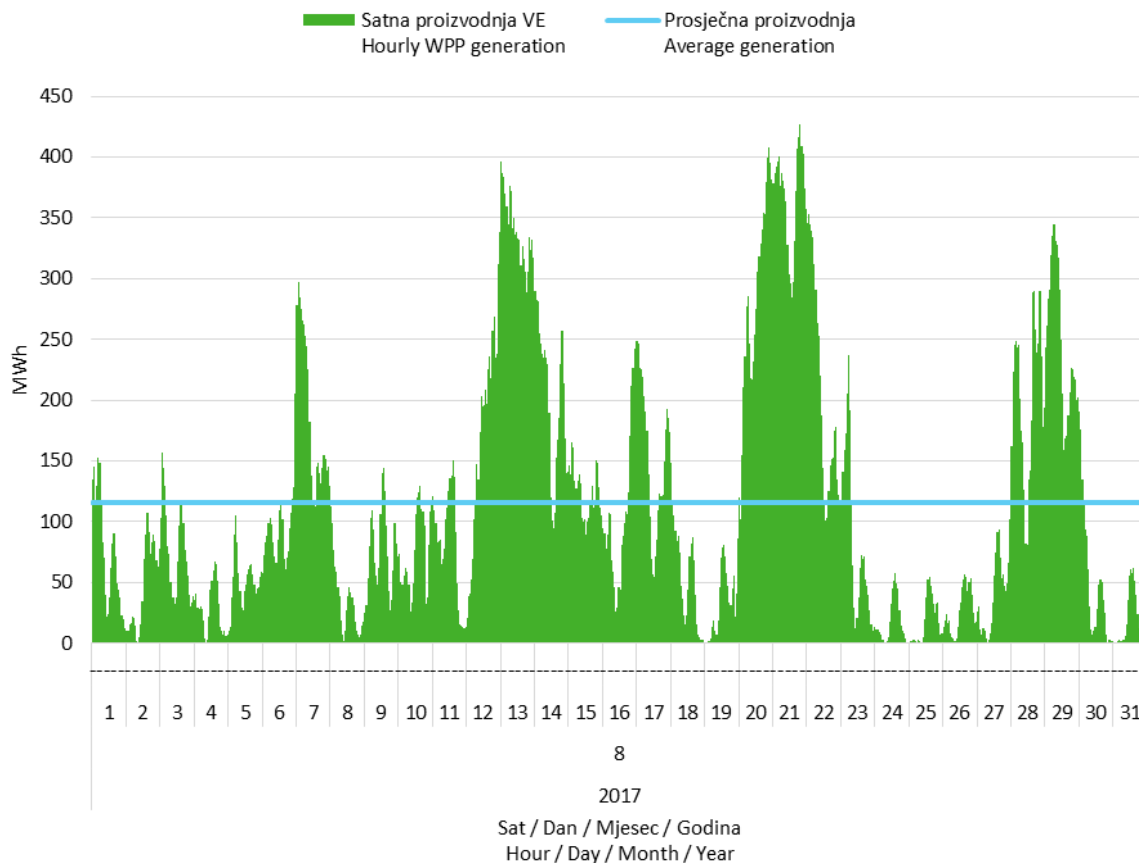
Slika 2 Satna proizvodnja svih vjetroelektrana u kolovozu 2017. godine
