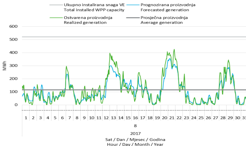
Slika 11 Prognozirana i ostvarena satna proizvodnja vjetroelektrana u kolovozu 2017. godine
