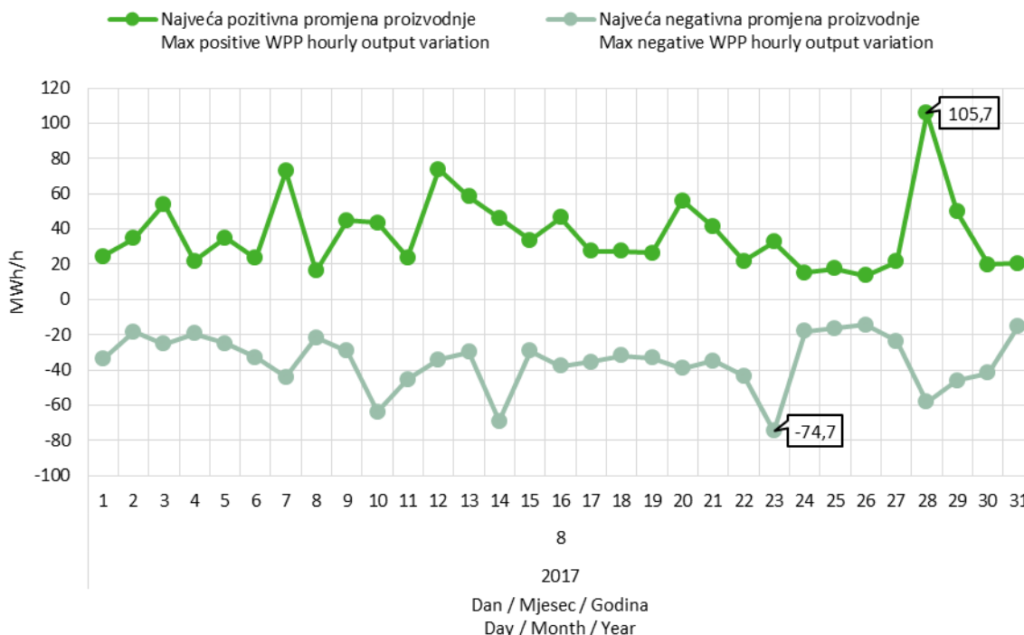
Slika 9 Maksimalna pozitivna i maksimalna negativna promjena satne proizvodnje VE u kolovozu 2017. godine
