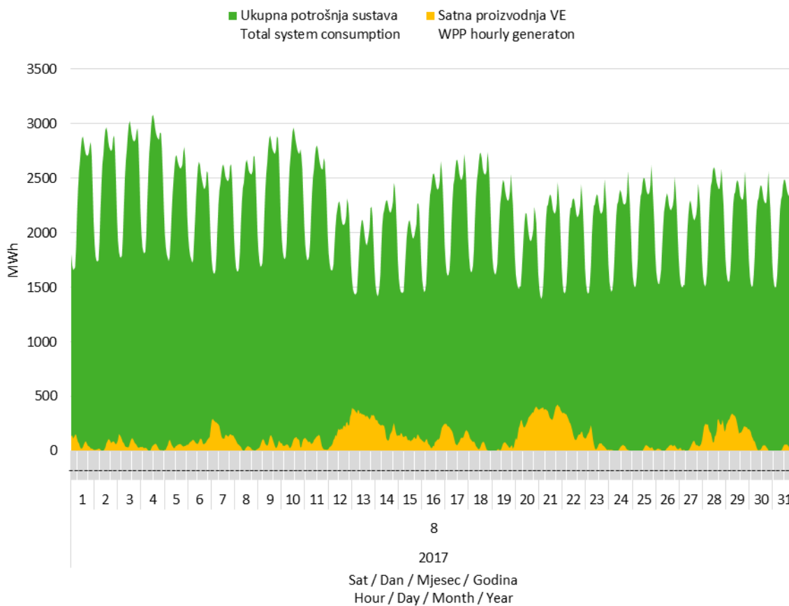
Slika 7 Usporedba satnog dijagrama opterećenja sustava i proizvodnje vjetroelektrana u kolovozu 2017. godine
