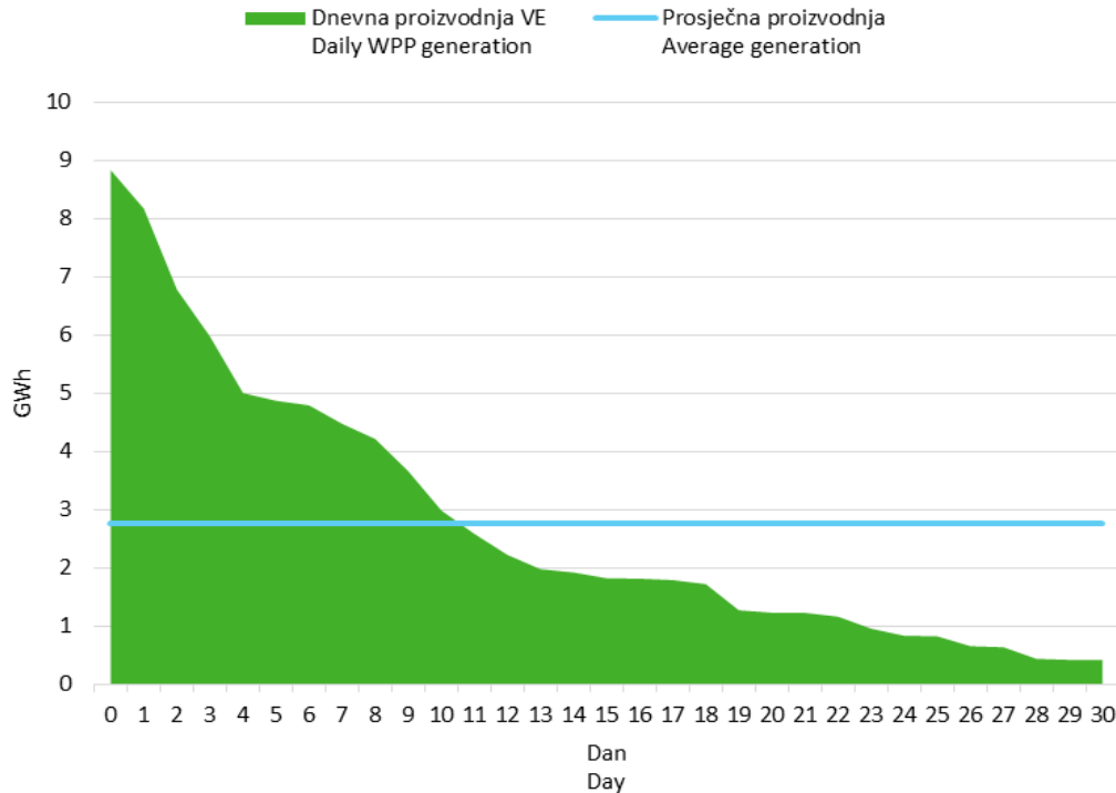
Slika 6 Krivulja trajanja dnevne proizvodnje vjetroelektrana u kolovozu 2017. godine
