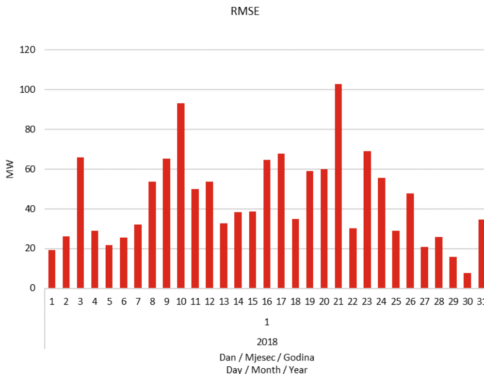
Slika 15 Korijen srednje kvadratne pogreške prognoze satne proizvodnje svih VE u siječnju 2018. godine
