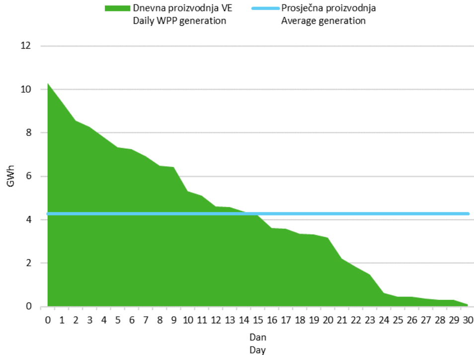
Slika 6 Krivulja trajanja dnevne proizvodnje vjetroelektrana u siječnju 2018. godine
