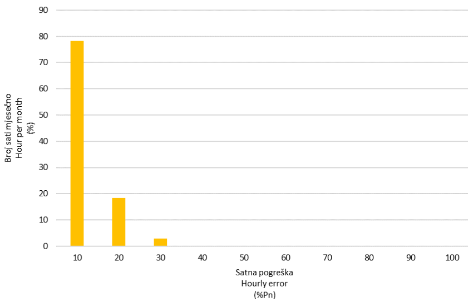
Slika 17 Frekvencija pojavljivanja pogreške prognoze satne proizvodnje svih VE u siječnju 2018. godine
