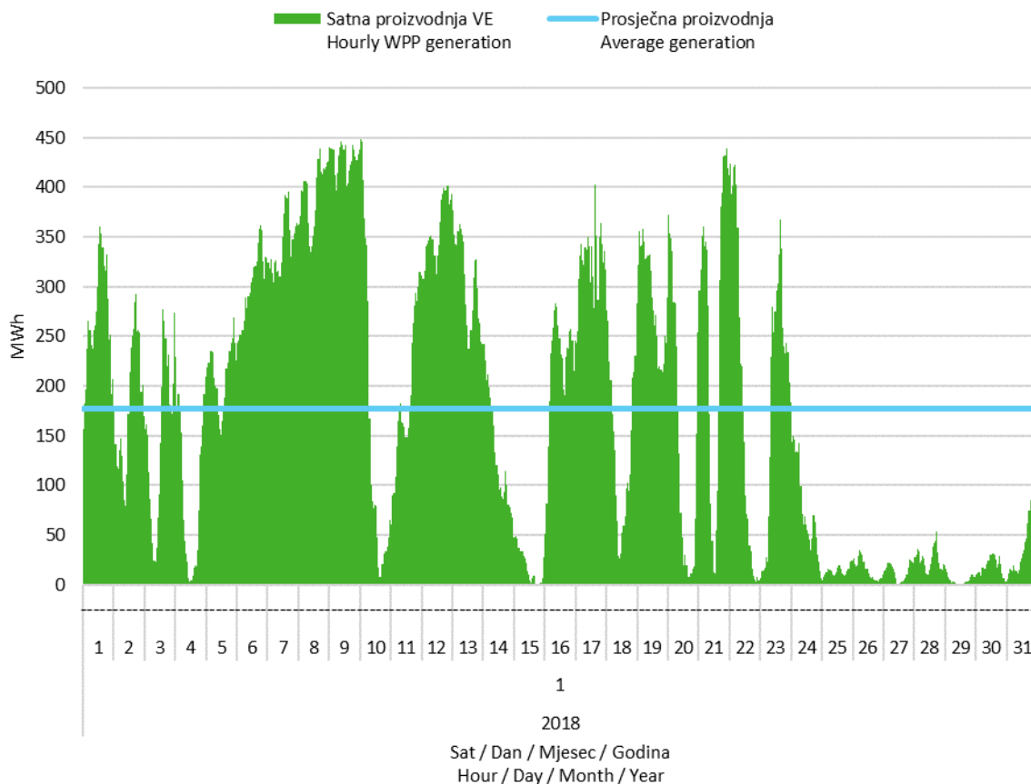
Slika 2 Satna proizvodnja svih vjetroelektrana u siječnju 2018. godine
