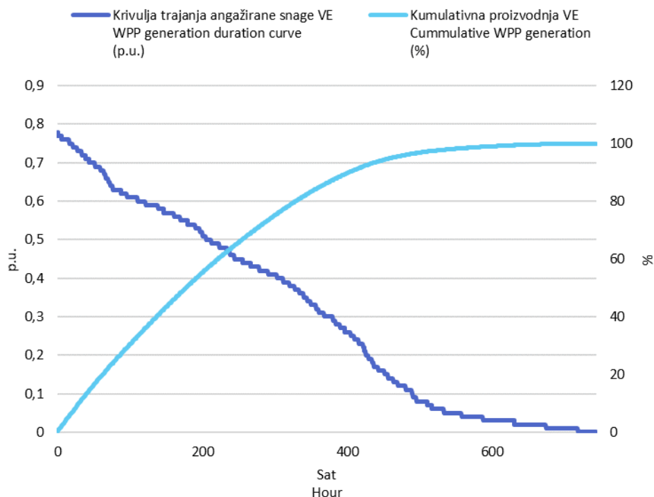
Slika 3 Krivulja trajanja angažirane snage svih VE i kumulativna proizvodnja VE u siječnju 2018. godine u jediničnim vrijednostima
