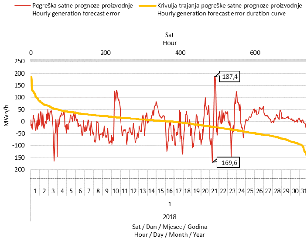
Slika 12 Razlika između prognozirane i ostvarene satne proizvodnje svih VE (pogreška prognoze) i pripadna krivulja trajanja u siječnju 2018. godine
