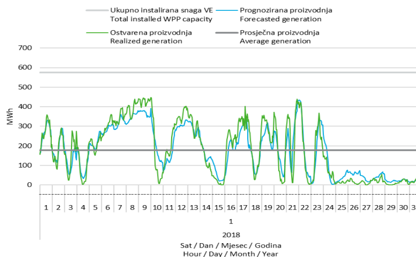
Slika 11 Prognozirana i ostvarena satna proizvodnja vjetroelektrana u siječnju 2018. godine
