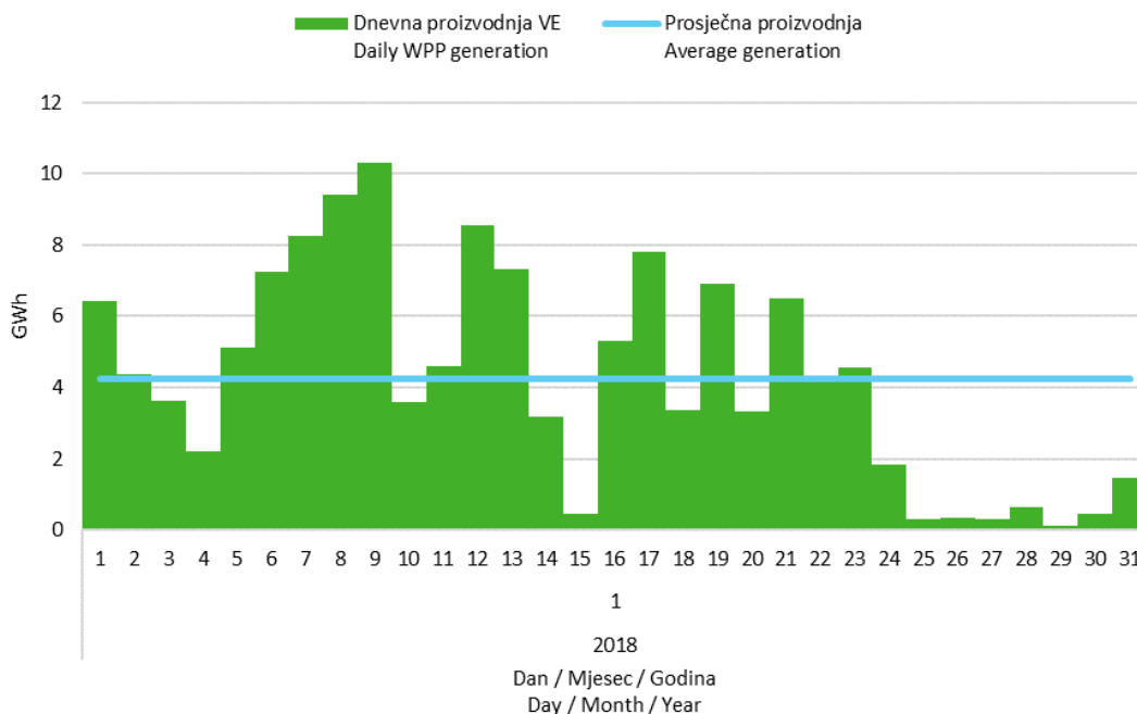
Slika 5 Dnevna proizvodnja svih vjetroelektrana u siječnju 2018. godine
