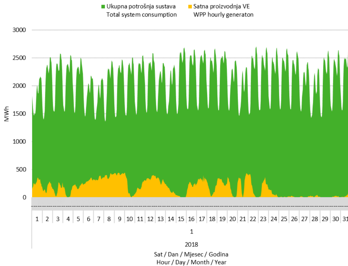
Slika 7 Usporedba satnog dijagrama opterećenja sustava i proizvodnje vjetroelektrana u siječnju 2018. godine
