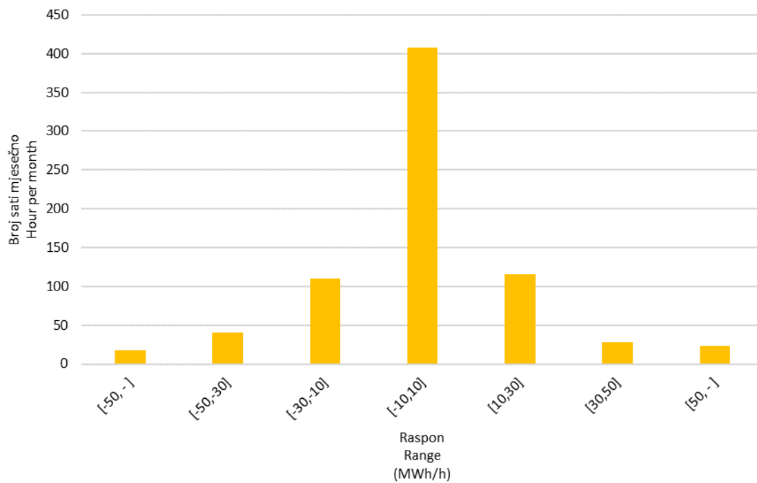
Slika 10 Statistička raspodjela satnih promjena proizvodnje VE u siječnju 2018. godine
