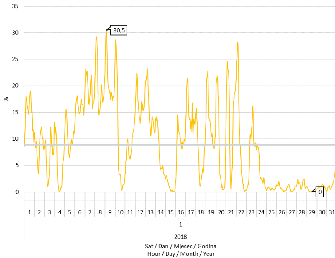
Slika 8 Udio proizvodnje vjetroelektrana u pokrivanju satnog opterećenja elektroenergetskog sustava u siječnju 2018. godine
