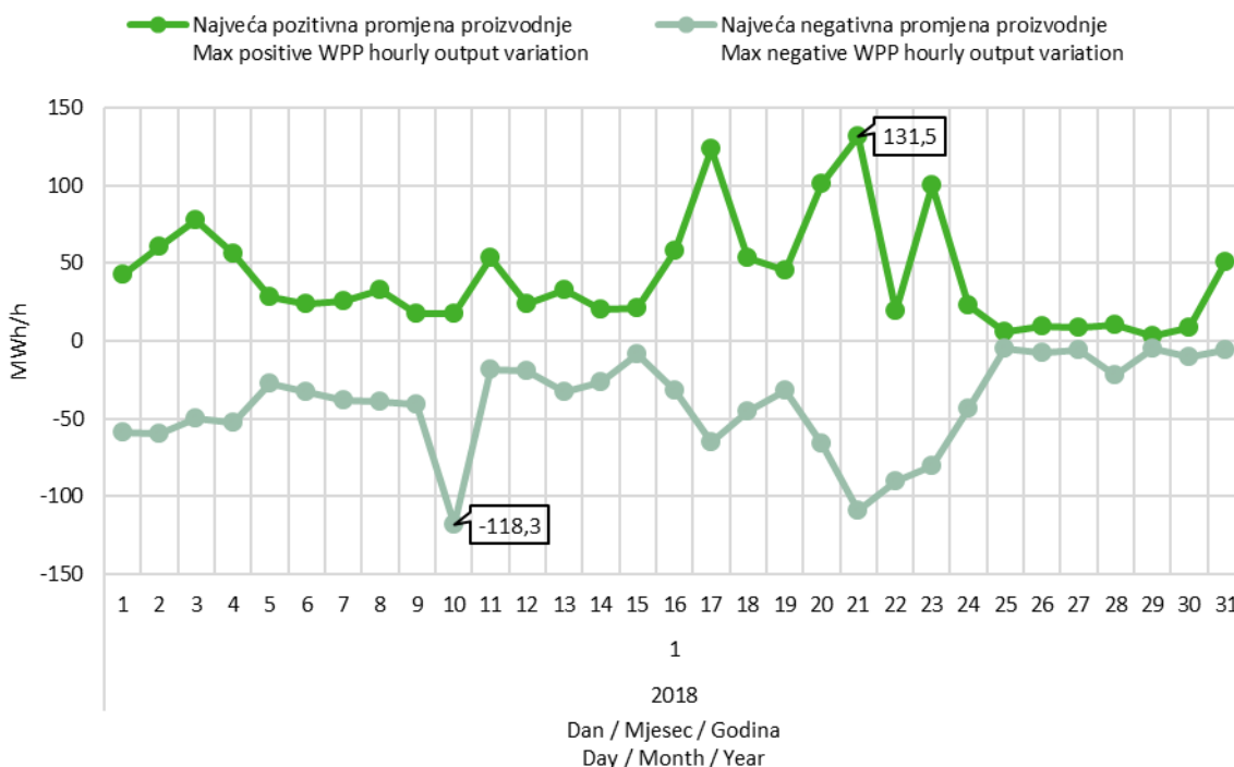
Slika 9 Maksimalna pozitivna i maksimalna negativna promjena satne proizvodnje VE u siječnju 2018. godine
