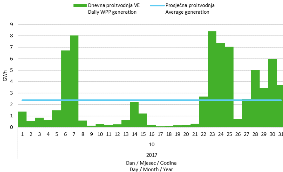
Slika 5 Dnevna proizvodnja svih vjetroelektrana u listopadu 2017. godine
