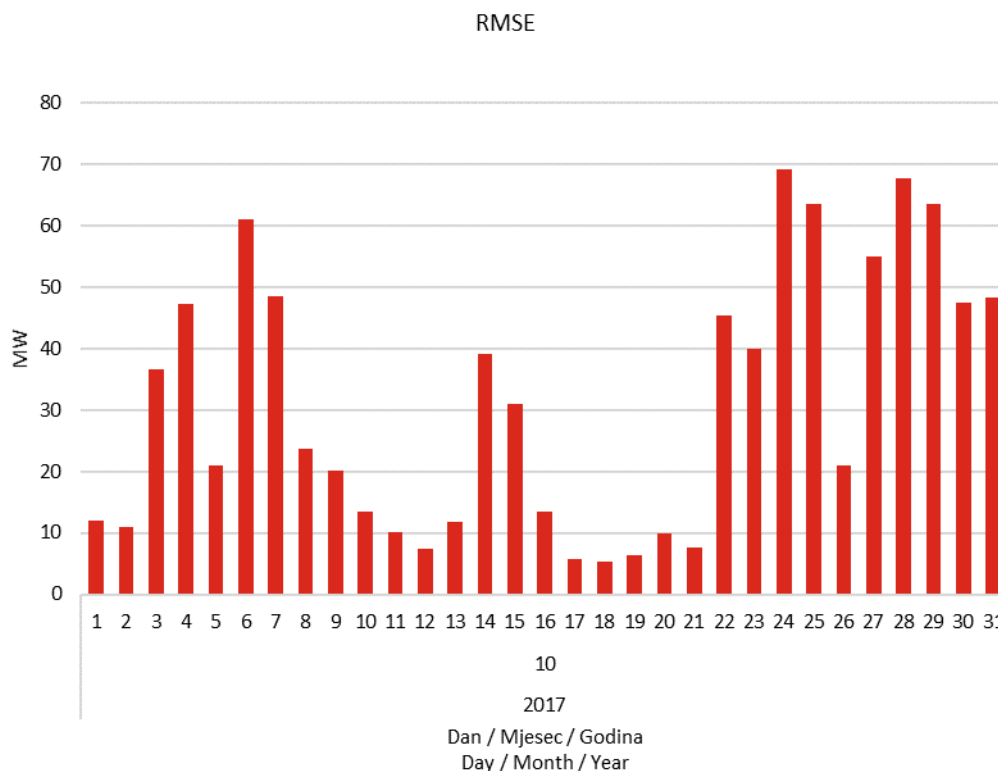
Slika 15 Korijen srednje kvadratne pogreške prognoze satne proizvodnje svih VE u listopadu 2017. godine
