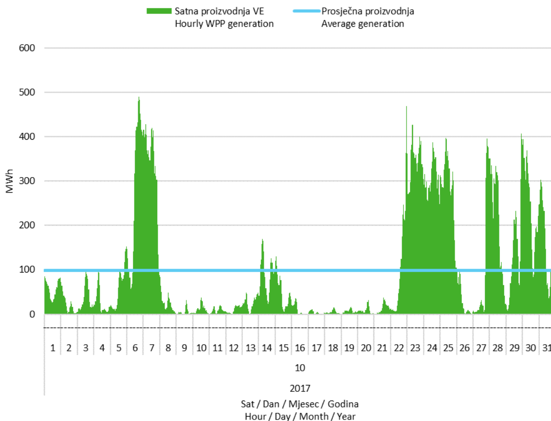
Slika 2 Satna proizvodnja svih vjetroelektrana u listopadu 2017. godine
