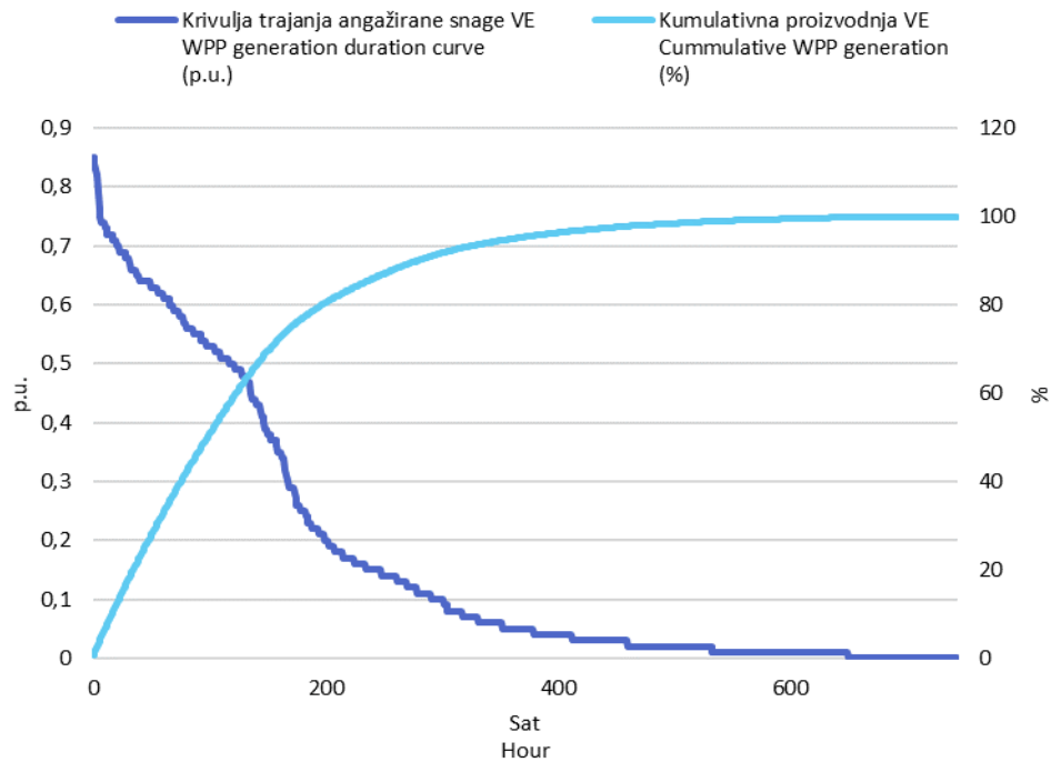
Slika 3 Krivulja trajanja angažirane snage svih VE i kumulativna proizvodnja VE u listopadu 2017. godine u jediničnim vrijednostima
