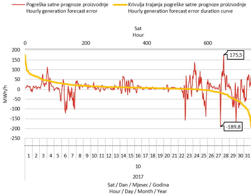
Slika 12 Razlika između prognozirane i ostvarene satne proizvodnje svih VE (pogreška prognoze) i pripadna krivulja trajanja u listopadu 2017. godine
