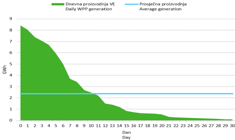
Slika 6 Krivulja trajanja dnevne proizvodnje vjetroelektrana u listopadu 2017. godine
