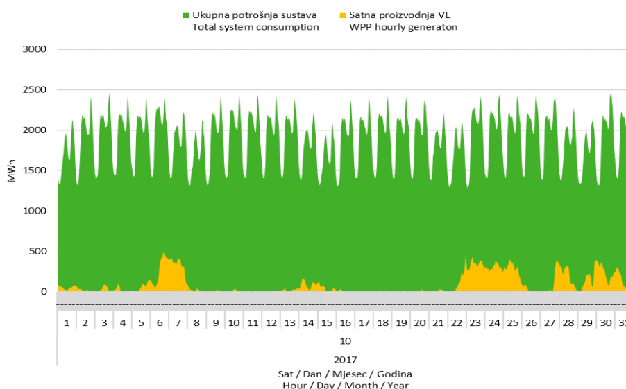
Slika 7 Usporedba satnog dijagrama opterećenja sustava i proizvodnje vjetroelektrana u listopadu 2017. godine
