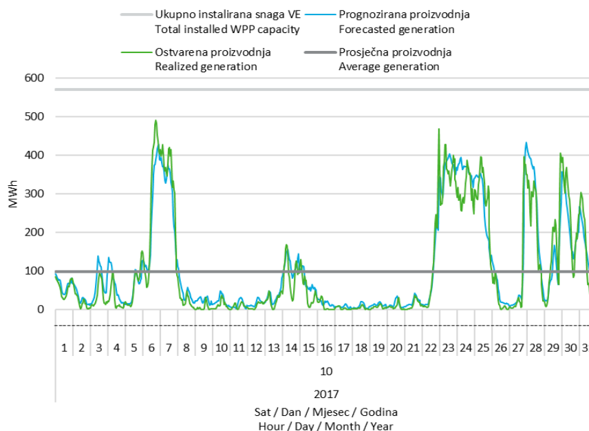
Slika 11 Prognozirana i ostvarena satna proizvodnja vjetroelektrana u listopadu 2017. godine
