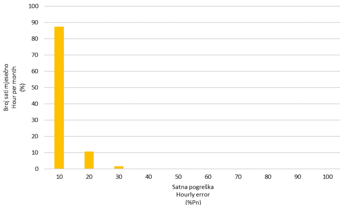
Slika 17 Frekvencija pojavljivanja pogreške prognoze satne proizvodnje svih VE u listopadu 2017. godine
