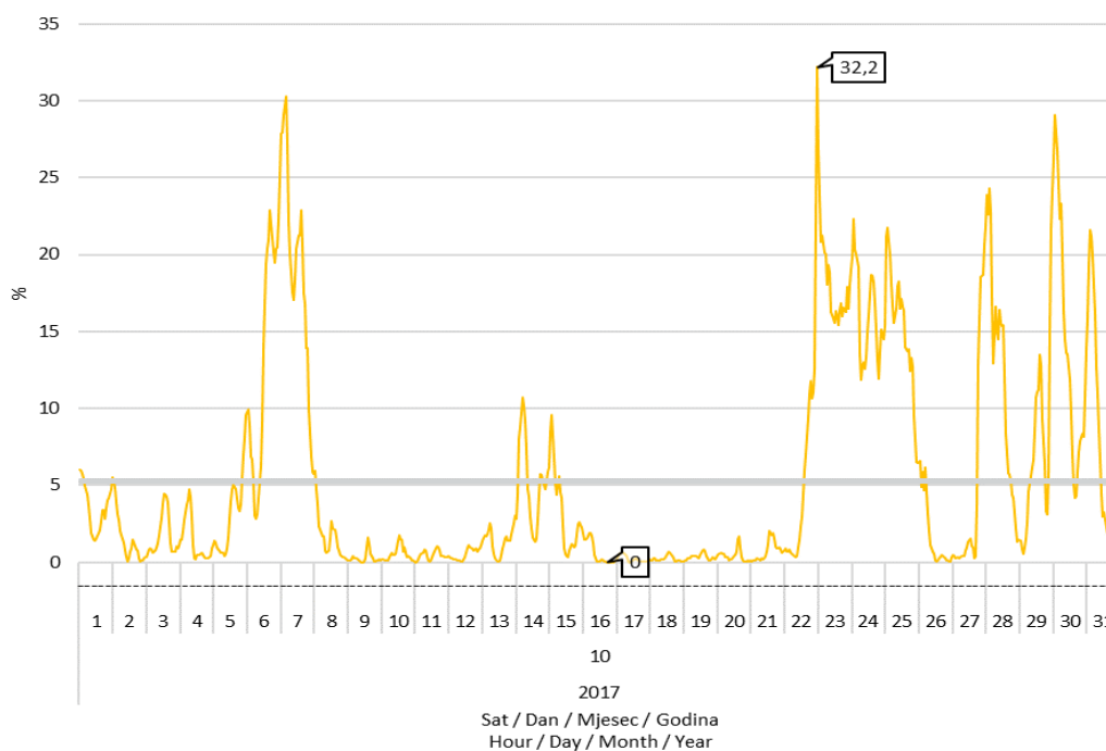
Slika 8 Udio proizvodnje vjetroelektrana u pokrivanju satnog opterećenja elektroenergetskog sustava u listopadu 2017. godine
