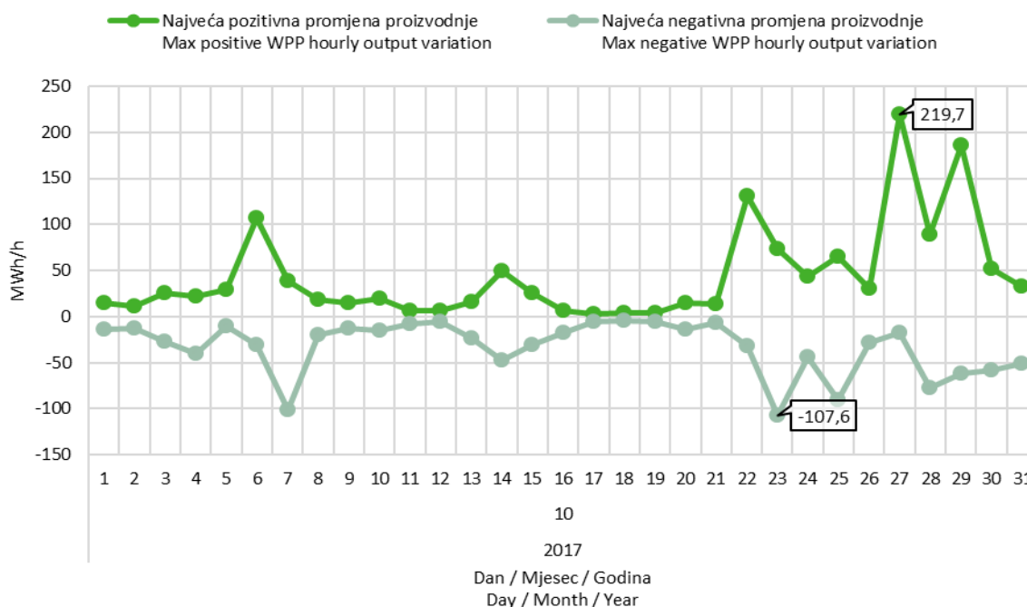
Slika 9 Maksimalna pozitivna i maksimalna negativna promjena satne proizvodnje VE u listopadu 2017. godine
