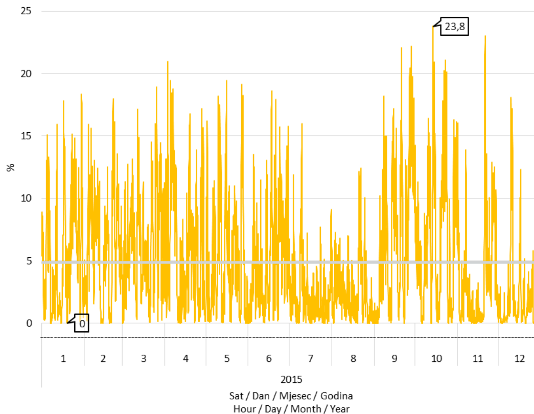
Slika 12 Udio proizvodnje vjetroelektrana u pokrivanju satnog opterećenja elektroenergetskog sustava Figure 12 WPP generation share in covering power system demand
