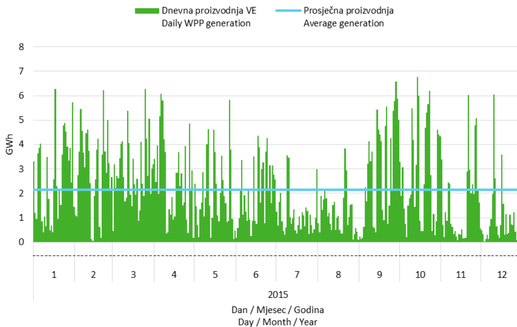
Slika 6 Dnevna proizvodnja svih vjetroelektrana
