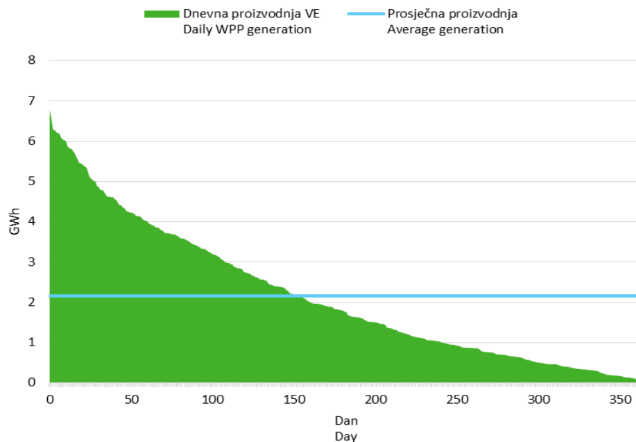
Slika 7 Krivulja trajanja dnevne proizvodnje vjetroelektrana
