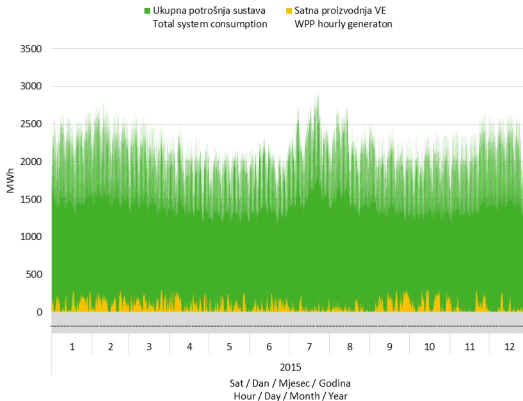
Slika 11 Usporedba satnog dijagrama opterećenja sustava i proizvodnje vjetroelektrana Figure 11 Comparison between hourly system demand and WPP generation
