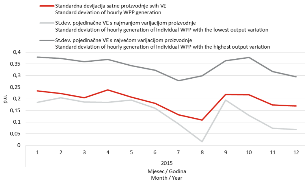
Slika 5 Standardna devijacija satne proizvodnje vjetroelektrana u jediničnim vrijednostima
