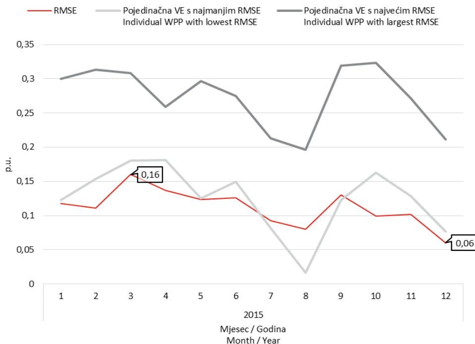
Slika 21 Korijen srednje kvadratne pogreške prognoze satne proizvodnje svih VE u jediničnim vrijednostima
