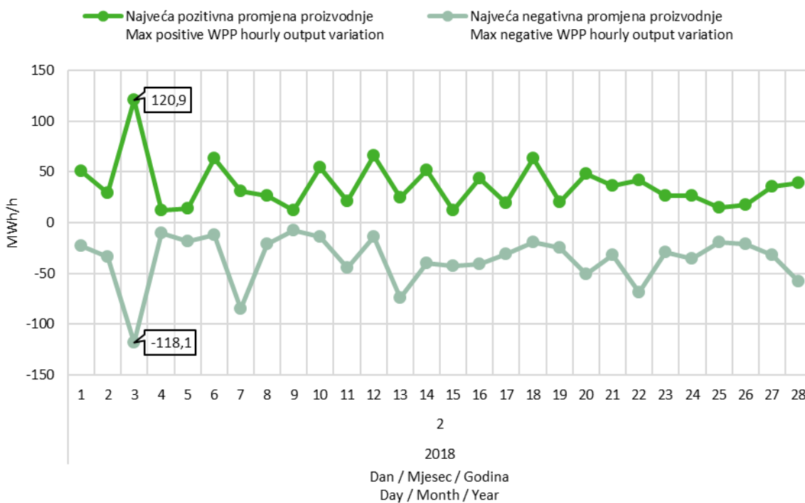
Slika 9 Maksimalna pozitivna i maksimalna negativna promjena satne proizvodnje VE u veljači 2018. godine
