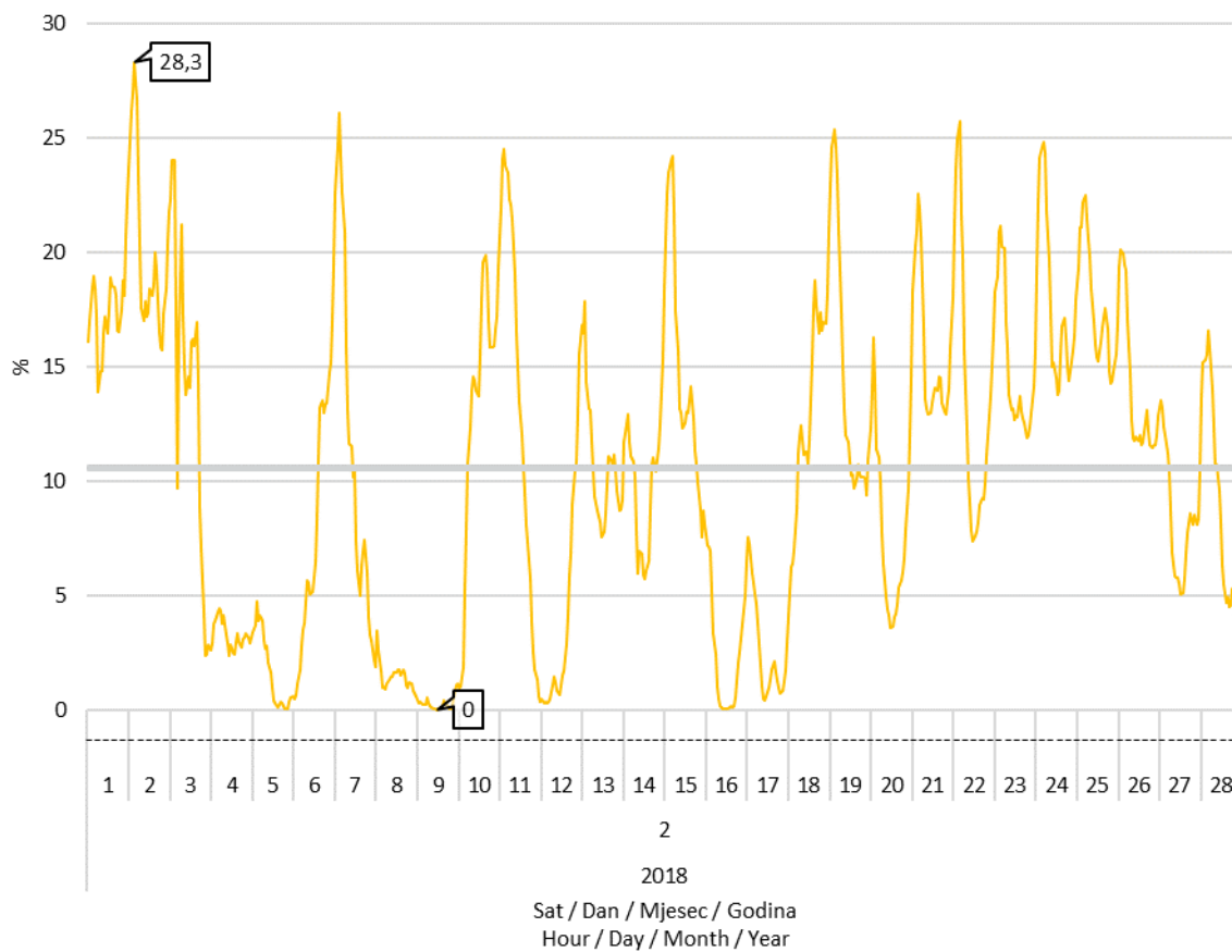
Slika 8 Udio proizvodnje vjetroelektrana u pokrivanju satnog opterećenja elektroenergetskog sustava u veljači 2018. godine
