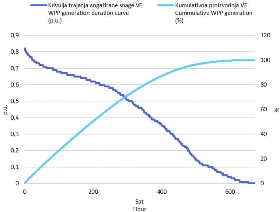
Slika 3 Krivulja trajanja angažirane snage svih VE i kumulativna proizvodnja VE u veljači 2018. godine u jediničnim vrijednostima
