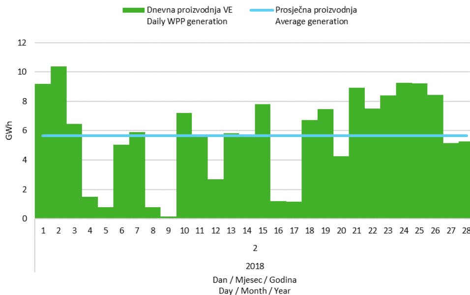
Slika 5 Dnevna proizvodnja svih vjetroelektrana u veljači 2018. godine
