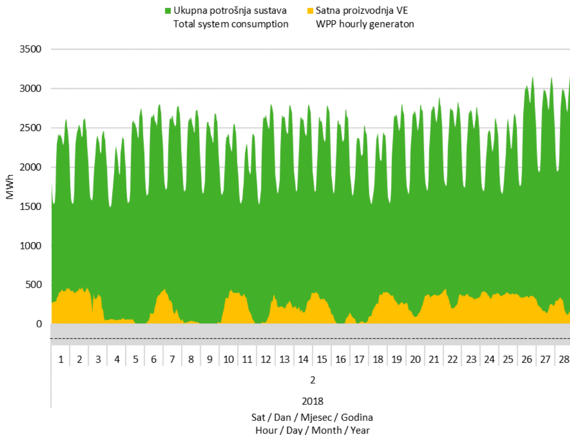
Slika 7 Usporedba satnog dijagrama opterećenja sustava i proizvodnje vjetroelektrana u veljači 2018. godine
