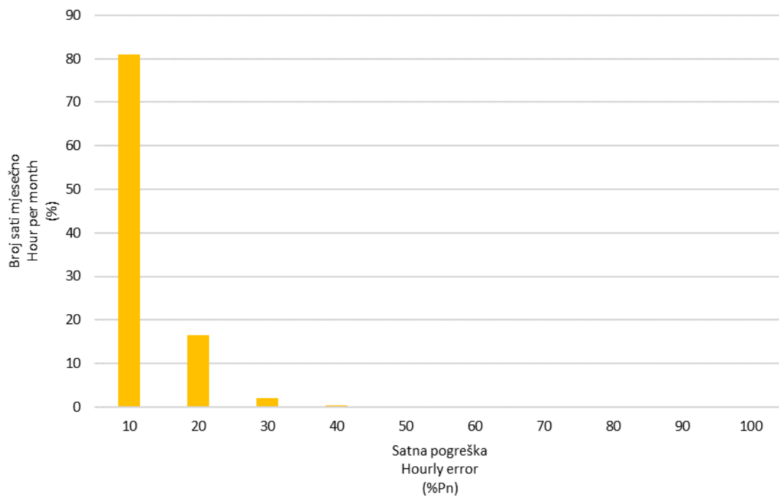
Slika 17 Frekvencija pojavljivanja pogreške prognoze satne proizvodnje svih VE u veljači 2018. godine
