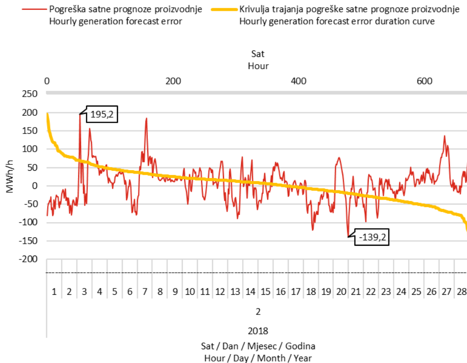
Slika 12 Razlika između prognozirane i ostvarene satne proizvodnje svih VE (pogreška prognoze) i pripadna krivulja trajanja u veljači 2018. godine
