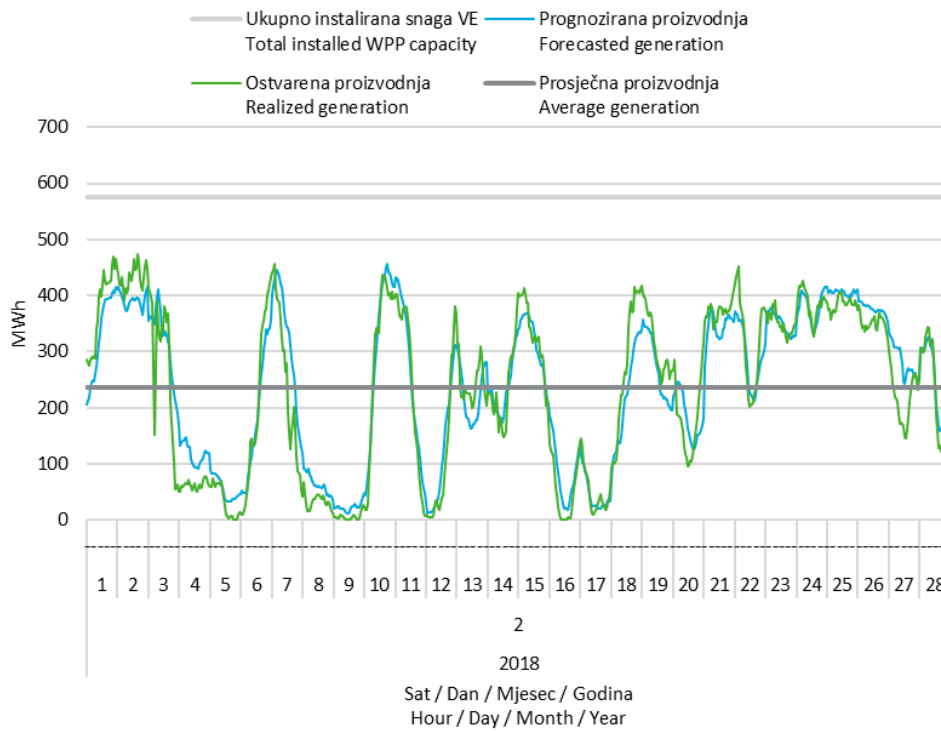
Slika 11 Prognozirana i ostvarena satna proizvodnja vjetroelektrana u veljači 2018. godine
