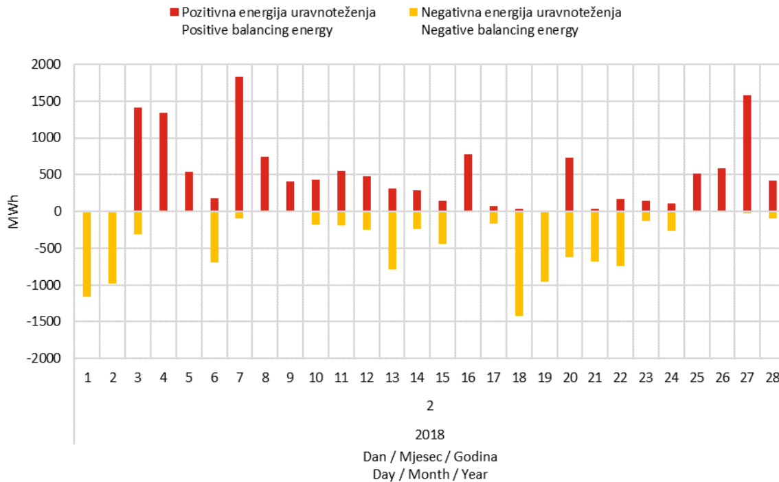
Slika 14 Suma pozitivnih pogreški prognoze satne proizvodnje VE (negativna energija uravnoteženja) i suma negativnih pogreški prognoze satne proizvodnje VE (pozitivna energija uravnoteženja) u veljači 2018. godine
