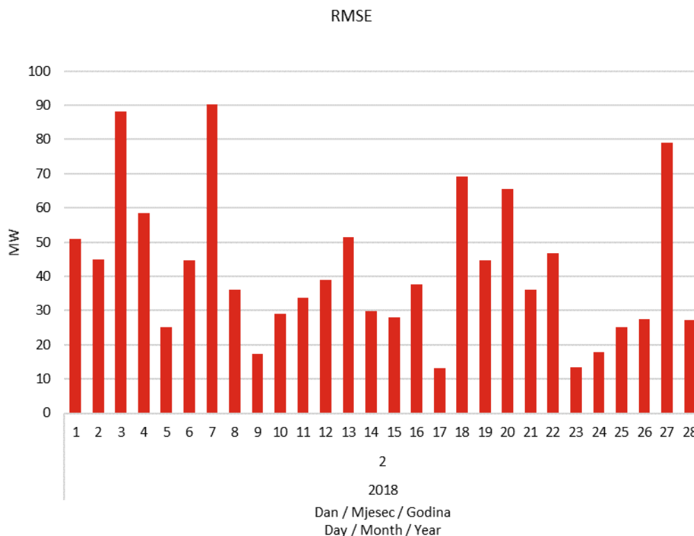
Slika 15 Korijen srednje kvadratne pogreške prognoze satne proizvodnje svih VE u veljači 2018. godine
