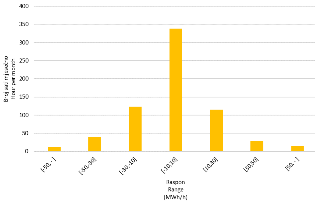
Slika 10 Statistička raspodjela satnih promjena proizvodnje VE u veljači 2018. godine
