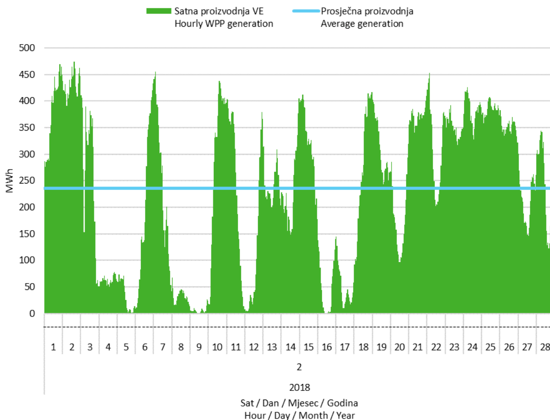
Slika 2 Satna proizvodnja svih vjetroelektrana u veljači 2018. godine Figure 2 Hourly generation of all wind power plants in February 2018
