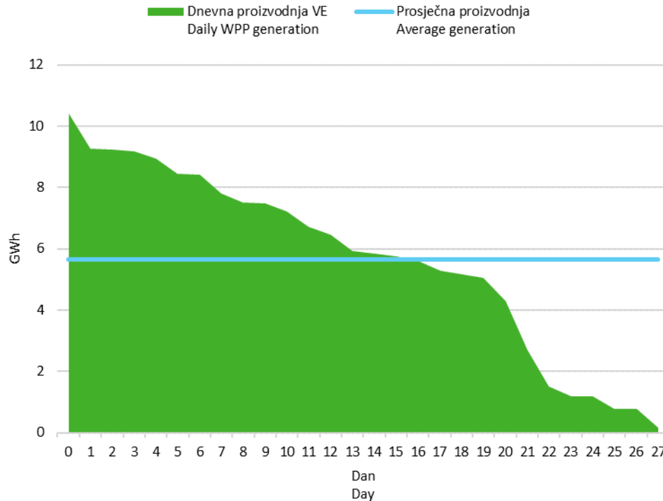
Slika 6 Krivulja trajanja dnevne proizvodnje vjetroelektrana u veljači 2018. godine
