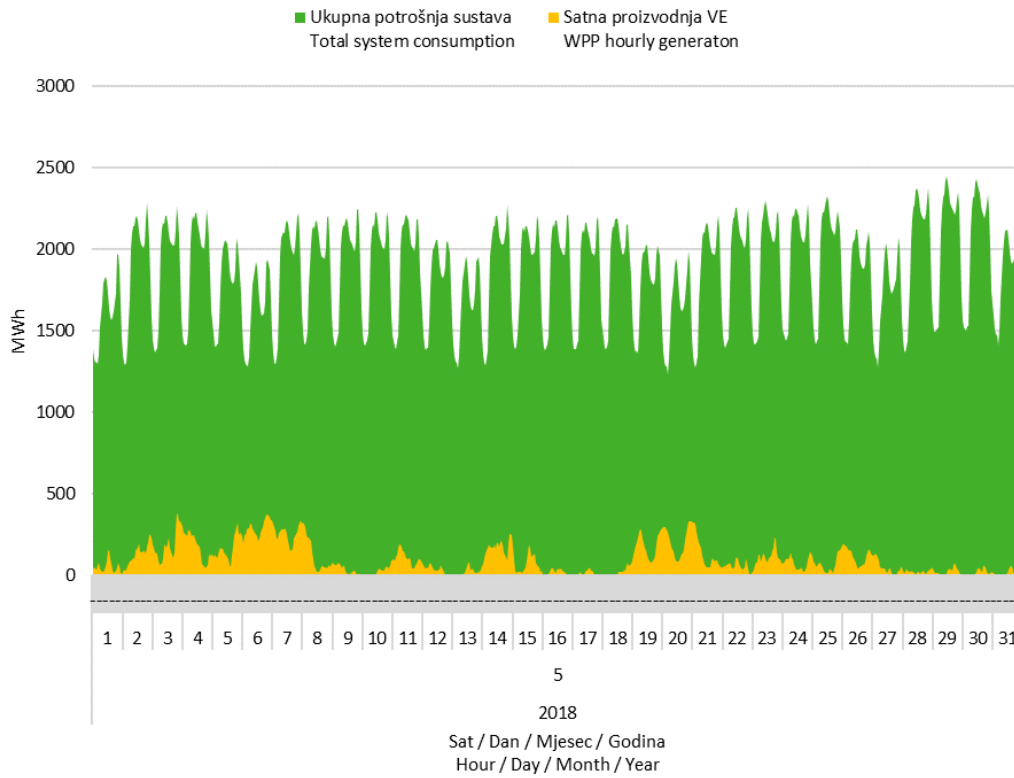
Slika 7 Usporedba satnog dijagrama opterećenja sustava i proizvodnje vjetroelektrana u svibnju 2018. godine
