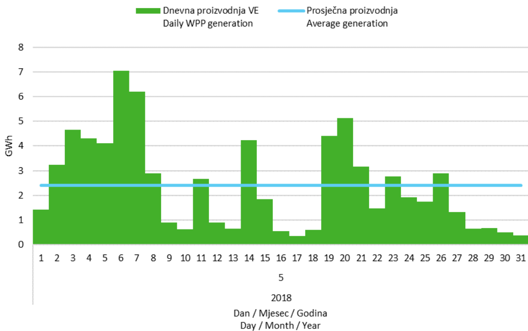
Slika 5 Dnevna proizvodnja svih vjetroelektrana u svibnju 2018. godine
