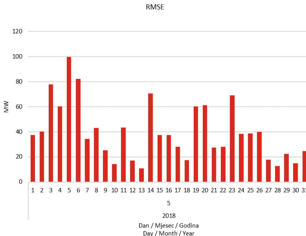
Slika 15 Korijen srednje kvadratne pogreške prognoze satne proizvodnje svih VE u svibnju 2018. godine
