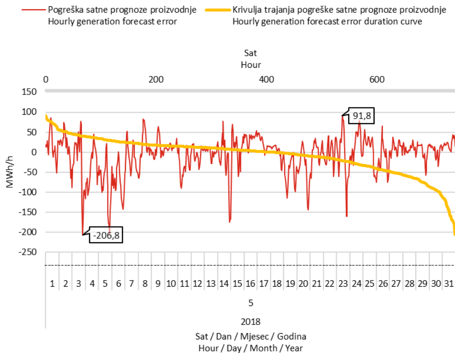
Slika 12 Razlika između prognozirane i ostvarene satne proizvodnje svih VE (pogreška prognoze) i pripadna krivulja trajanja u svibnju 2018. godine
