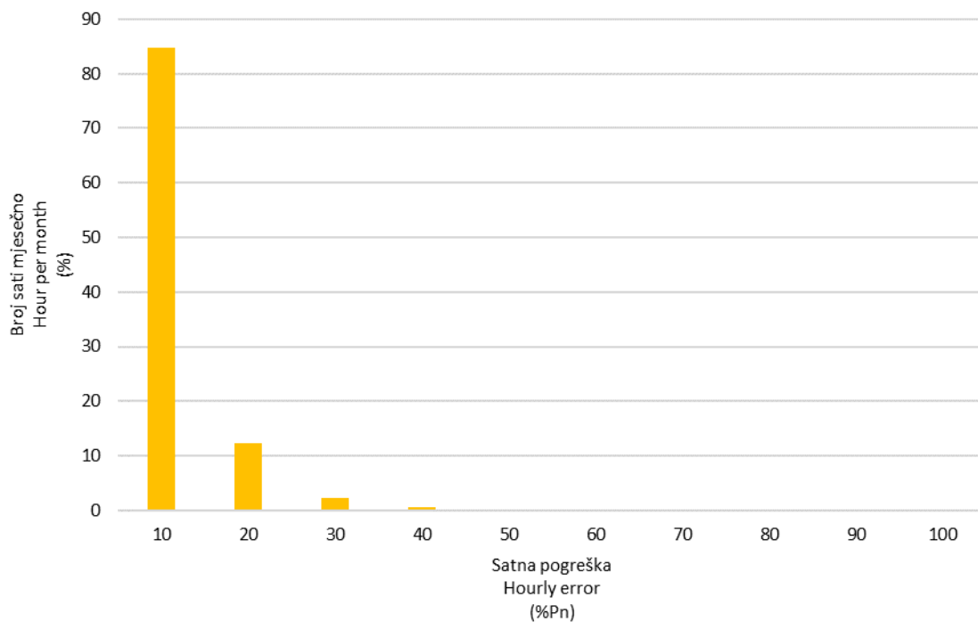
Slika 17 Frekvencija pojavljivanja pogreške prognoze satne proizvodnje svih VE u svibnju 2018. godine
