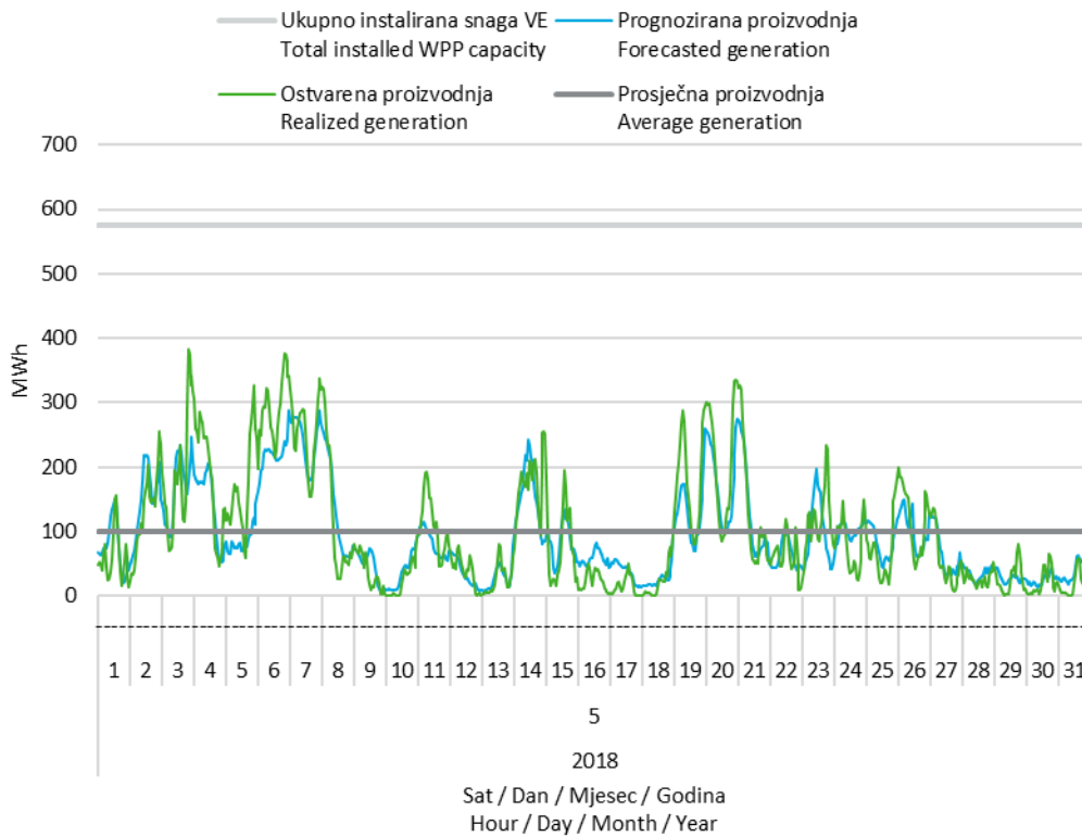
Slika 11 Prognozirana i ostvarena satna proizvodnja vjetroelektrana u svibnju 2018. godine
