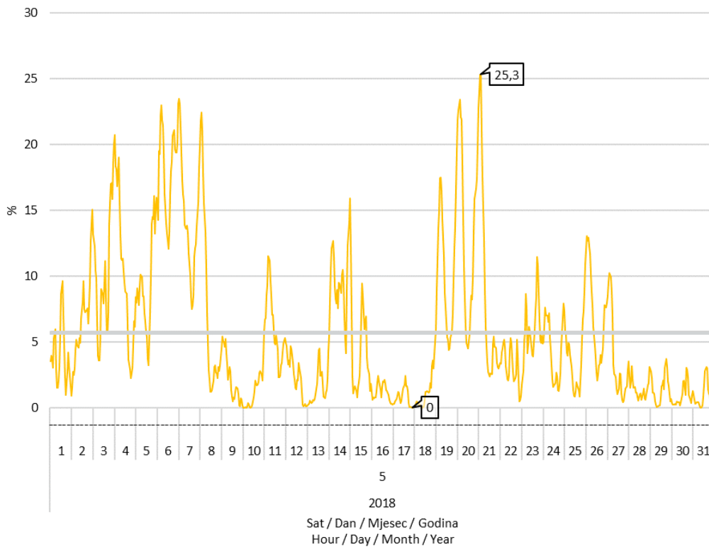
Slika 8 Udio proizvodnje vjetroelektrana u pokrivanju satnog opterećenja elektroenergetskog sustava u svibnju 2018. godine
