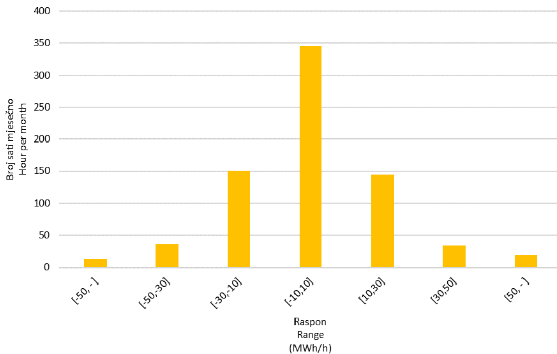
Slika 10 Statistička raspodjela satnih promjena proizvodnje VE u svibnju 2018. godine
