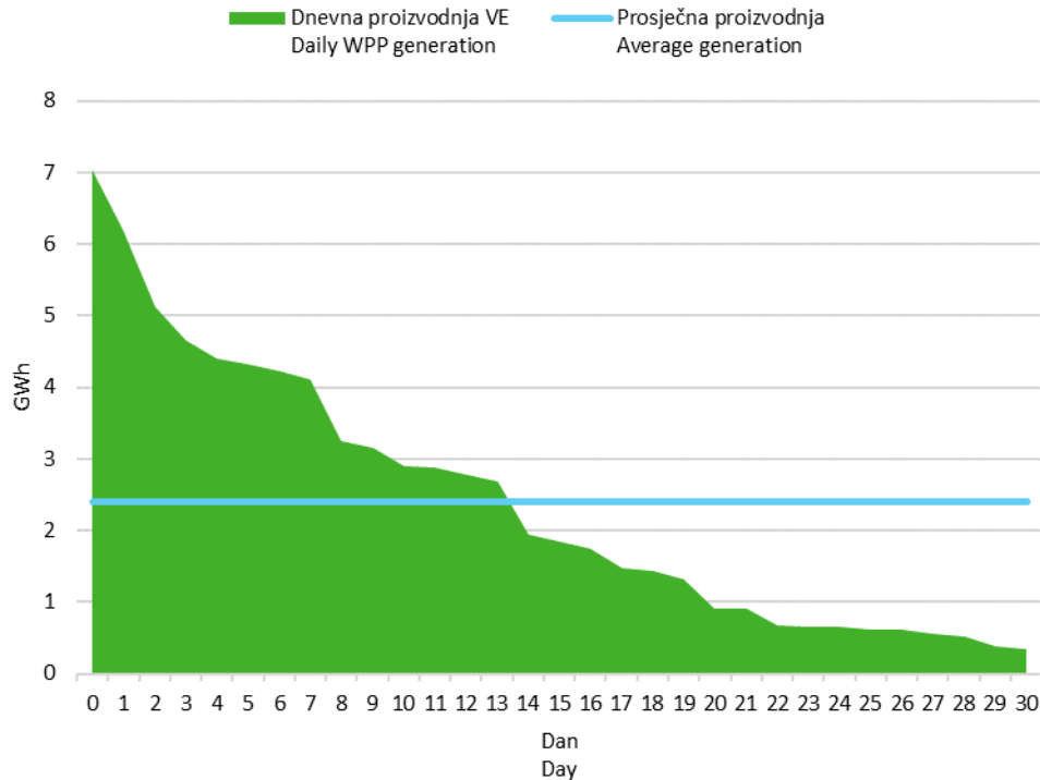
Slika 6 Krivulja trajanja dnevne proizvodnje vjetroelektrana u svibnju 2018. godine
