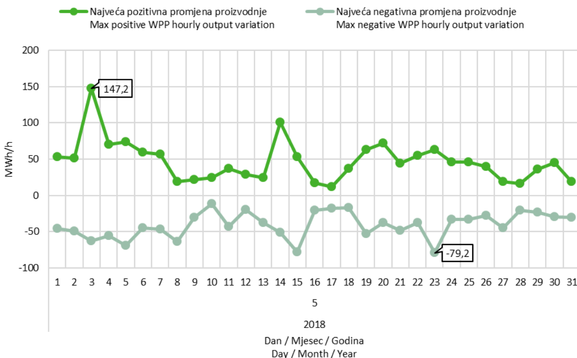
Slika 9 Maksimalna pozitivna i maksimalna negativna promjena satne proizvodnje VE u svibnju 2018. godine
