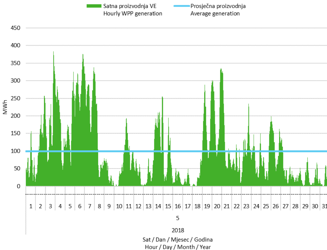
Slika 2 Satna proizvodnja svih vjetroelektrana u svibnju 2018. godine
