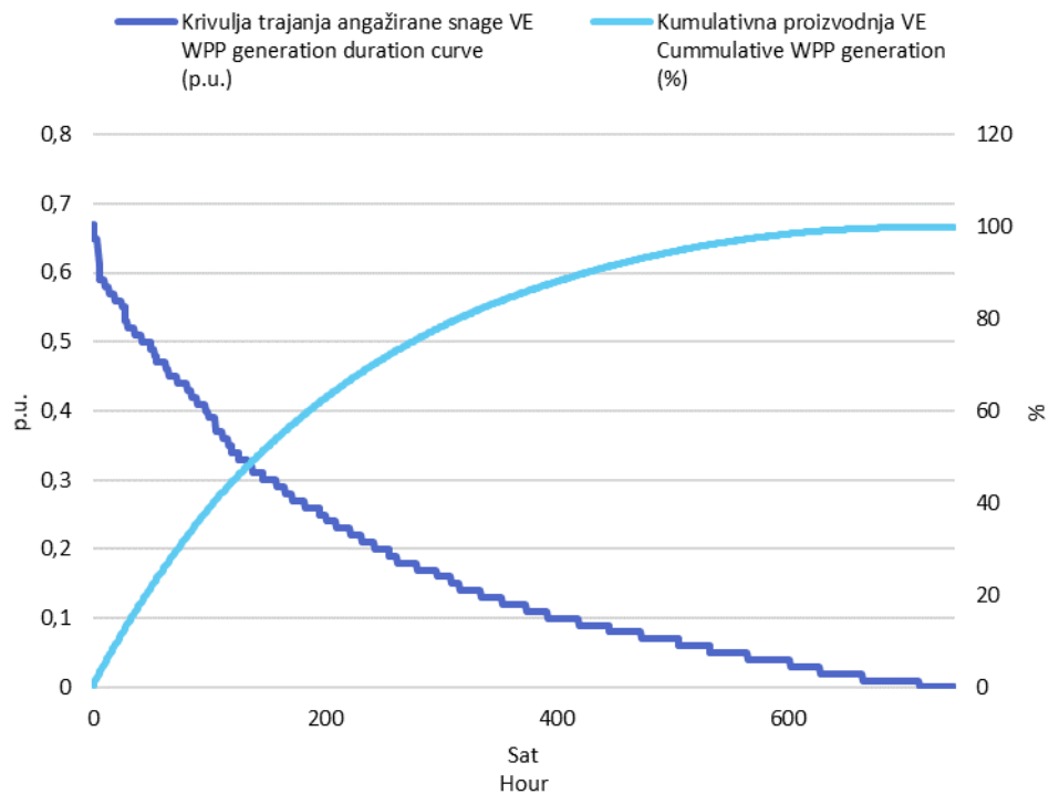
Slika 3 Krivulja trajanja angažirane snage svih VE i kumulativna proizvodnja VE u svibnju 2018. godine u jediničnim vrijednostima
