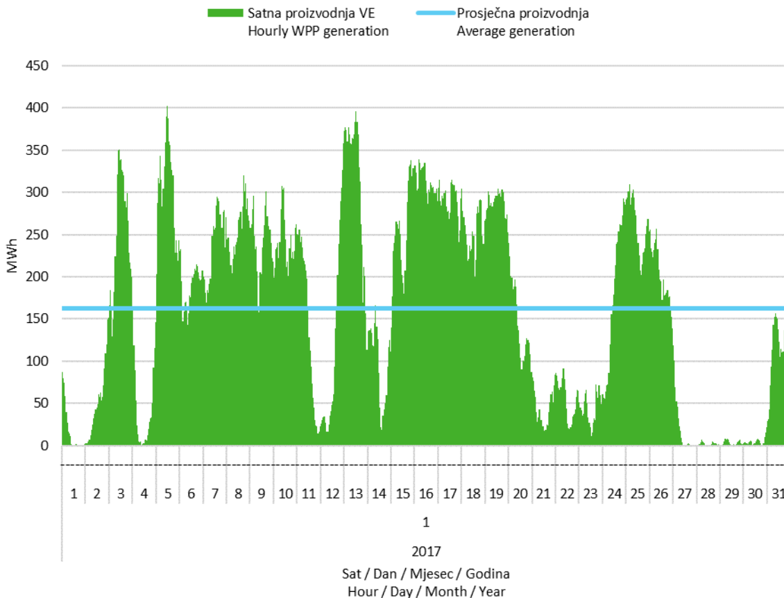
Slika 2 Satna proizvodnja svih vjetroelektrana u siječnju 2017. godine
