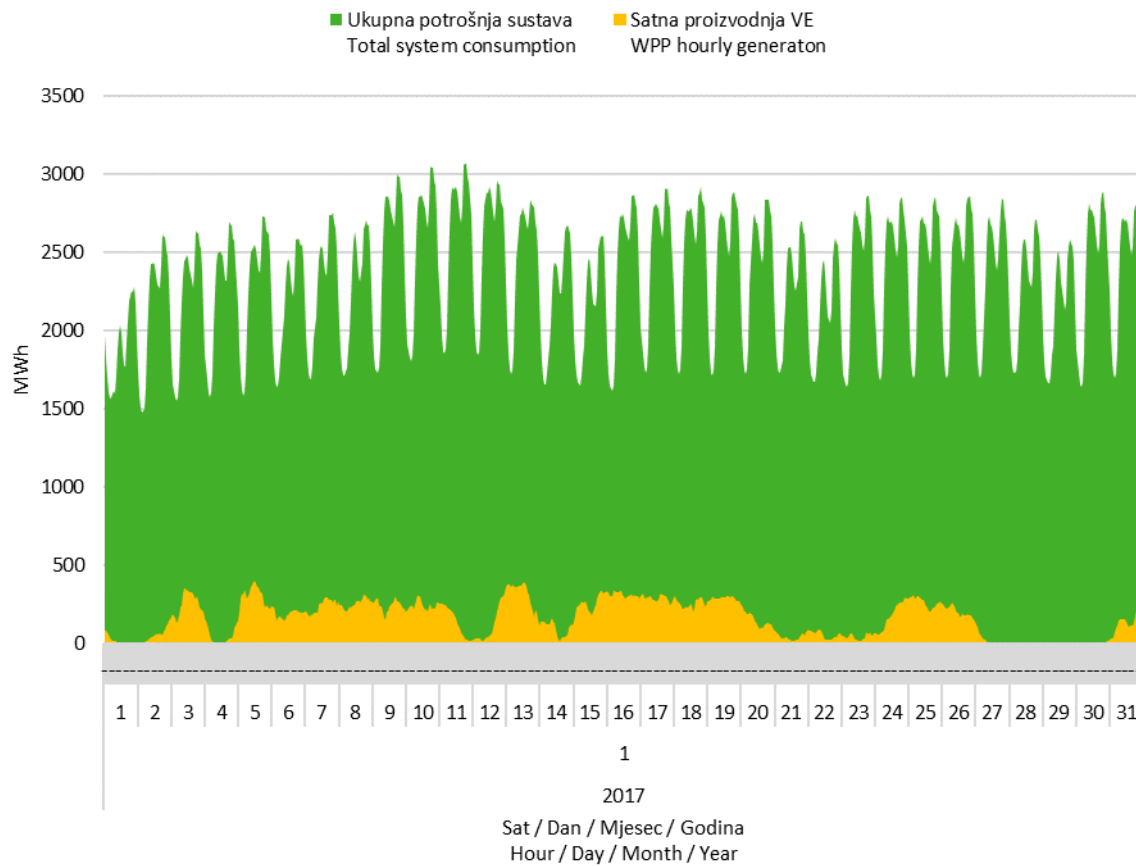
Slika 7 Usporedba satnog dijagrama opterećenja sustava i proizvodnje vjetroelektrana u siječnju 2017. godine
