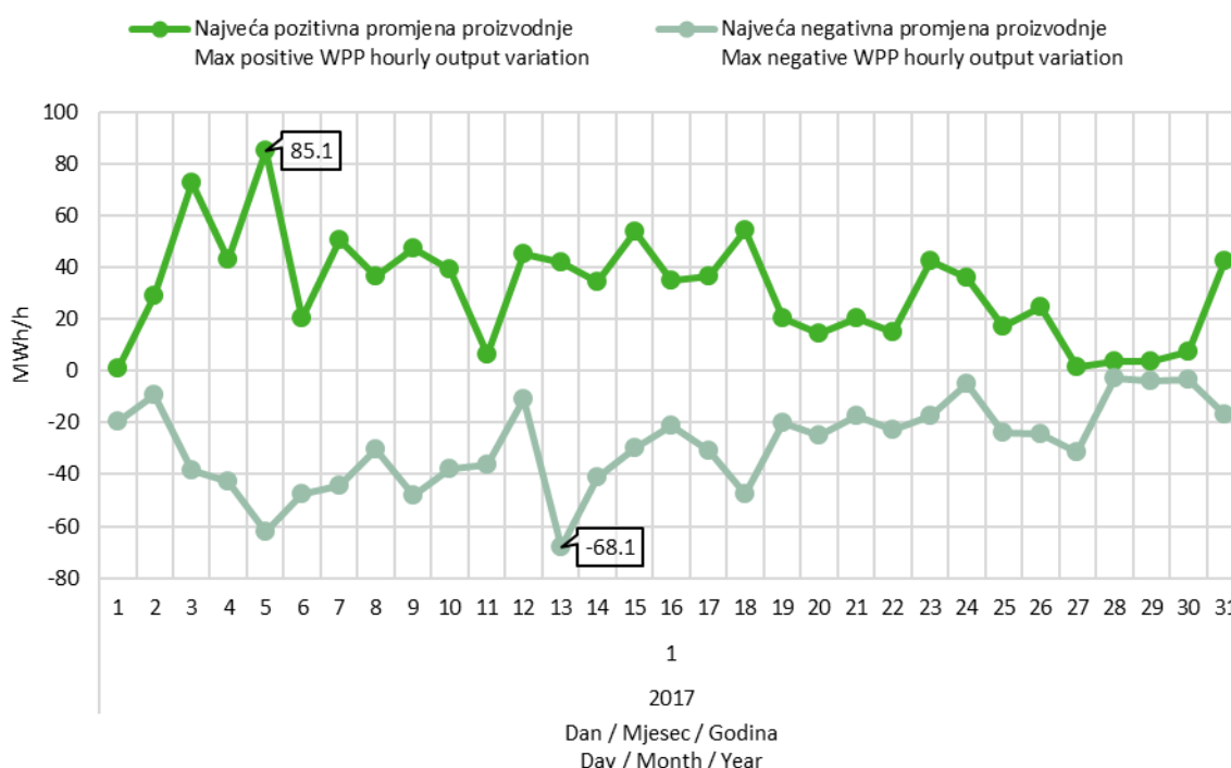
Slika 9 Maksimalna pozitivna i maksimalna negativna promjena satne proizvodnje VE u siječnju 2017. godine
