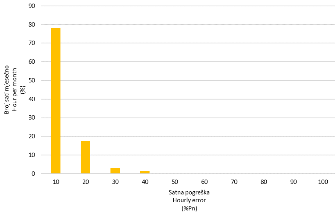
Slika 17 Frekvencija pojavljivanja pogreške prognoze satne proizvodnje svih VE u siječnju 2017. godine
