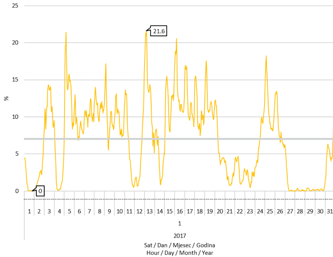
Slika 8 Udio proizvodnje vjetroelektrana u pokrivanju satnog opterećenja elektroenergetskog sustava u siječnju 2017. godine
