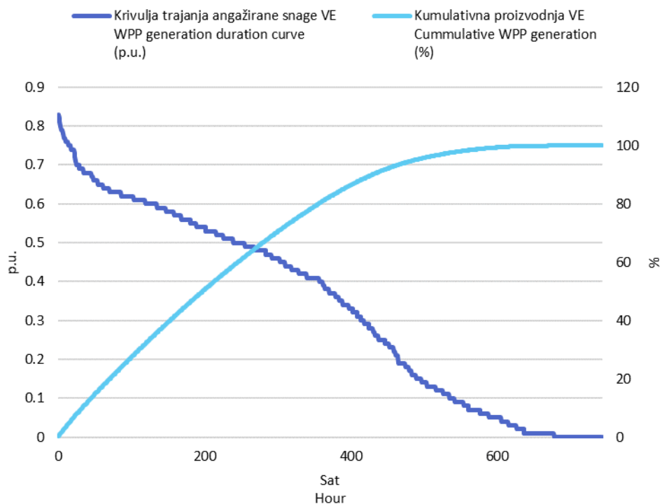
Slika 3 Krivulja trajanja angažirane snage svih VE i kumulativna proizvodnja VE u siječnju 2017. godine u jediničnim vrijednostima
