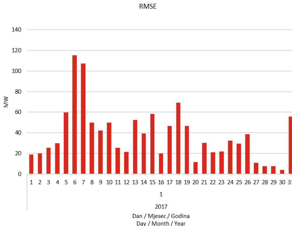
Slika 15 Korijen srednje kvadratne pogreške prognoze satne proizvodnje svih VE u siječnju 2017. godine
