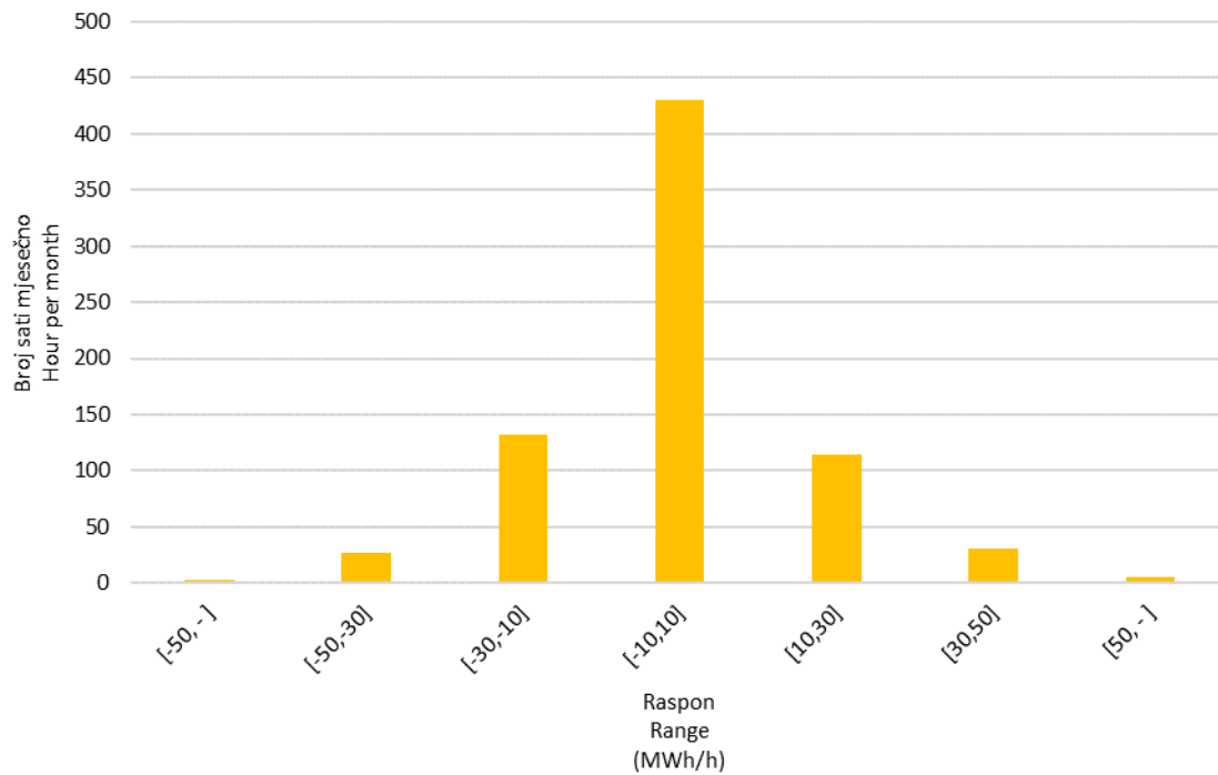
Slika 10 Statistička raspodjela satnih promjena proizvodnje VE u siječnju 2017. godine
