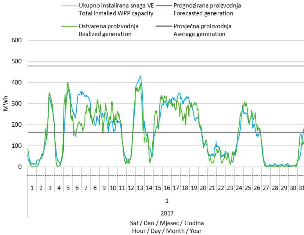
Slika 11 Prognozirana i ostvarena satna proizvodnja vjetroelektrana u siječnju 2017. godine
