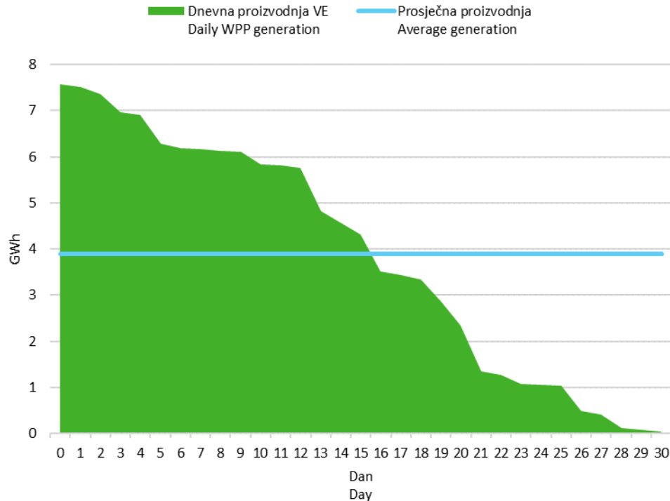
Slika 6 Krivulja trajanja dnevne proizvodnje vjetroelektrana u siječnju 2017. godine
