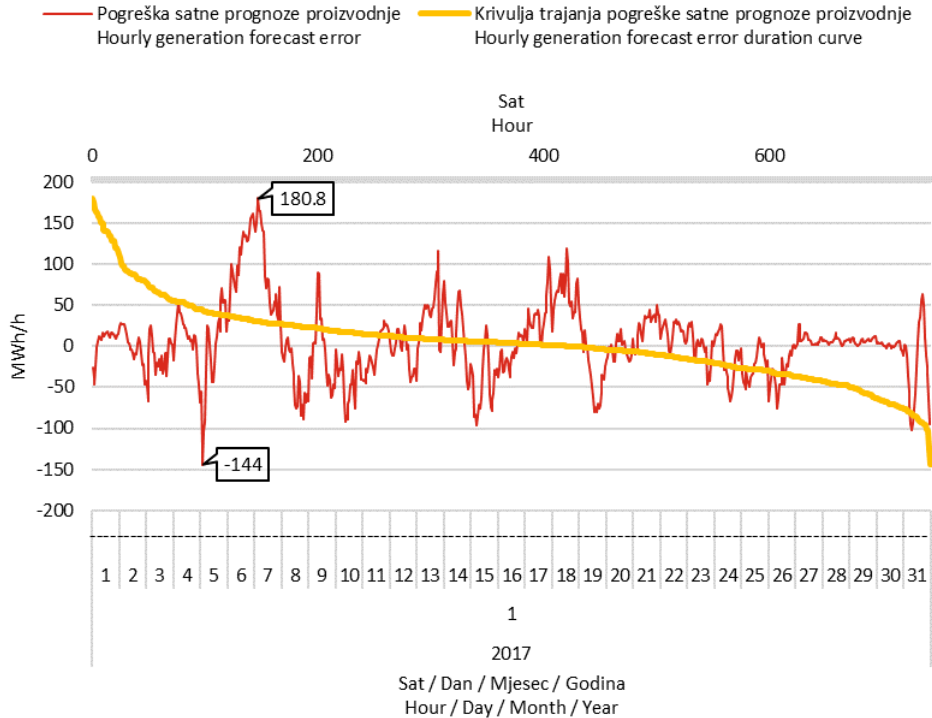
Slika 12 Razlika između prognozirane i ostvarene satne proizvodnje svih VE (pogreška prognoze) i pripadna krivulja trajanja u siječnju 2017. godine
