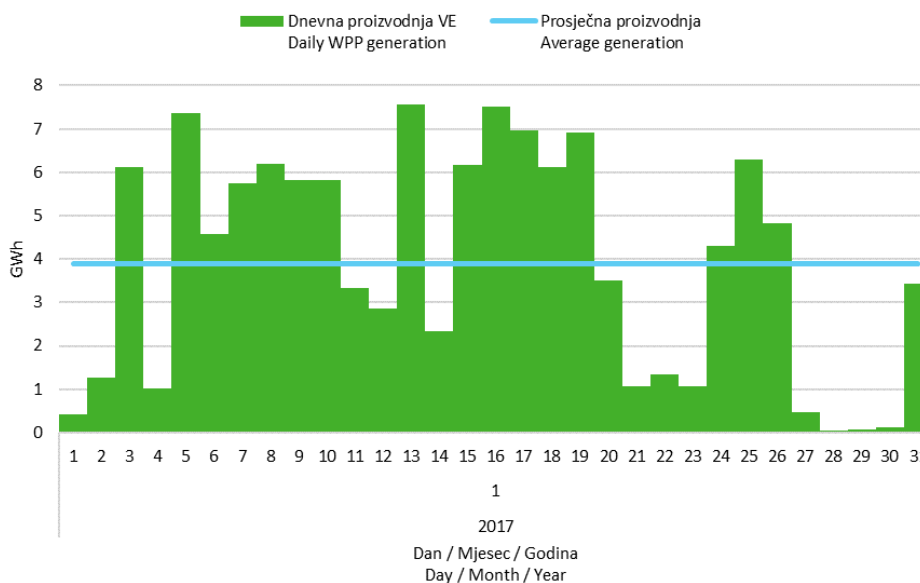
Slika 5 Dnevna proizvodnja svih vjetroelektrana u siječnju 2017. godine
