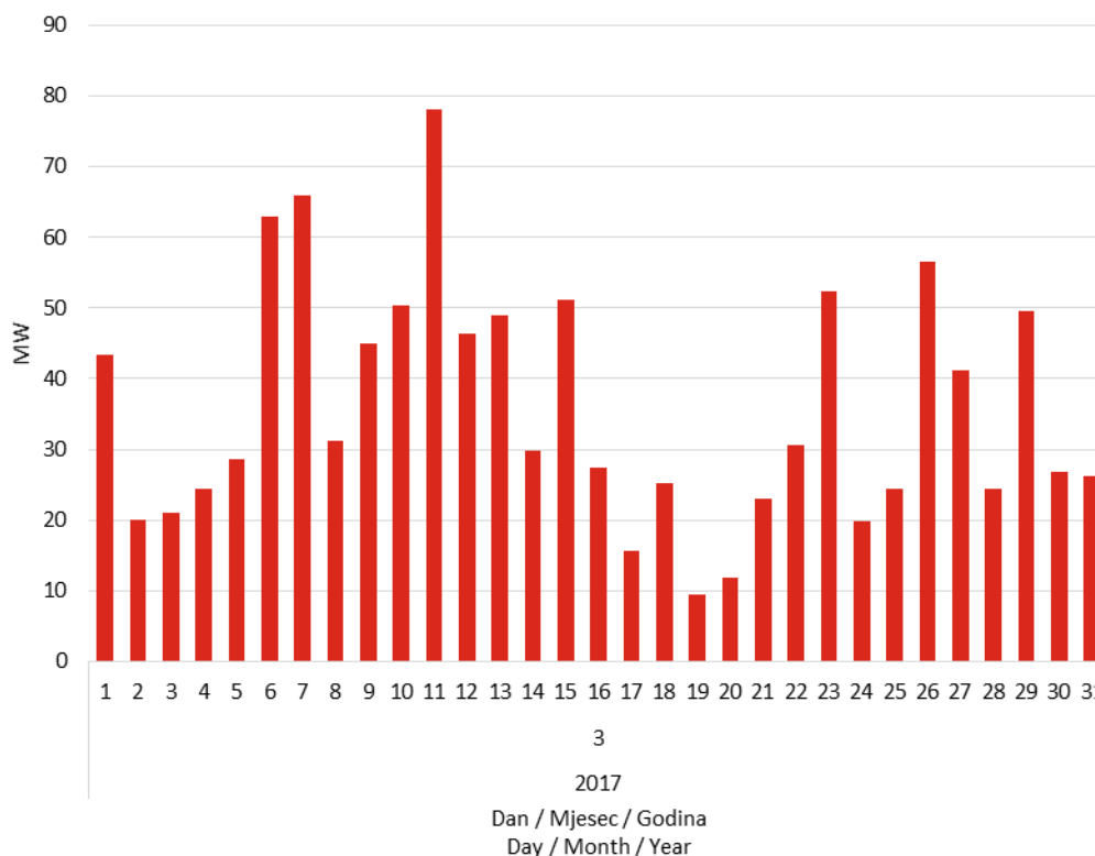
Slika 15 Korijen srednje kvadratne pogreške prognoze satne proizvodnje svih VE u ožujku 2017. godine
