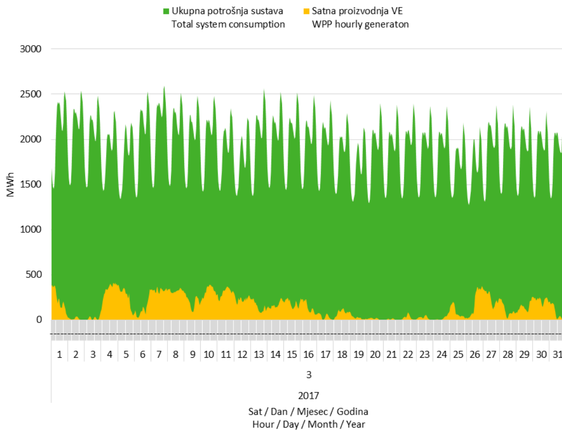
Slika 7 Usporedba satnog dijagrama opterećenja sustava i proizvodnje vjetroelektrana u ožujku 2017. godine
