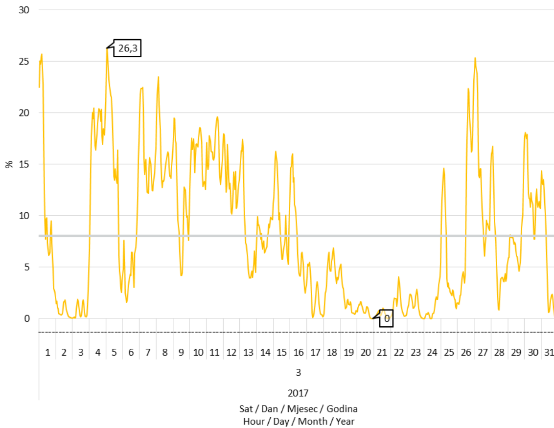
Slika 8 Udio proizvodnje vjetroelektrana u pokrivanju satnog opterećenja elektroenergetskog sustava u ožujku 2017. godine
