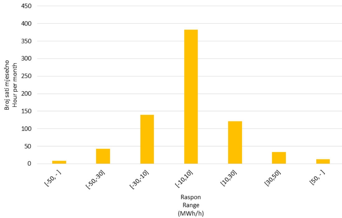
Slika 10 Statistička raspodjela satnih promjena proizvodnje VE u ožujku 2017. godine
