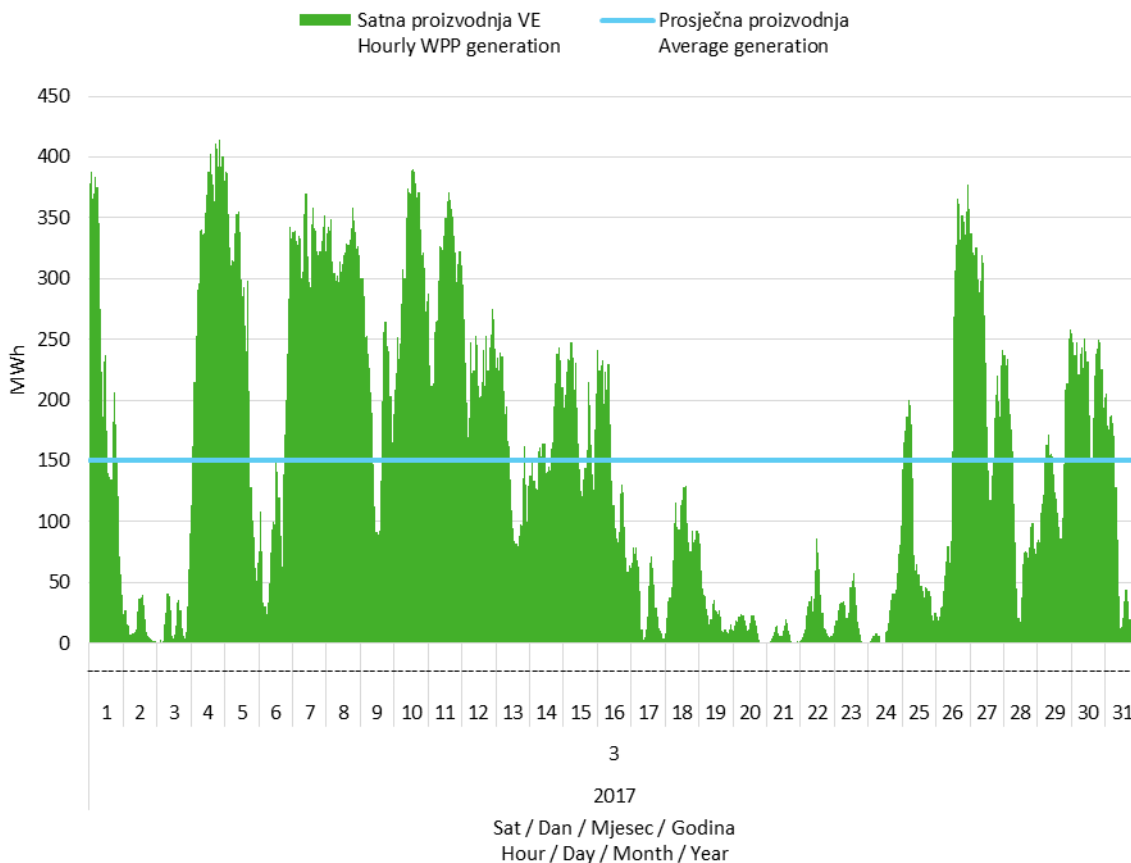
Slika 2 Satna proizvodnja svih vjetroelektrana u ožujku 2017. godine
