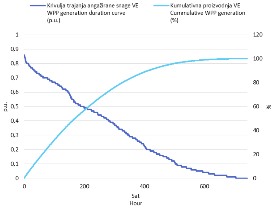
Slika 3 Krivulja trajanja angažirane snage svih VE i kumulativna proizvodnja VE u ožujku 2017. godine u jediničnim vrijednostima
