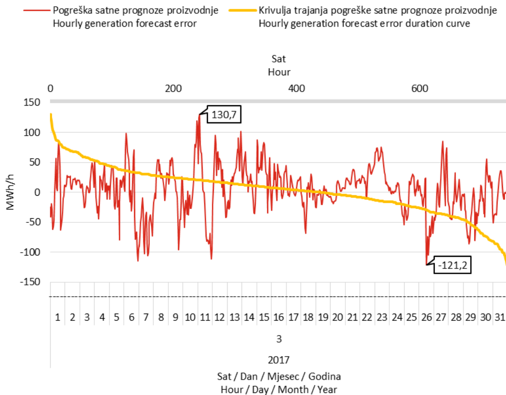
Slika 12 Razlika između prognozirane i ostvarene satne proizvodnje svih VE (pogreška prognoze) i pripadna krivulja trajanja u ožujku 2017. godine
