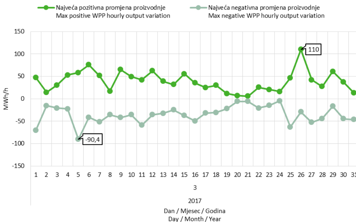
Slika 9 Maksimalna pozitivna i maksimalna negativna promjena satne proizvodnje VE u ožujku 2017. godine
