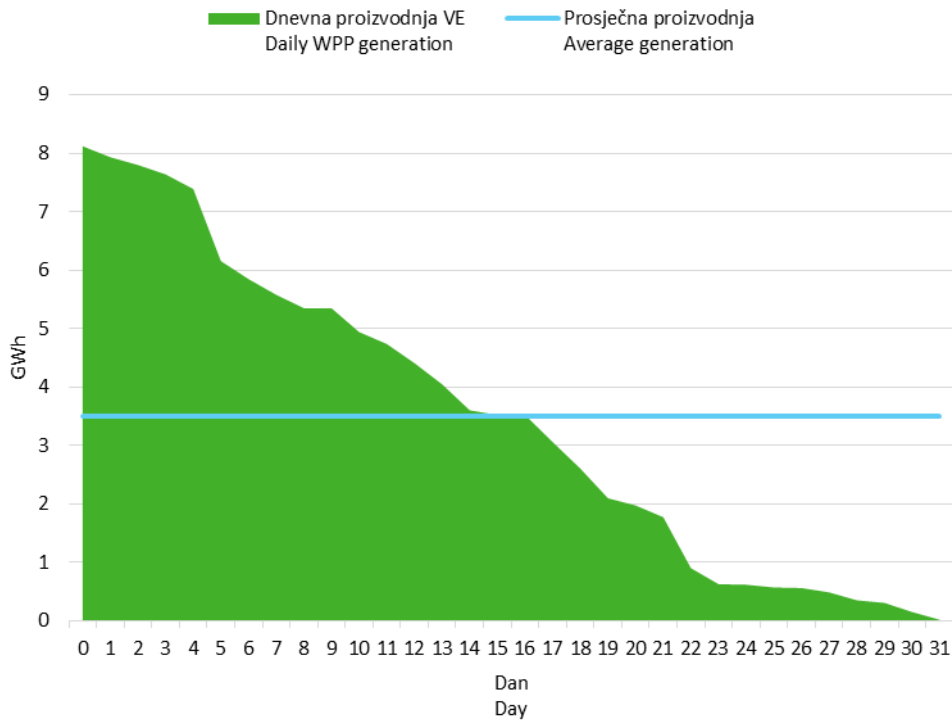
Slika 6 Krivulja trajanja dnevne proizvodnje vjetroelektrana u ožujku 2017. godine
