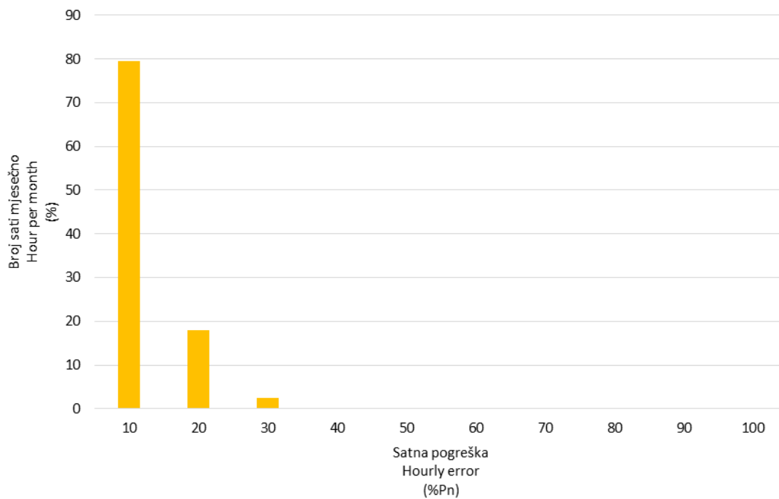
Slika 17 Frekvencija pojavljivanja pogreške prognoze satne proizvodnje svih VE u ožujku 2017. godine
