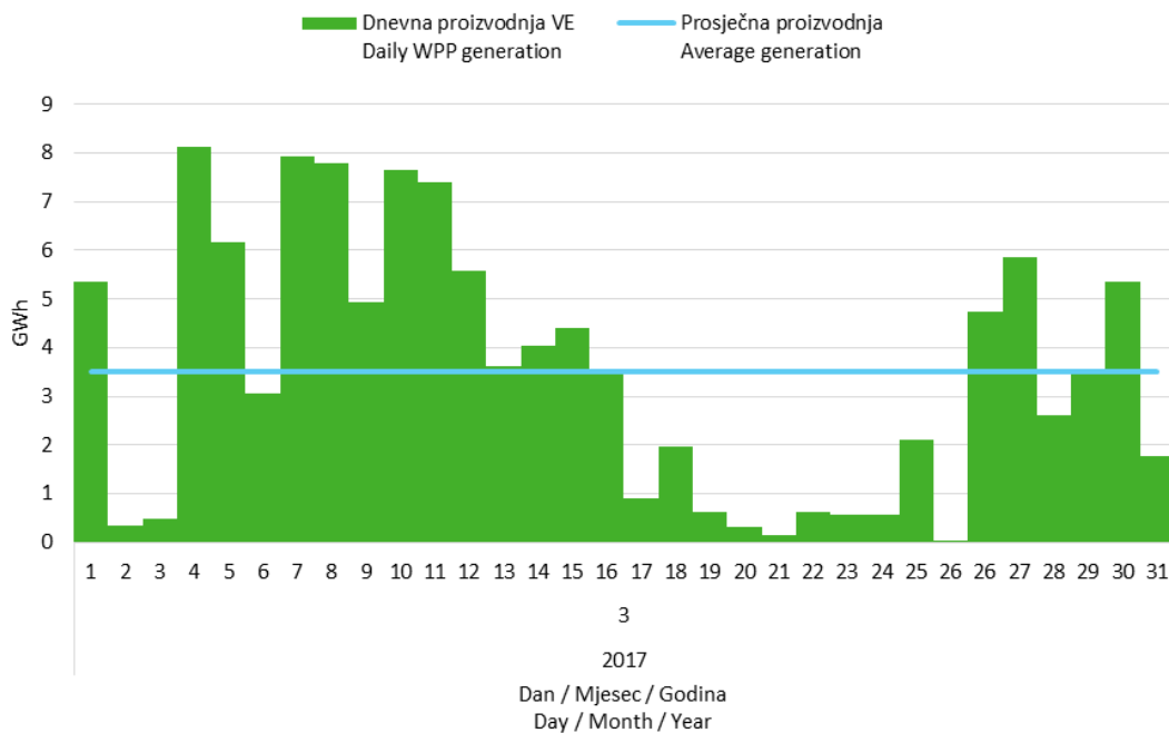
Slika 5 Dnevna proizvodnja svih vjetroelektrana u ožujku 2017. godine
