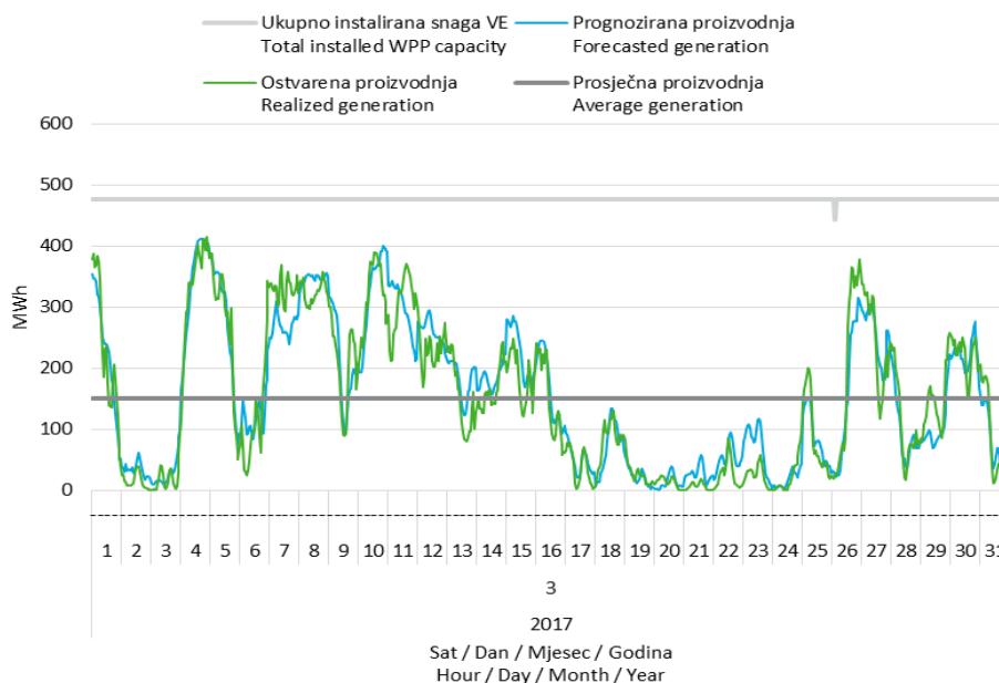
Slika 11 Prognozirana i ostvarena satna proizvodnja vjetroelektrana u ožujku 2017. godine
