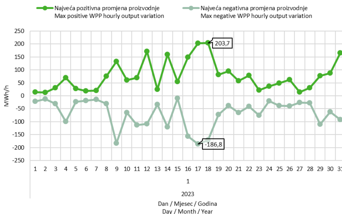
Slika 9 Maksimalna pozitivna i maksimalna negativna promjena satne proizvodnje VE u siječnju 2023. godine
