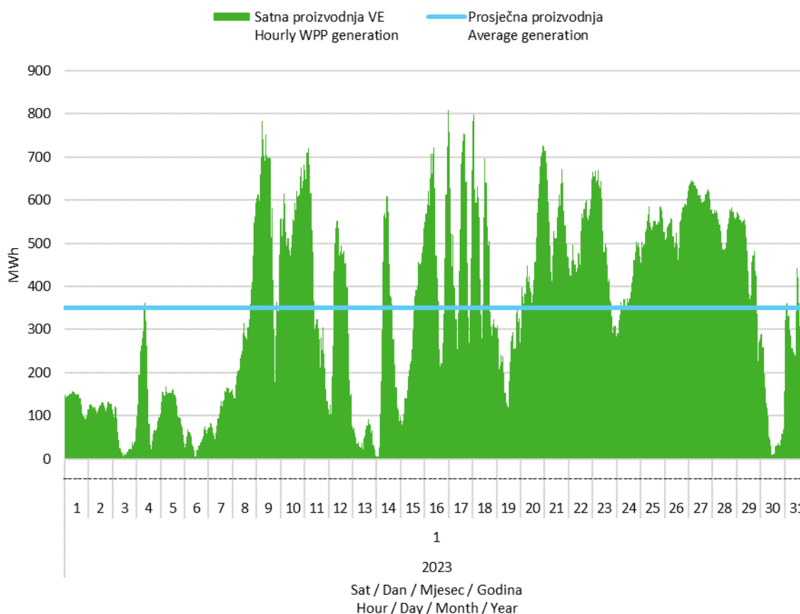
Slika 2 Satna proizvodnja svih vjetroelektrana u siječnju 2023. godine
