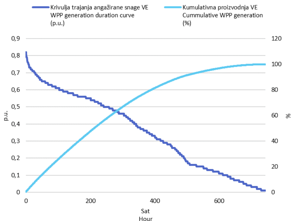
Slika 3 Krivulja trajanja angažirane snage svih VE i kumulativna proizvodnja VE u siječnju 2023. godine u jediničnim vrijednostima
