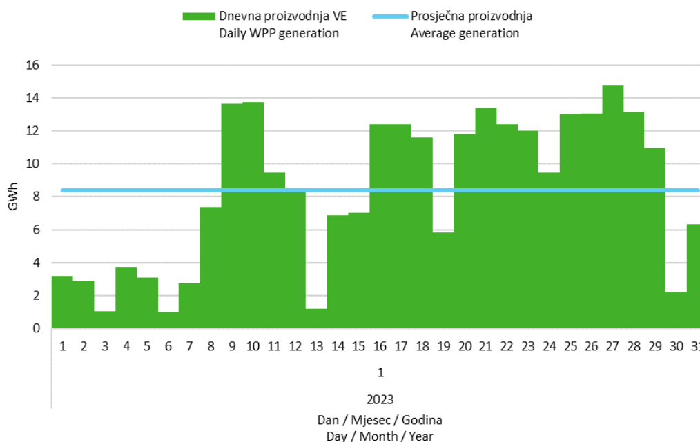
Slika 5 Dnevna proizvodnja svih vjetroelektrana u siječnju 2023. godine
