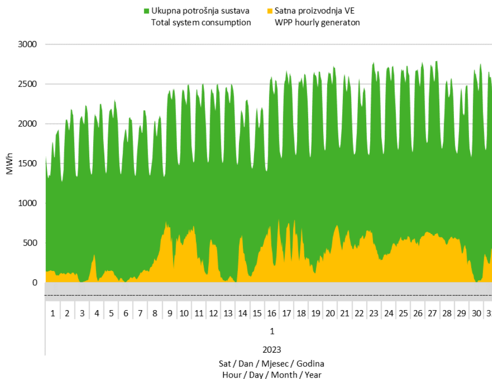
Slika 7 Usporedba satnog dijagrama opterećenja sustava i proizvodnje vjetroelektrana u siječnju 2023. godine
