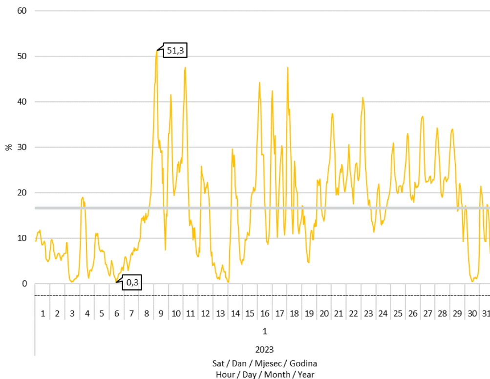
Slika 8 Udio proizvodnje vjetroelektrana u pokrivanju satnog opterećenja elektroenergetskog sustava u siječnju 2023. godine
