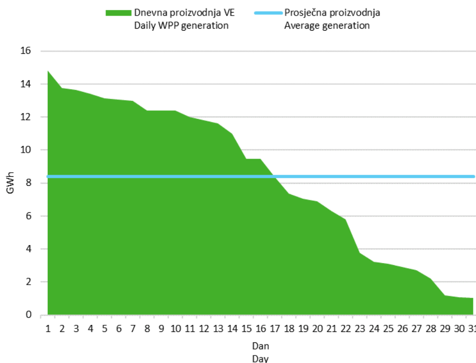
Slika 6 Krivulja trajanja dnevne proizvodnje vjetroelektrana u siječnju 2023. godine
