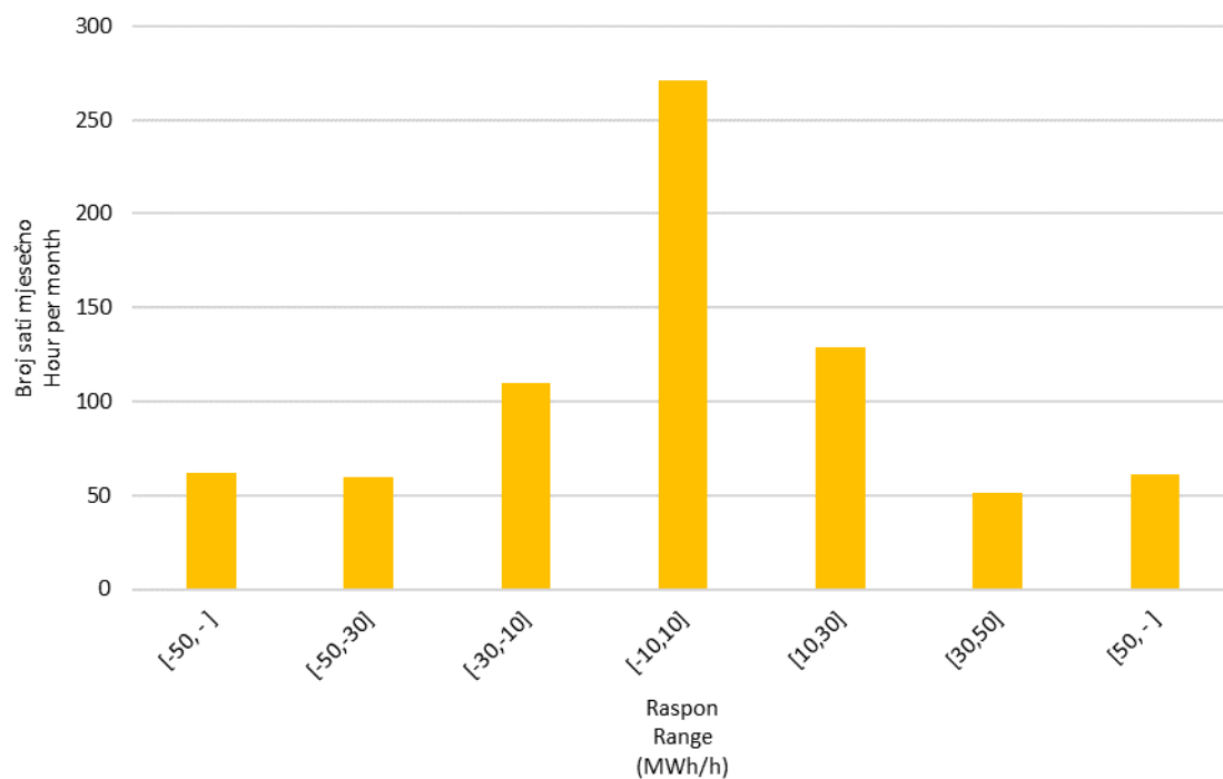
Slika 10 Statistička raspodjela satnih promjena proizvodnje VE u siječnju 2023. godine
