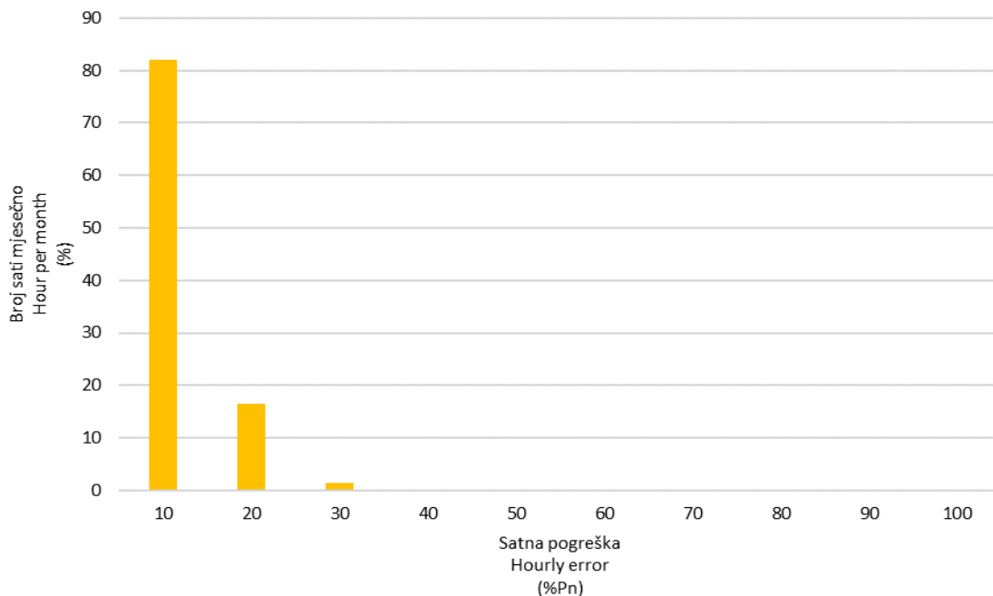
Slika 17 Frekvencija pojavljivanja pogreške prognoze satne proizvodnje svih VE u studenom 2017. godine
