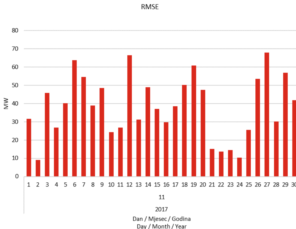
Slika 15 Korijen srednje kvadratne pogreške prognoze satne proizvodnje svih VE u studenom 2017. godine
