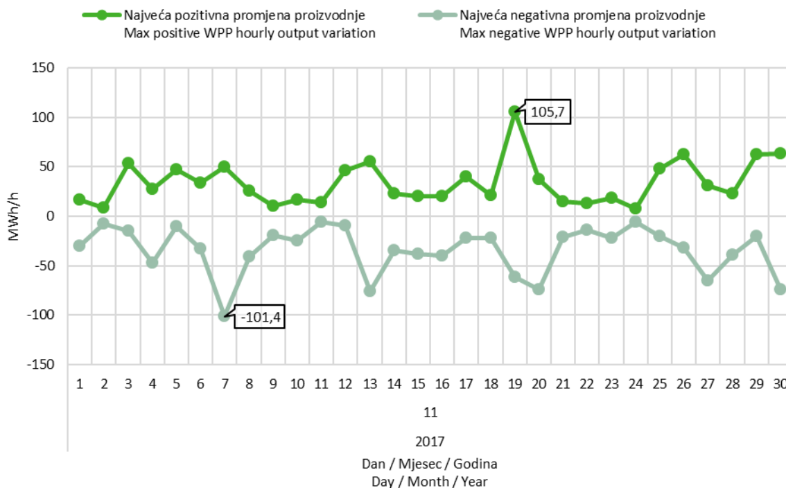
Slika 9 Maksimalna pozitivna i maksimalna negativna promjena satne proizvodnje VE u studenom 2017. godine
