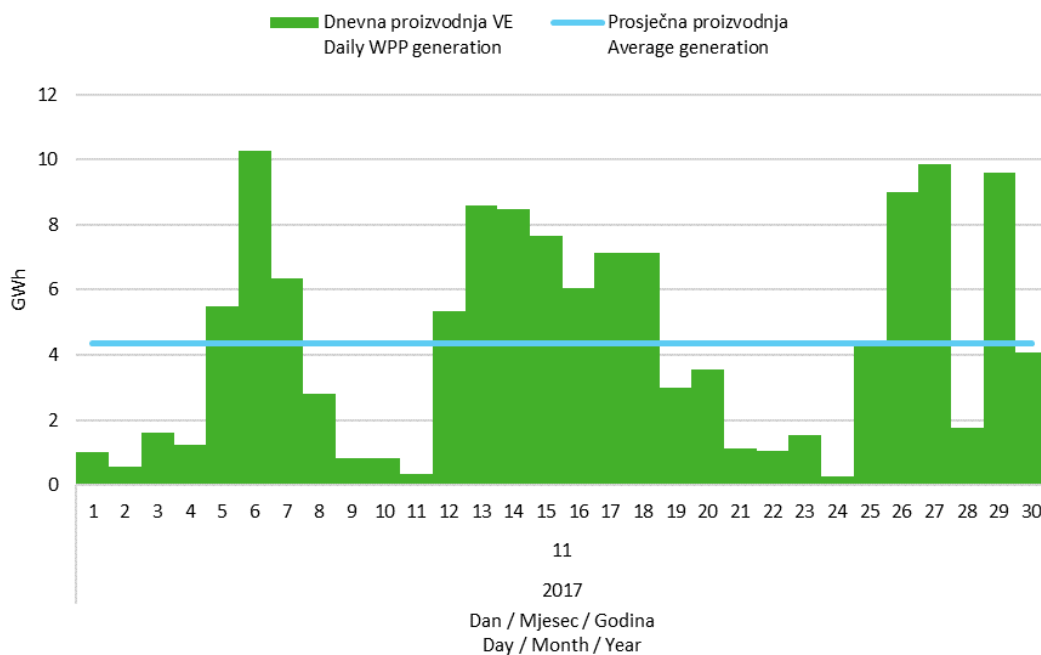
Slika 5 Dnevna proizvodnja svih vjetroelektrana u studenom 2017. godine Figure 5 Daily generation of all wind power plants in November 2017
