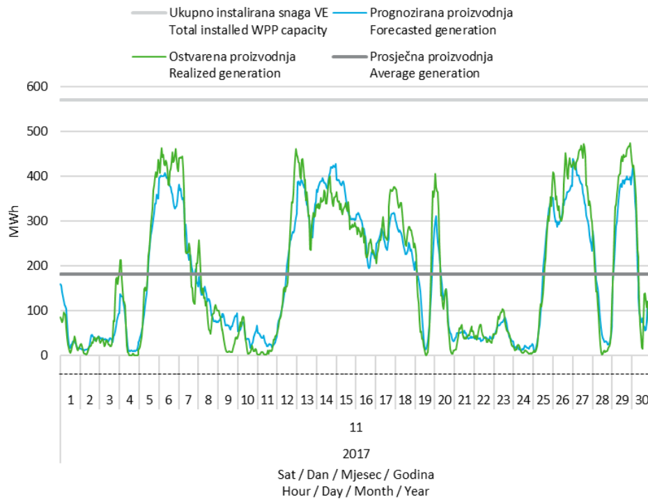
Slika 11 Prognozirana i ostvarena satna proizvodnja vjetroelektrana u studenom 2017. godine
