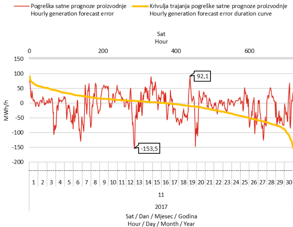
Slika 12 Razlika između prognozirane i ostvarene satne proizvodnje svih VE (pogreška prognoze) i pripadna krivulja trajanja u studenom 2017. godine
