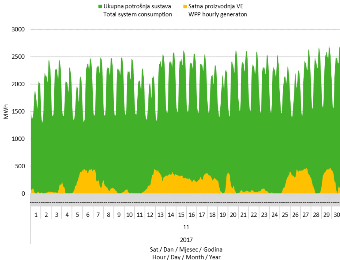
Slika 7 Usporedba satnog dijagrama opterećenja sustava i proizvodnje vjetroelektrana u studenom 2017. godine
