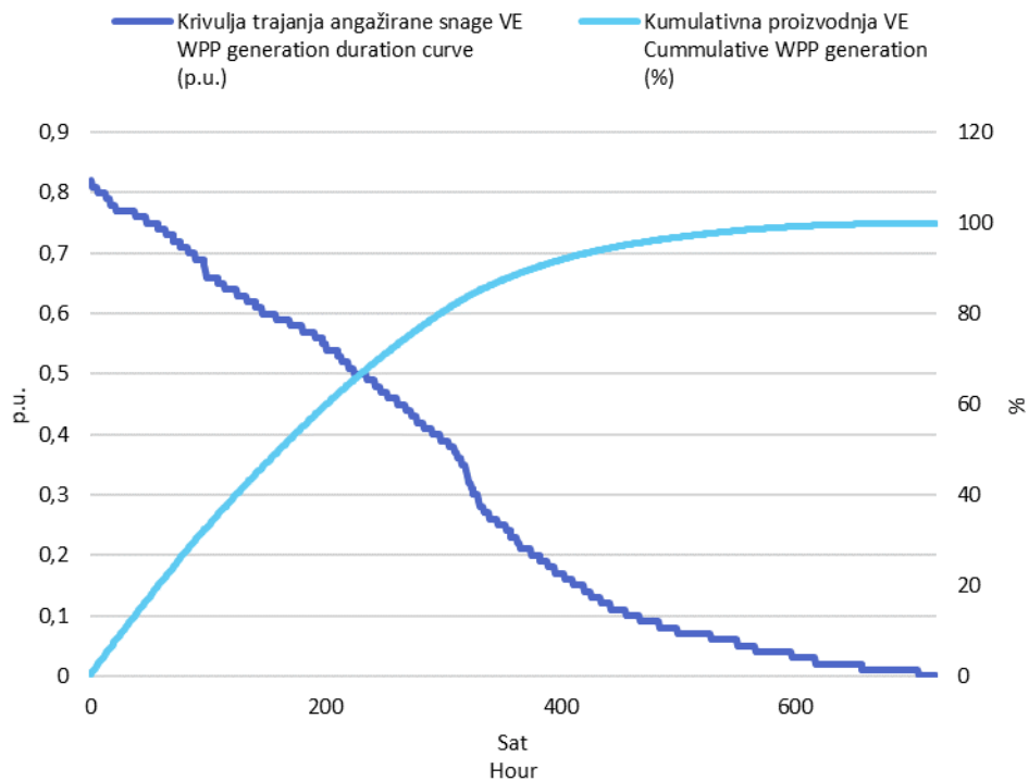
Slika 3 Krivulja trajanja angažirane snage svih VE i kumulativna proizvodnja VE u studenom 2017. godine u jediničnim vrijednostima
