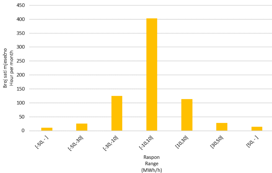
Slika 10 Statistička raspodjela satnih promjena proizvodnje VE u studenom 2017. godine
