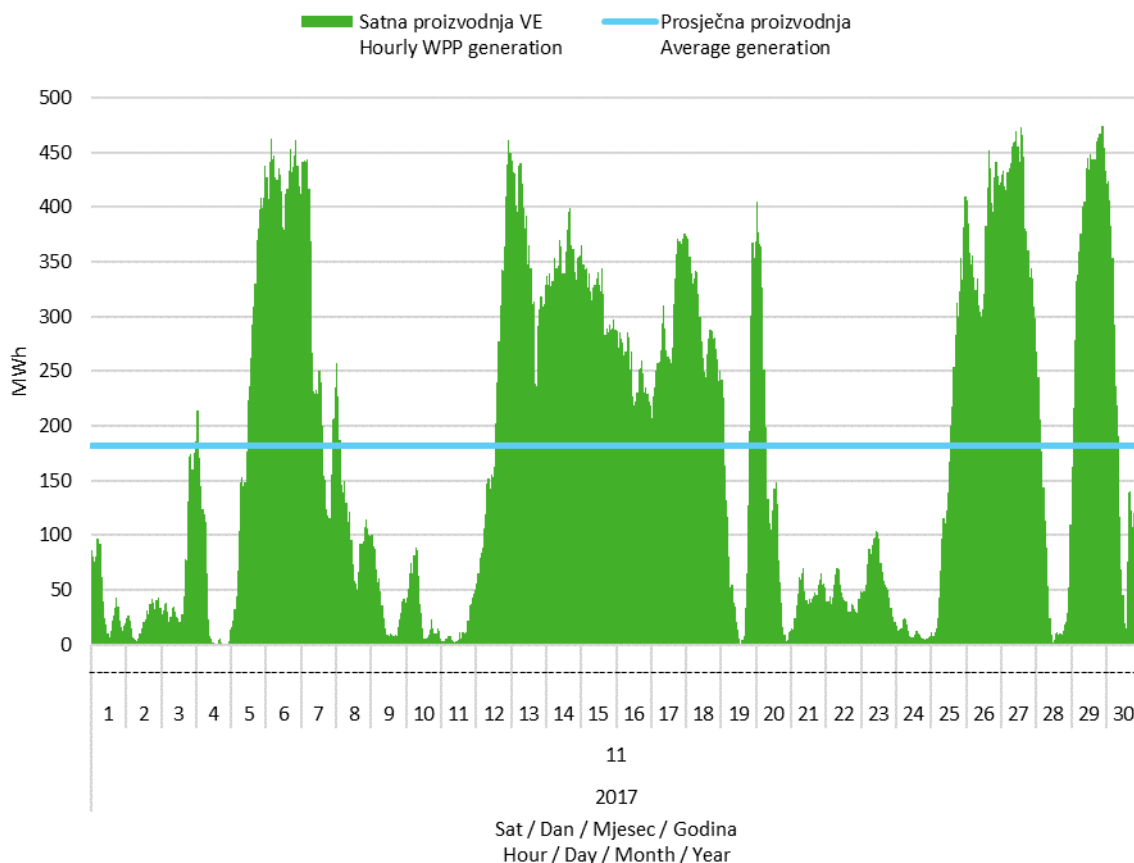
Slika 2 Satna proizvodnja svih vjetroelektrana u studenom 2017. godine
