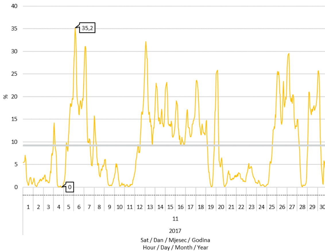
Slika 8 Udio proizvodnje vjetroelektrana u pokrivanju satnog opterećenja elektroenergetskog sustava u studenom 2017. godine
