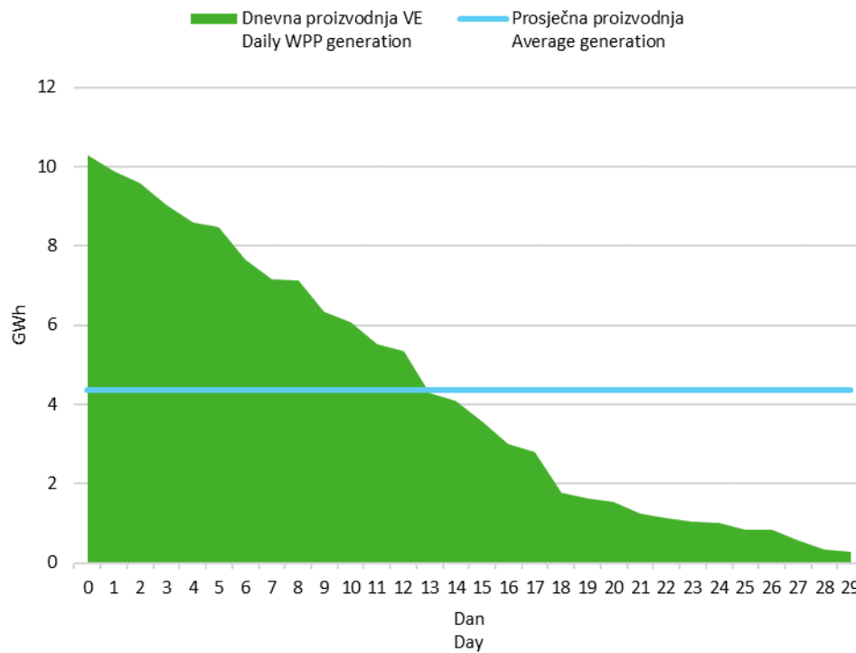
Slika 6 Krivulja trajanja dnevne proizvodnje vjetroelektrana u studenom 2017. godine
