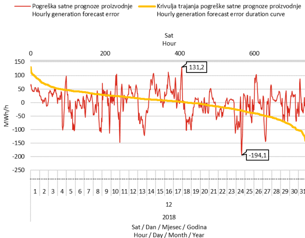
Slika 12 Razlika između prognozirane i ostvarene satne proizvodnje svih VE (pogreška prognoze) i pripadna krivulja trajanja u prosincu 2018. godine
