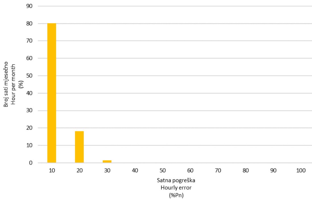
Slika 17 Frekvencija pojavljivanja pogreške prognoze satne proizvodnje svih VE u prosincu 2018. godine
