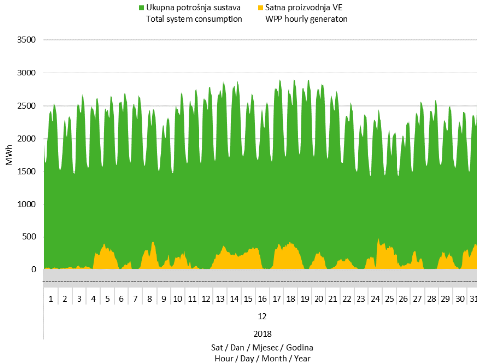
Slika 7 Usporedba satnog dijagrama opterećenja sustava i proizvodnje vjetroelektrana u prosincu 2018. godine
