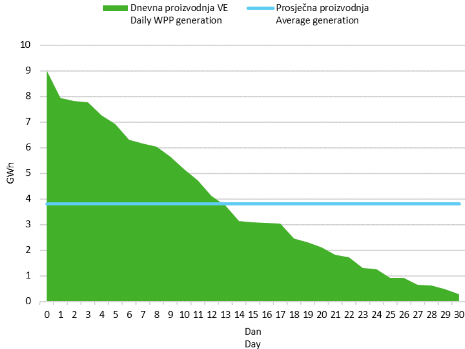
Slika 6 Krivulja trajanja dnevne proizvodnje vjetroelektrana u prosincu 2018. godine
