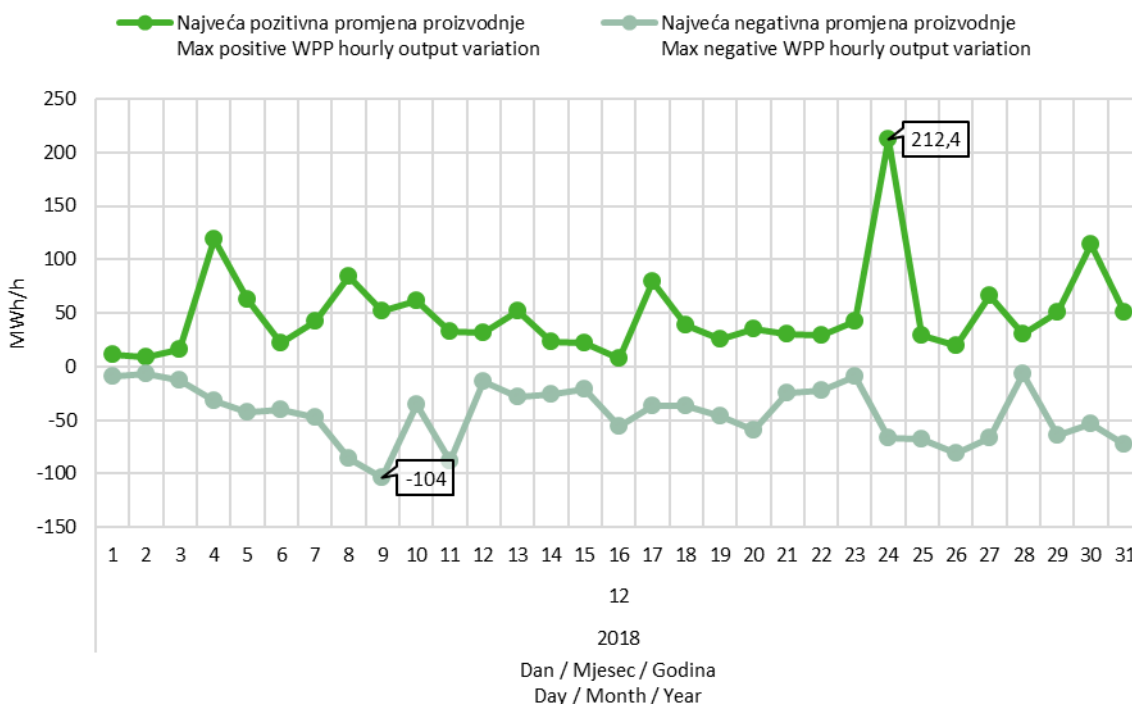
Slika 9 Maksimalna pozitivna i maksimalna negativna promjena satne proizvodnje VE u prosincu 2018. godine
