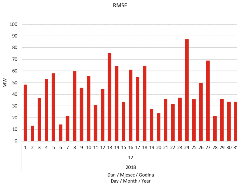
Slika 15 Korijen srednje kvadratne pogreške prognoze satne proizvodnje svih VE u prosincu 2018. godine
