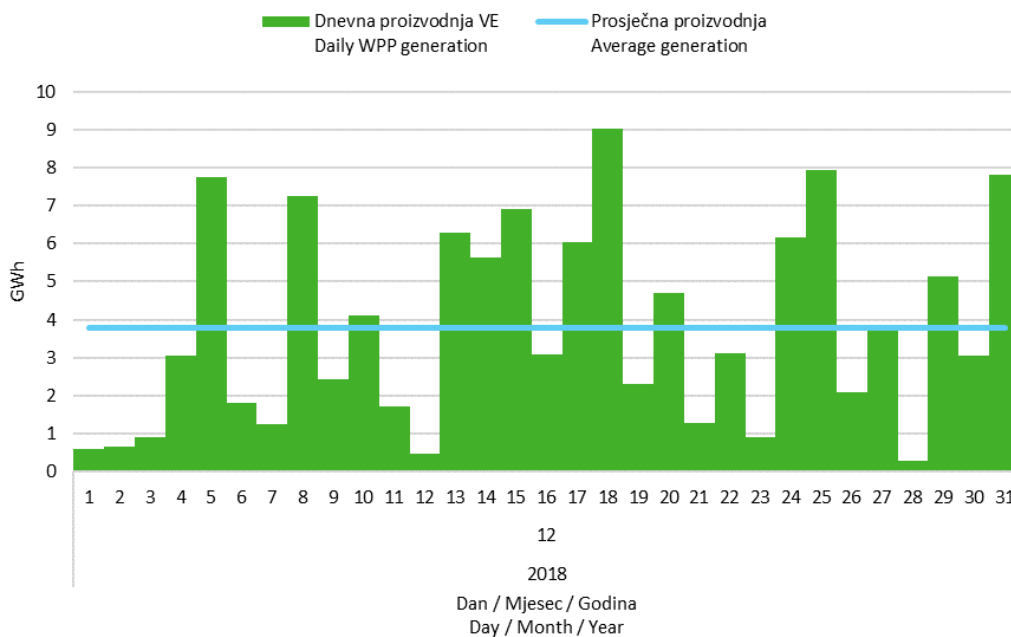
Slika 5 Dnevna proizvodnja svih vjetroelektrana u prosincu 2018. godine
