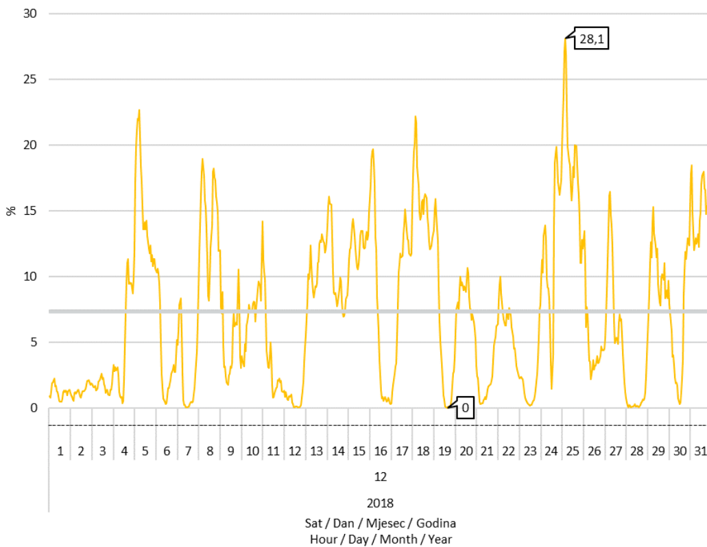
Slika 8 Udio proizvodnje vjetroelektrana u pokrivanju satnog opterećenja elektroenergetskog sustava u prosincu 2018. godine
