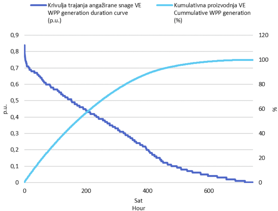
Slika 3 Krivulja trajanja angažirane snage svih VE i kumulativna proizvodnja VE u prosincu 2018. godine u jediničnim vrijednostima
