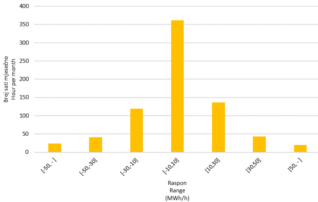
Slika 10 Statistička raspodjela satnih promjena proizvodnje VE u prosincu 2018. godine
