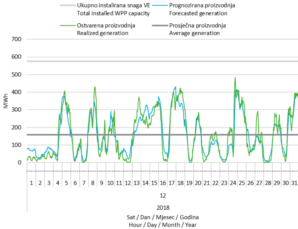
Slika 11 Prognozirana i ostvarena satna proizvodnja vjetroelektrana u prosincu 2018. godine
