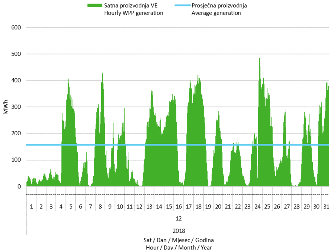
Slika 2 Satna proizvodnja svih vjetroelektrana u prosincu 2018. godine
