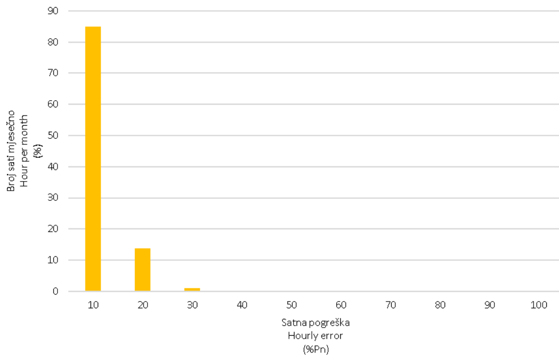
Slika 17 Frekvencija pojavljivanja pogreške prognoze satne proizvodnje svih VE u rujnu 2018. godine
