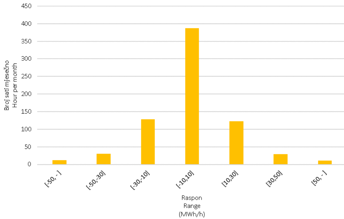
Slika 10 Statistička raspodjela satnih promjena proizvodnje VE u rujnu 2018. godine Figure 10 Statistical distribution of WPP hourly output variations in September 2018
