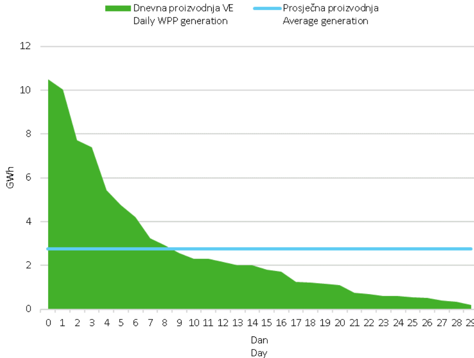
Slika 6 Krivulja trajanja dnevne proizvodnje vjetroelektrana u rujnu 2018. godine
