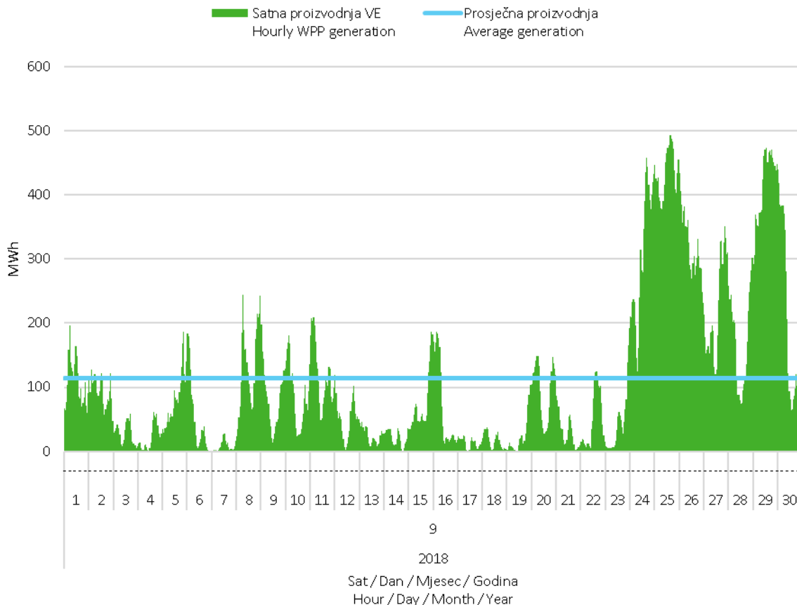
Slika 2 Satna proizvodnja svih vjetroelektrana u rujnu 2018. godine
