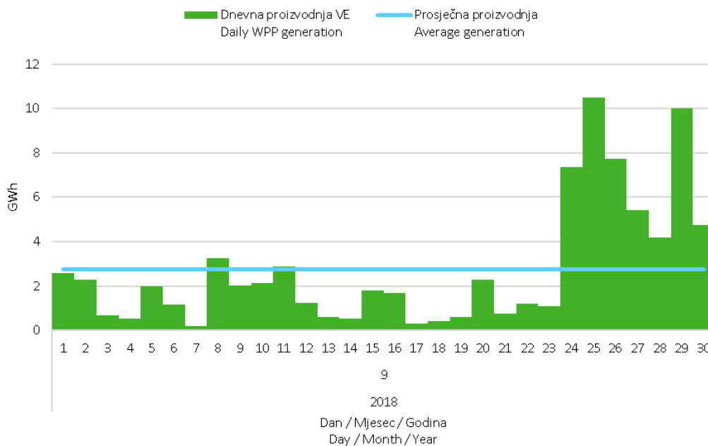
Slika 5 Dnevna proizvodnja svih vjetroelektrana u rujnu 2018. godine
