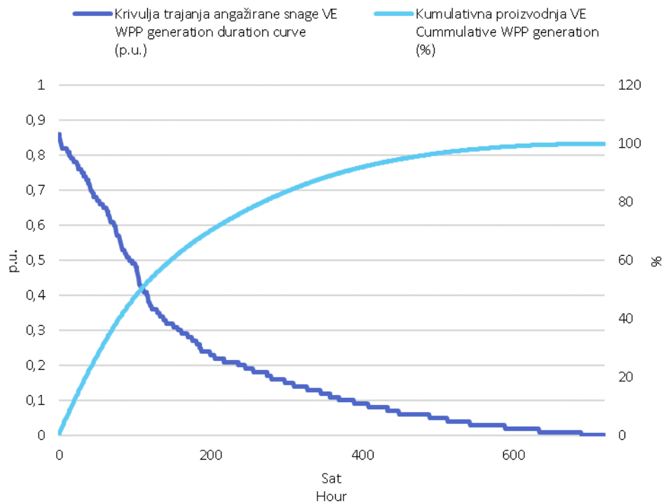
Slika 3 Krivulja trajanja angažirane snage svih VE i kumulativna proizvodnja VE u rujnu 2018. godine u jediničnim vrijednostima
