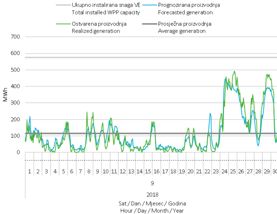
Slika 11 Prognozirana i ostvarena satna proizvodnja vjetroelektrana u rujnu 2018. godine
