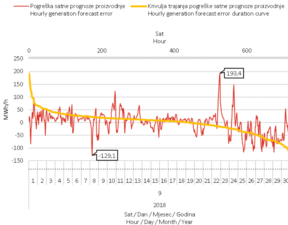
Slika 12 Razlika između prognozirane i ostvarene satne proizvodnje svih VE (pogreška prognoze) i pripadna krivulja trajanja u rujnu 2018. godine
