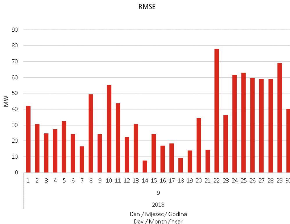
Slika 15 Korijen srednje kvadratne pogreške prognoze satne proizvodnje svih VE u rujnu 2018. godine
