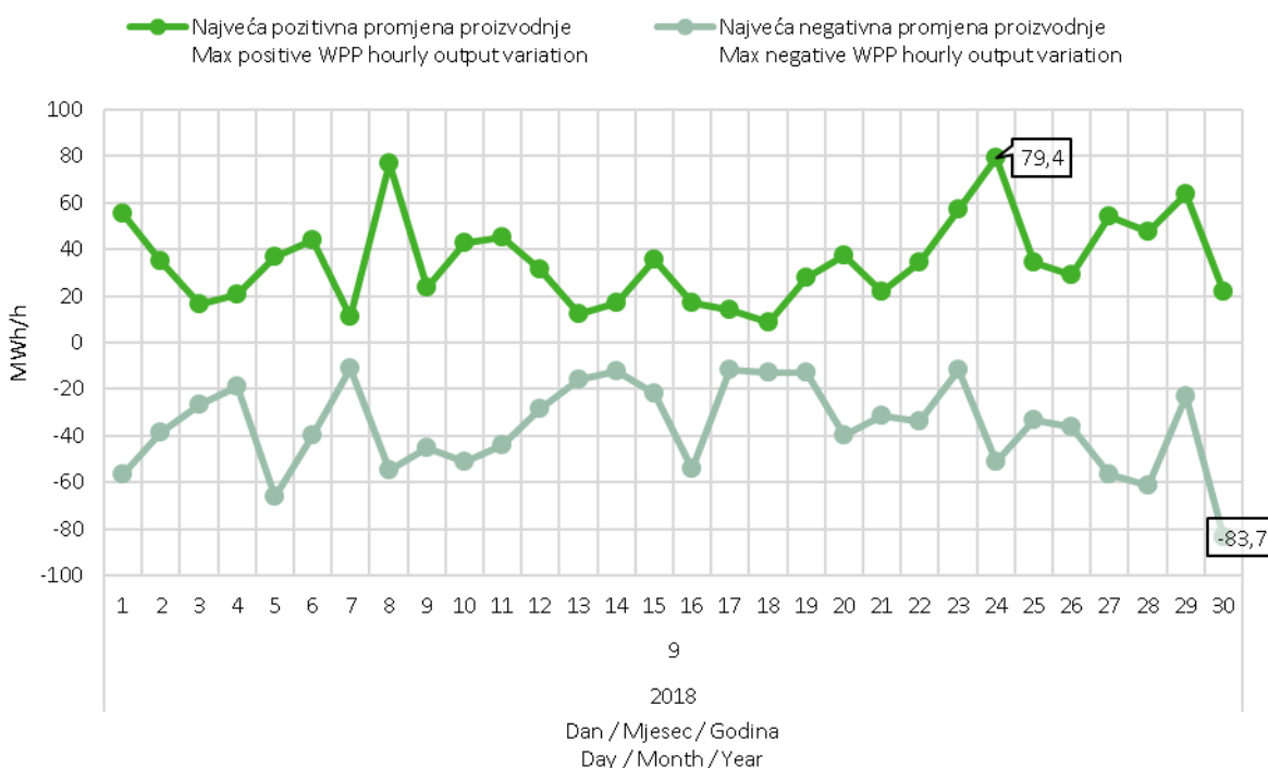
Slika 9 Maksimalna pozitivna i maksimalna negativna promjena satne proizvodnje VE u rujnu 2018. godine
