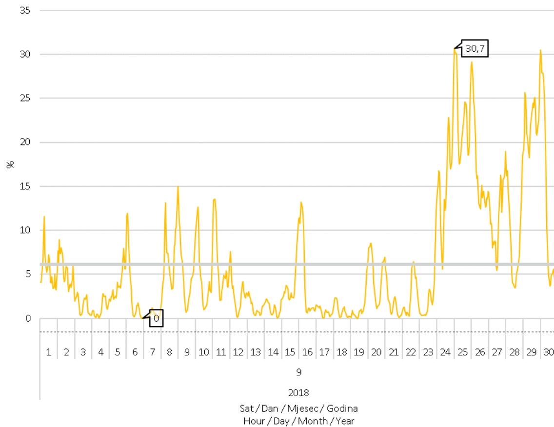
Slika 8 Udio proizvodnje vjetroelektrana u pokrivanju satnog opterećenja elektroenergetskog sustava u rujnu 2018. godine
