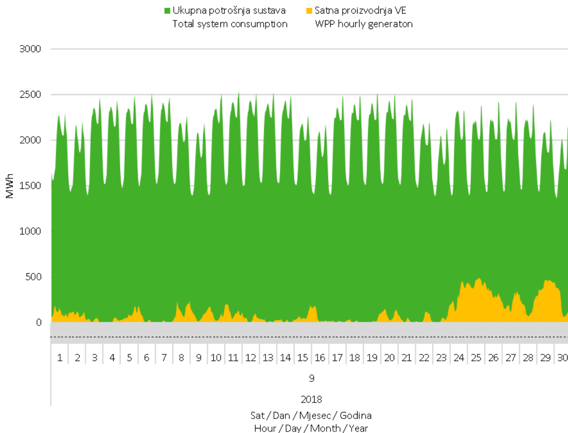
Slika 7 Usporedba satnog dijagrama opterećenja sustava i proizvodnje vjetroelektrana u rujnu 2018. godine
