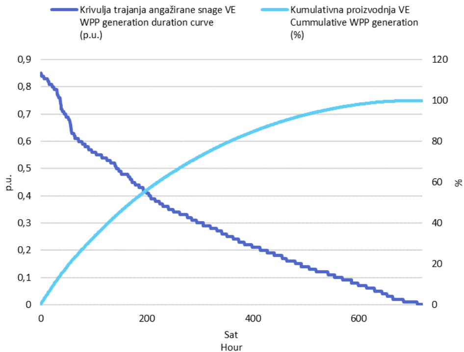
Slika 3 Krivulja trajanja angažirane snage svih VE i kumulativna proizvodnja VE u travnju 2019. godine u jediničnim vrijednostima
