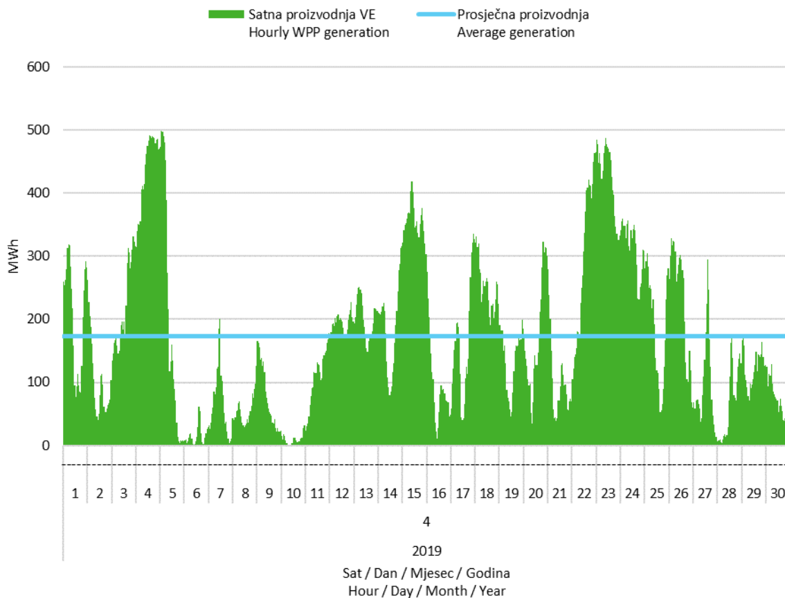
Slika 2 Satna proizvodnja svih vjetroelektrana u travnju 2019. godine
