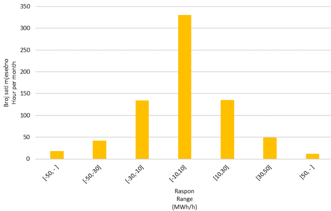
Slika 10 Statistička raspodjela satnih promjena proizvodnje VE u travnju 2019. godine
