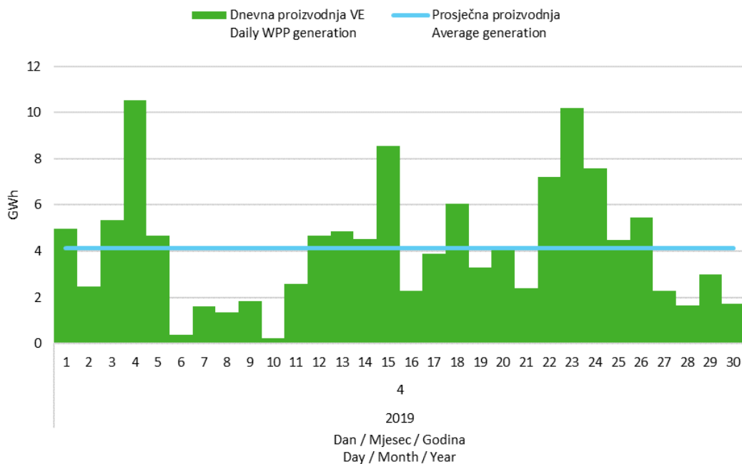
Slika 5 Dnevna proizvodnja svih vjetroelektrana u travnju 2019. godine Figure 5 Daily generation of all wind power plants in April 2019
