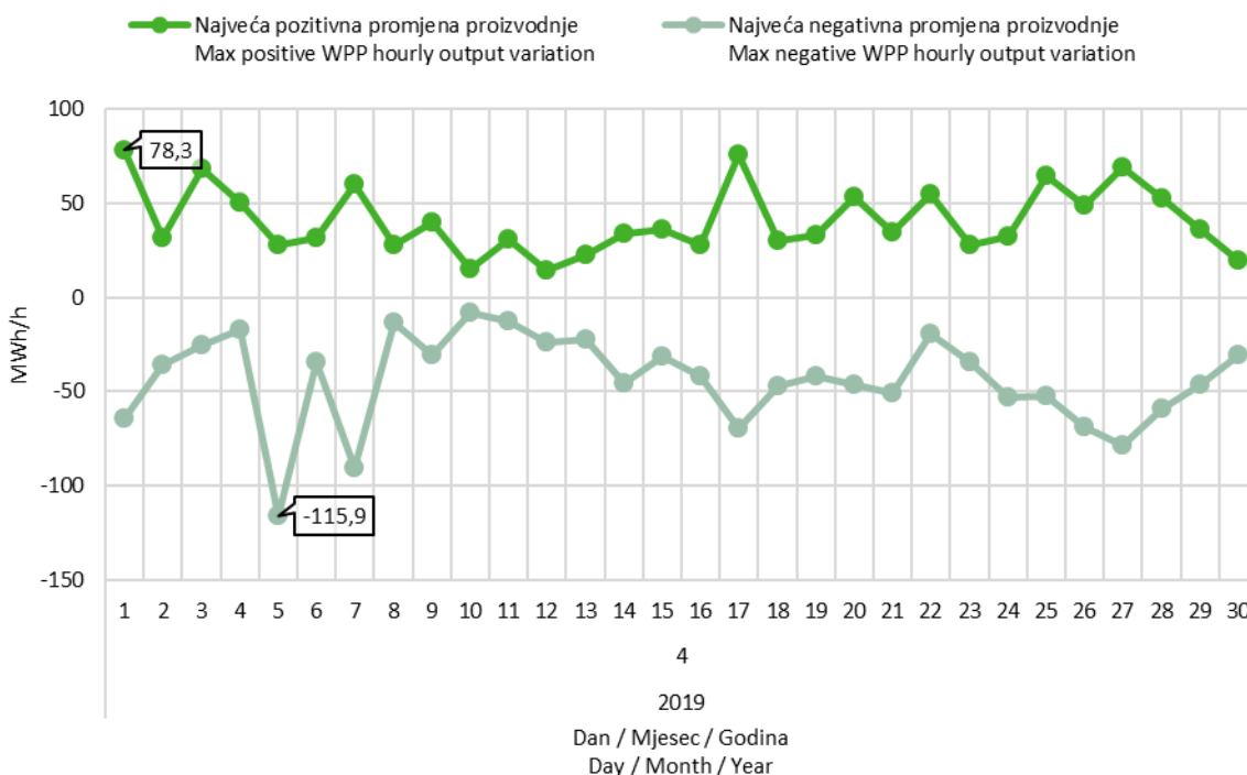
Slika 9 Maksimalna pozitivna i maksimalna negativna promjena satne proizvodnje VE u travnju 2019. godine
