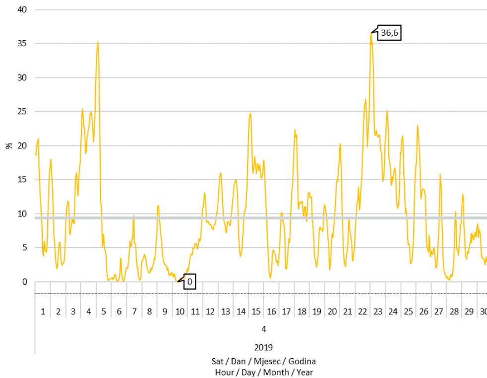
Slika 8 Udio proizvodnje vjetroelektrana u pokrivanju satnog opterećenja elektroenergetskog sustava u travnju 2019. godine
