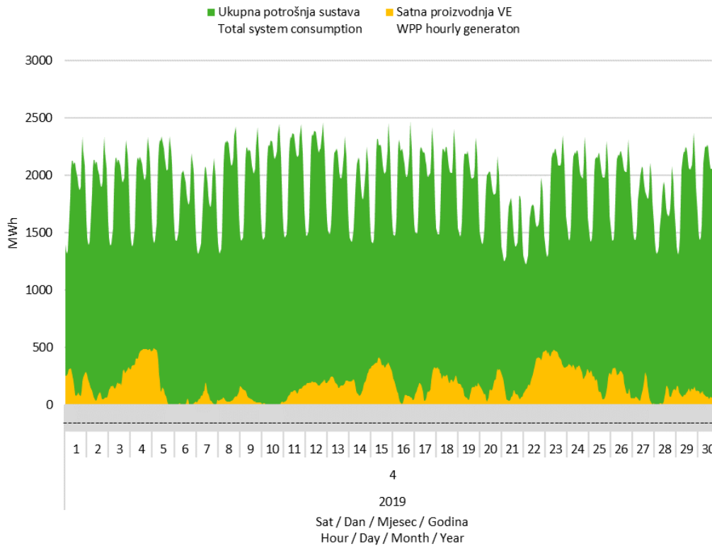
Slika 7 Usporedba satnog dijagrama opterećenja sustava i proizvodnje vjetroelektrana u travnju 2019. godine
