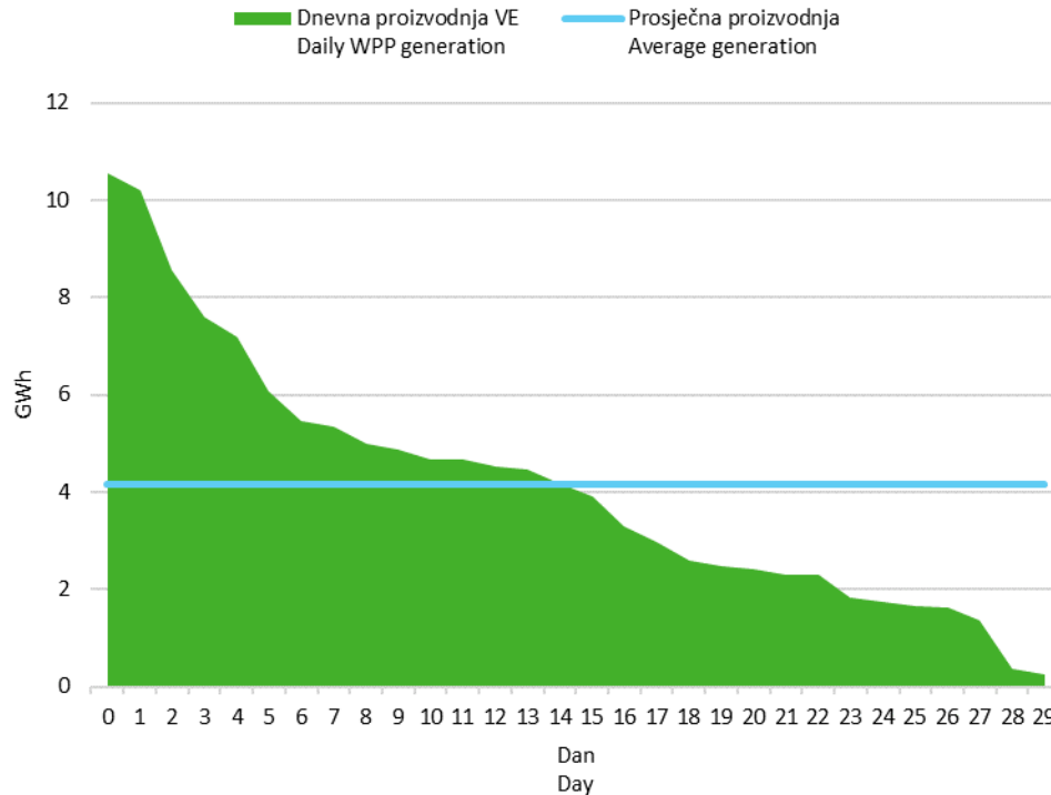
Slika 6 Krivulja trajanja dnevne proizvodnje vjetroelektrana u travnju 2019. godine
