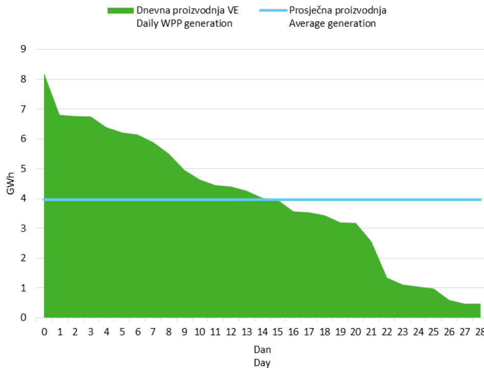
Slika 6 Krivulja trajanja dnevne proizvodnje vjetroelektrana u veljači 2016. godine
