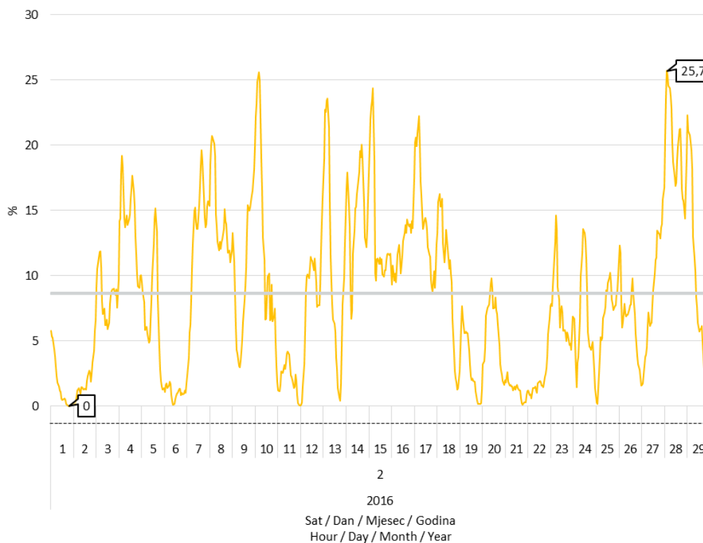
Slika 8 Udio proizvodnje vjetroelektrana u pokrivanju satnog opterećenja elektroenergetskog sustava u veljači 2016. godine
