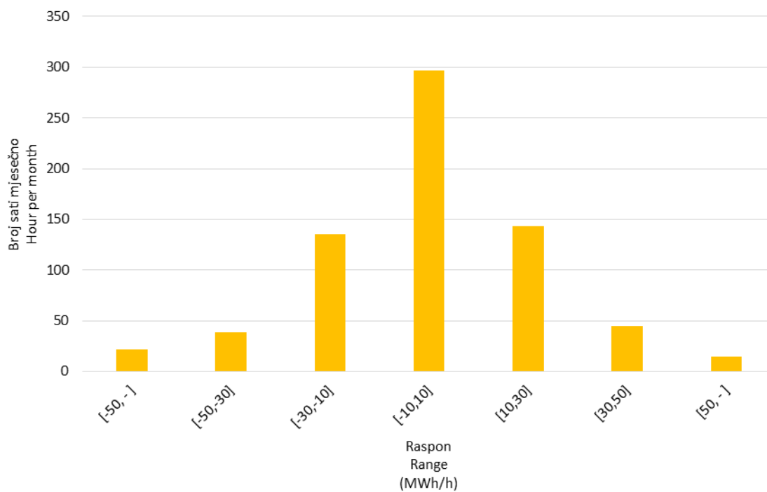
Slika 10 Statistička raspodjela satnih promjena proizvodnje VE u veljači 2016. godine
