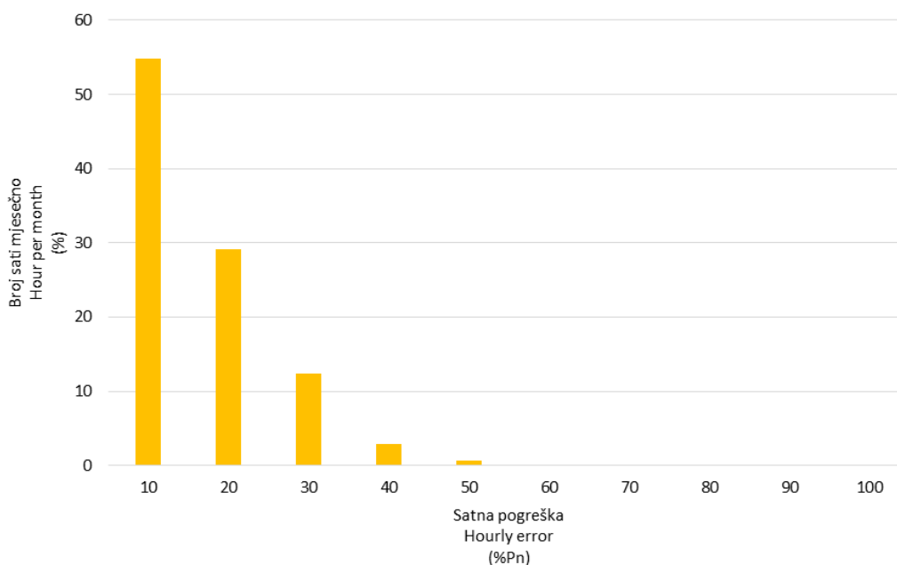
Slika 17 Frekvencija pojavljivanja pogreške prognoze satne proizvodnje svih VE u veljači 2016. godine
