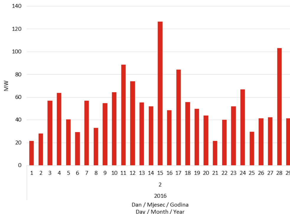
Slika 15 Korijen srednje kvadratne pogreške prognoze satne proizvodnje svih VE u veljači 2016. godine
