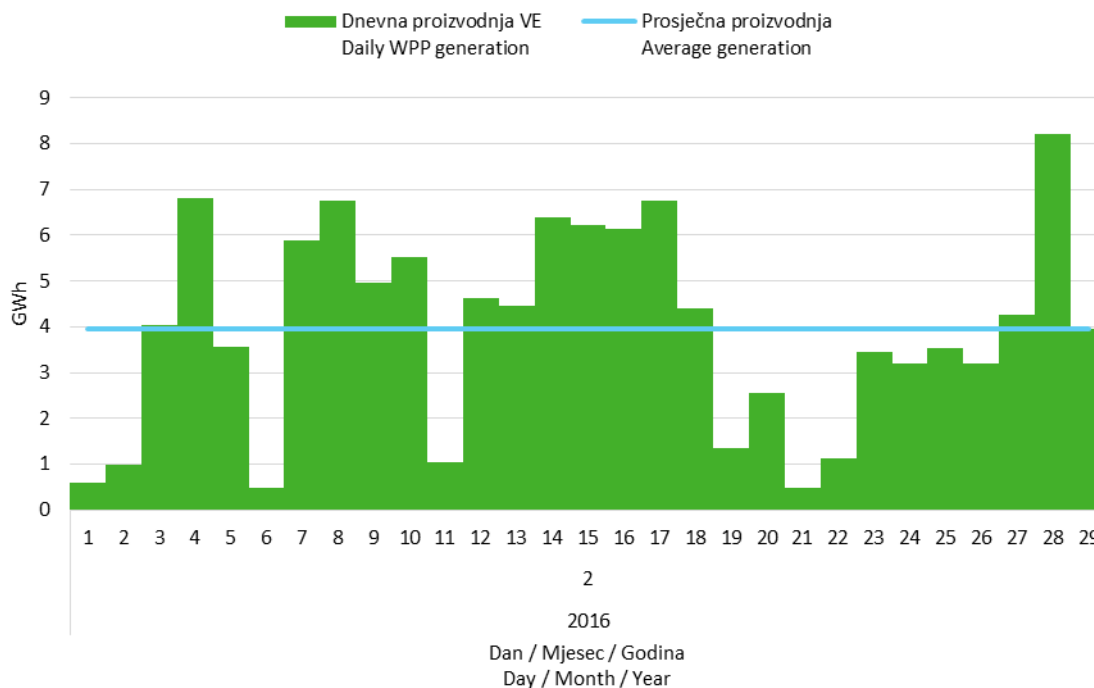
Slika 5 Dnevna proizvodnja svih vjetroelektrana u veljači 2016. godine
