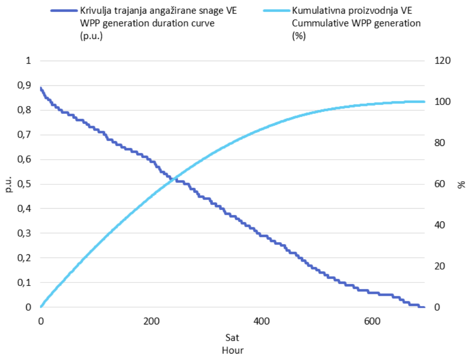
Slika 3 Krivulja trajanja angažirane snage svih VE i kumulativna proizvodnja VE u veljači 2016. godine u jediničnim vrijednostima
