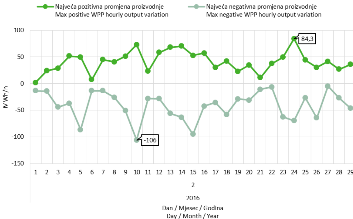
Slika 9 Maksimalna pozitivna i maksimalna negativna promjena satne proizvodnje VE u veljači 2016. godine
