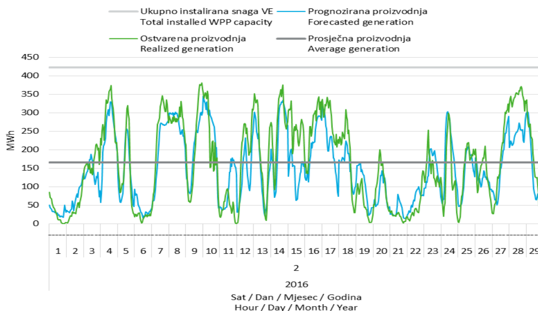
Slika 11 Prognozirana i ostvarena satna proizvodnja vjetroelektrana u veljači 2016. godine
