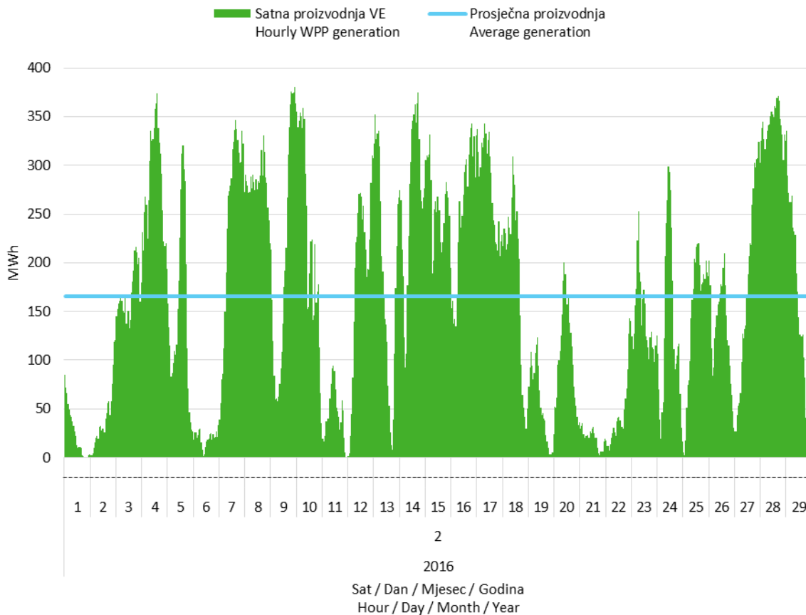
Slika 2 Satna proizvodnja svih vjetroelektrana u veljači 2016. godine Figure 2 Hourly generation of all wind power plants in February 2016
