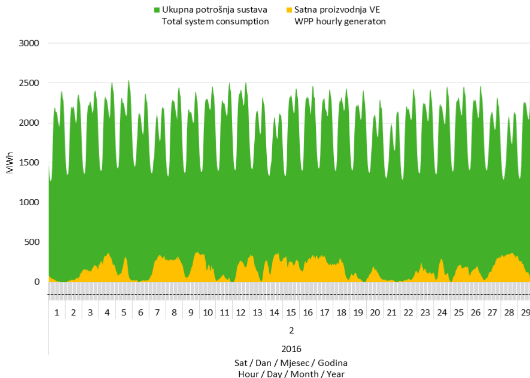
Slika 7 Usporedba satnog dijagrama opterećenja sustava i proizvodnje vjetroelektrana u veljači 2016. godine
