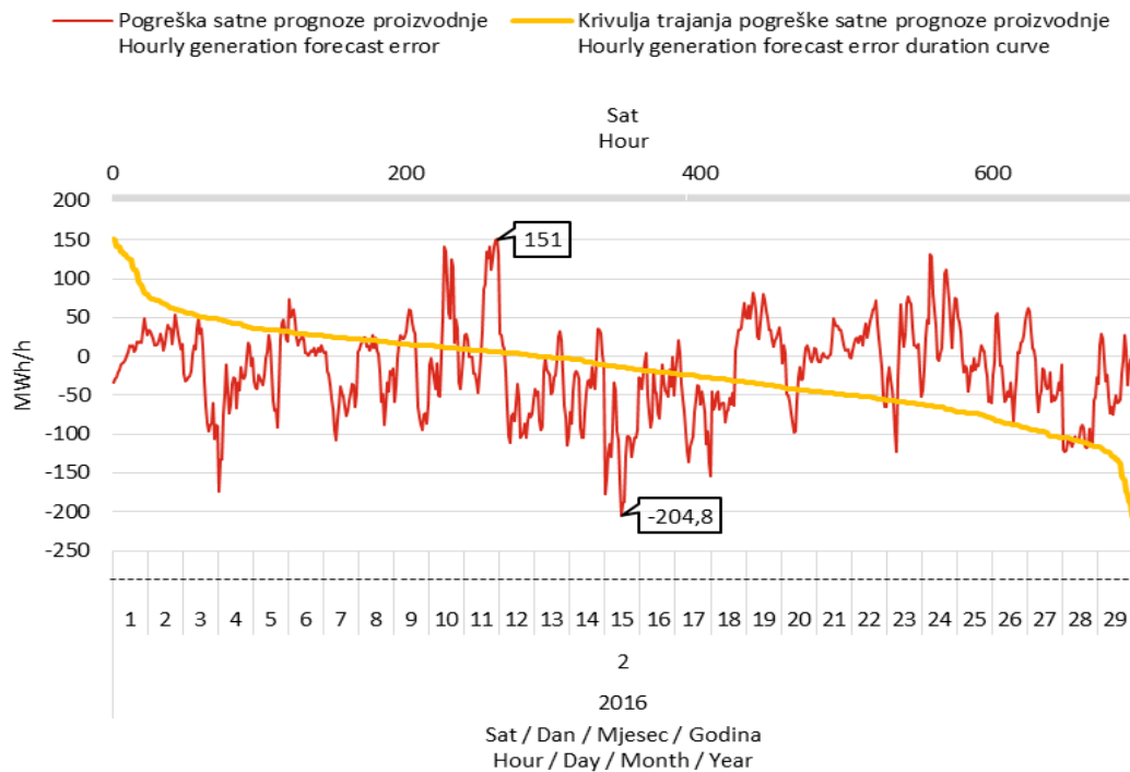
Slika 12 Razlika između prognozirane i ostvarene satne proizvodnje svih VE (pogreška prognoze) i pripadna krivulja trajanja u veljači 2016. godine
