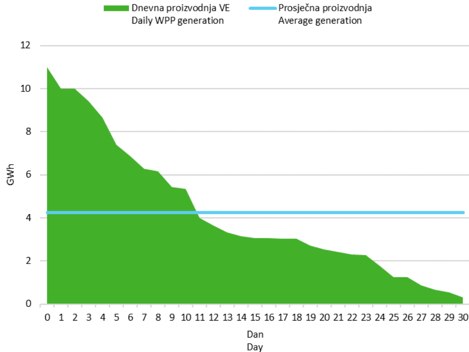
Slika 6 Krivulja trajanja dnevne proizvodnje vjetroelektrana u listopadu 2018. godine
