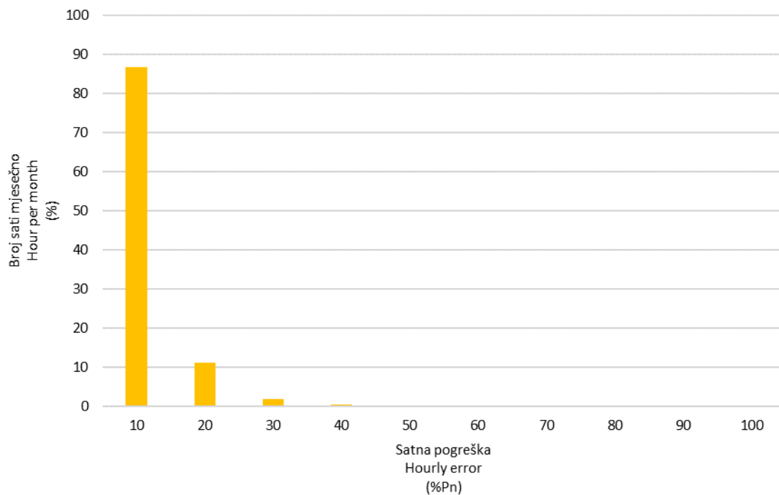
Slika 17 Frekvencija pojavljivanja pogreške prognoze satne proizvodnje svih VE u listopadu 2018. godine
