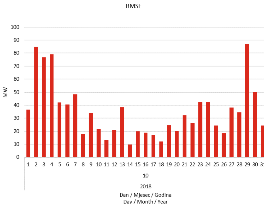
Slika 15 Korijen srednje kvadratne pogreške prognoze satne proizvodnje svih VE u listopadu 2018. godine
