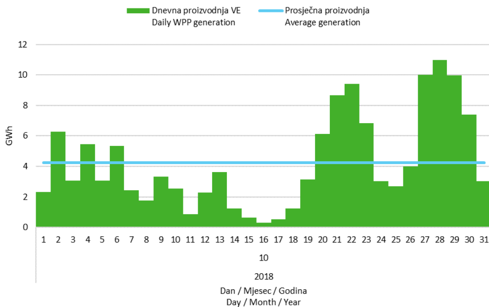
Slika 5 Dnevna proizvodnja svih vjetroelektrana u listopadu 2018. godine
