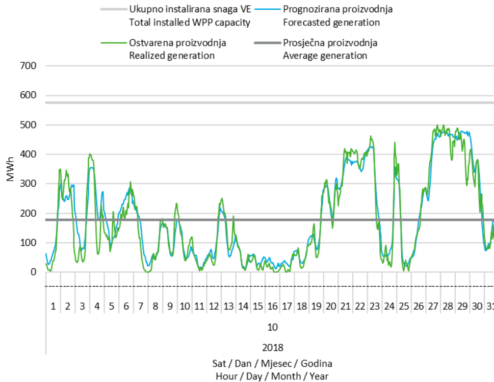
Slika 11 Prognozirana i ostvarena satna proizvodnja vjetroelektrana u listopadu 2018. godine
