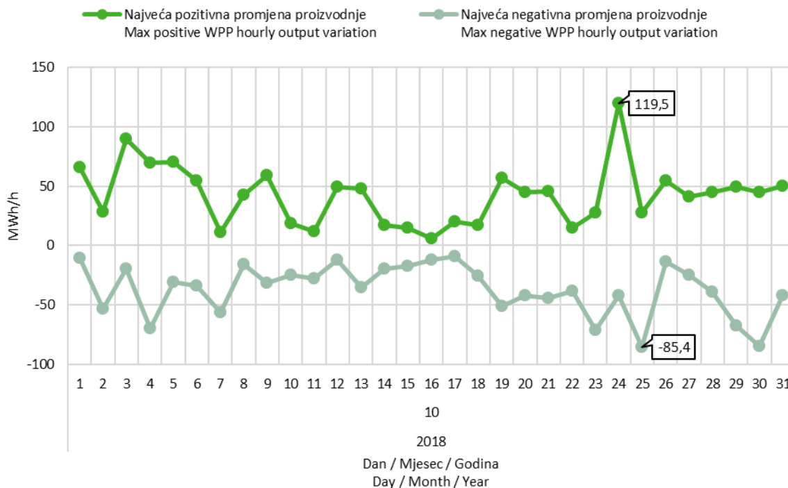
Slika 9 Maksimalna pozitivna i maksimalna negativna promjena satne proizvodnje VE u listopadu 2018. godine
