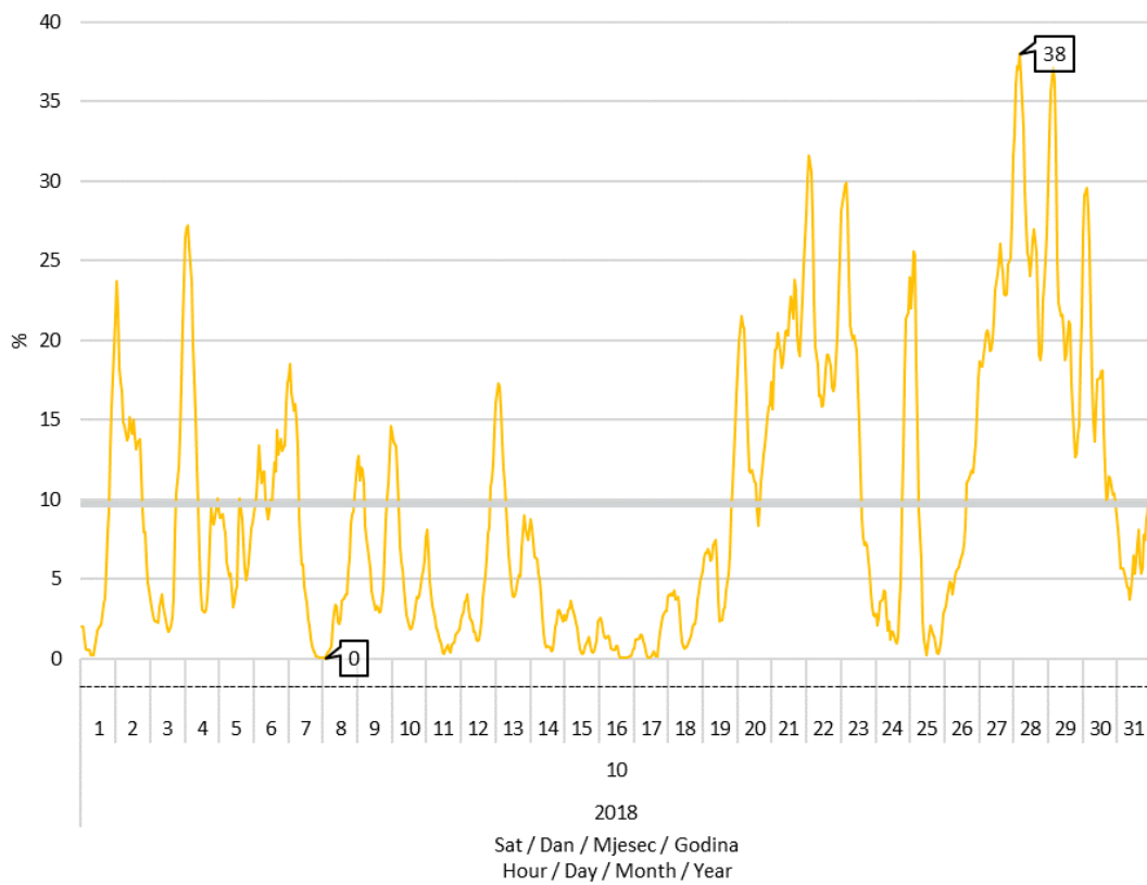
Slika 8 Udio proizvodnje vjetroelektrana u pokrivanju satnog opterećenja elektroenergetskog sustava u listopadu 2018. godine
