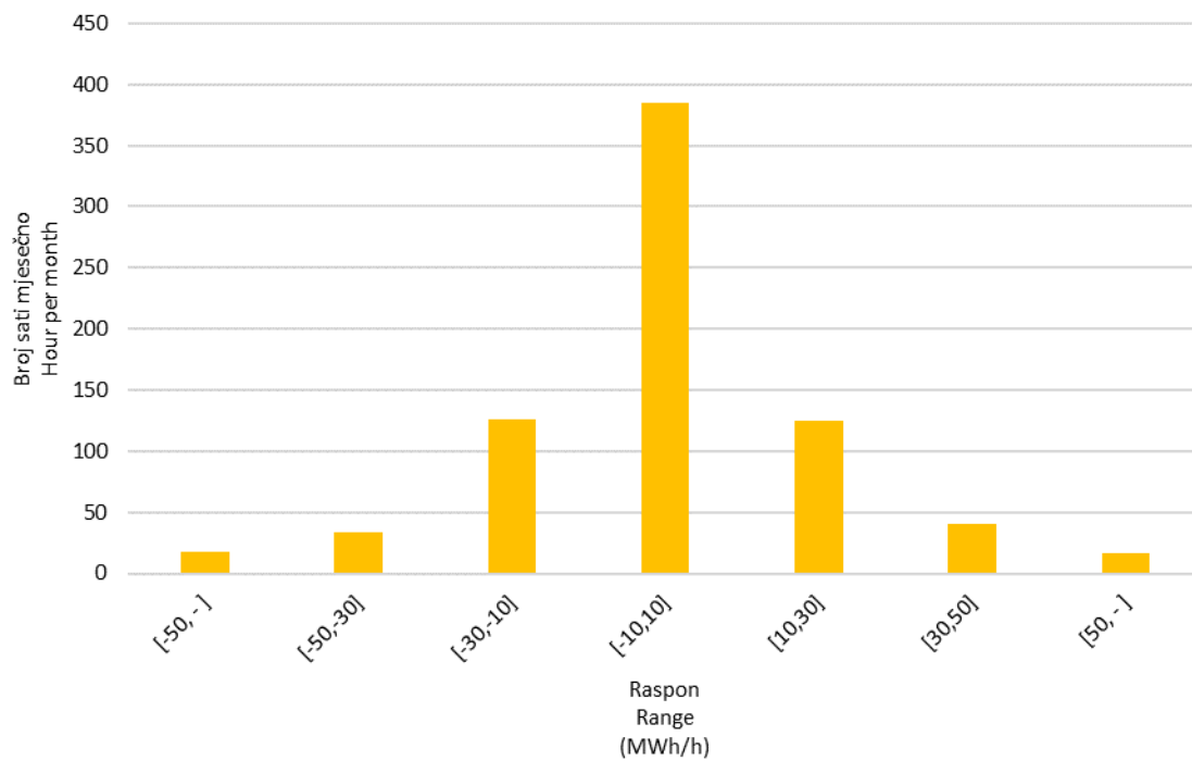
Slika 10 Statistička raspodjela satnih promjena proizvodnje VE u listopadu 2018. godine
