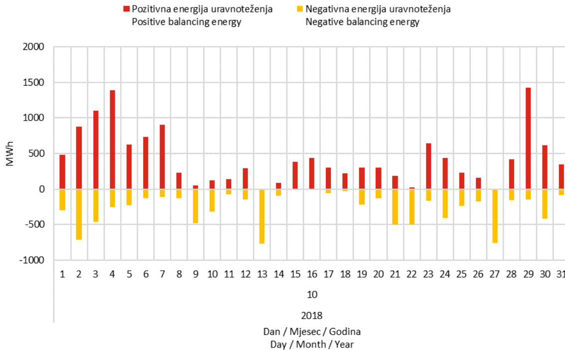
Slika 14 Suma pozitivnih pogreški prognoze satne proizvodnje VE (negativna energija uravnoteženja) i suma negativnih pogreški prognoze satne proizvodnje VE (pozitivna energija uravnoteženja) u listopadu 2018. godine
