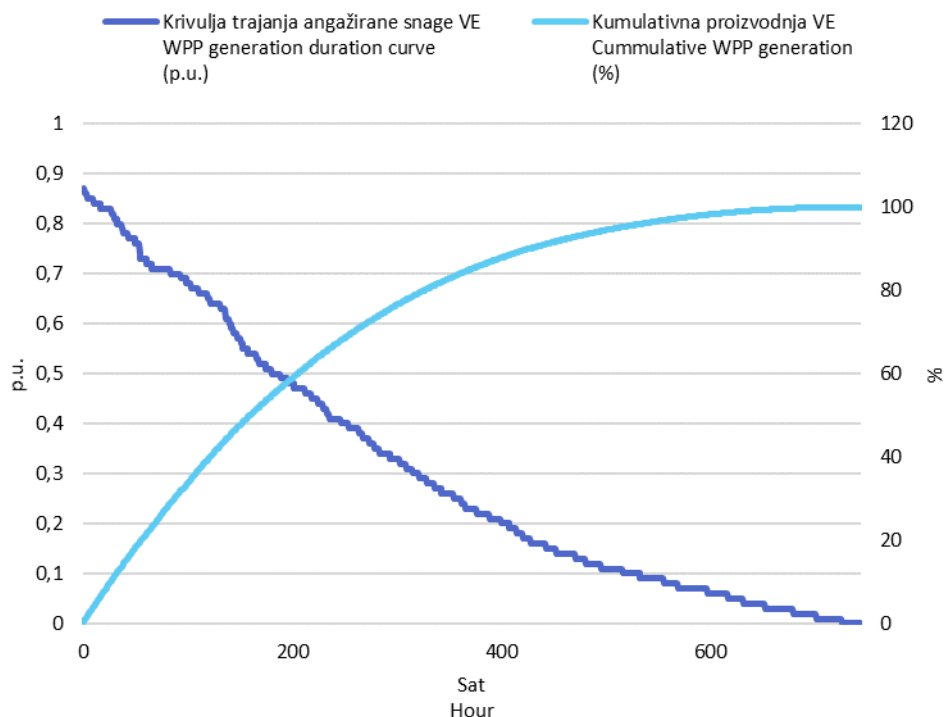
Slika 3 Krivulja trajanja angažirane snage svih VE i kumulativna proizvodnja VE u listopadu 2018. godine u jediničnim vrijednostima
