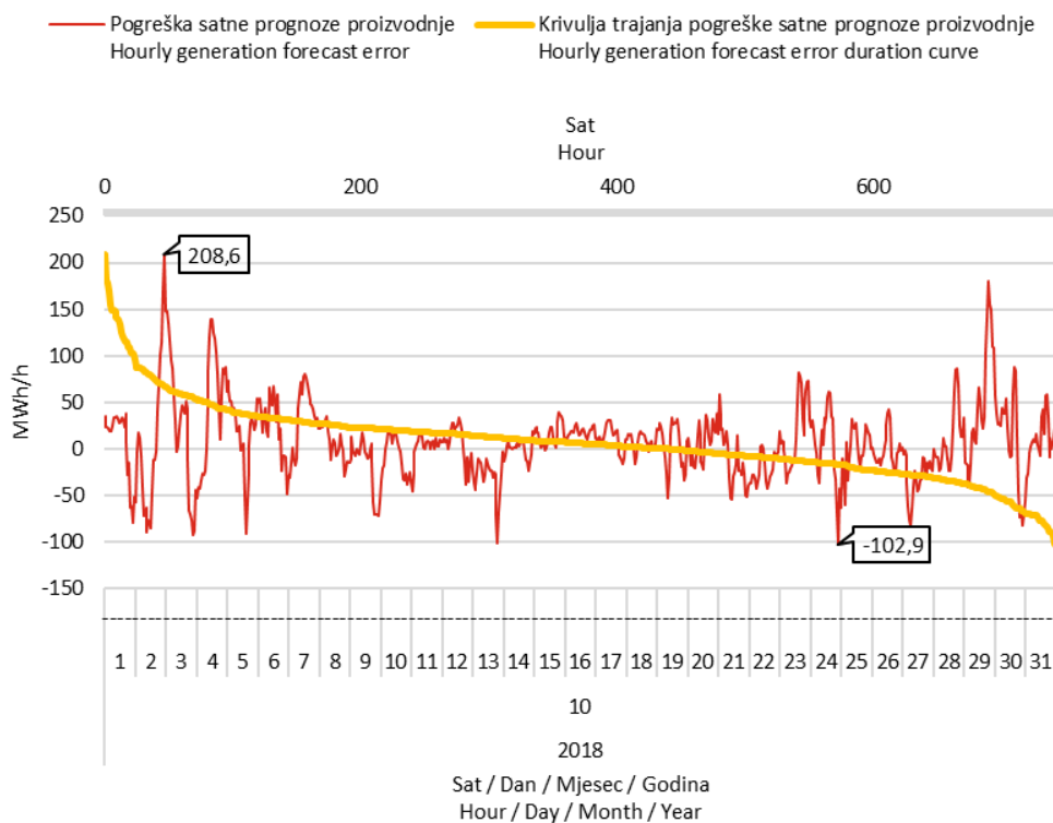
Slika 12 Razlika između prognozirane i ostvarene satne proizvodnje svih VE (pogreška prognoze) i pripadna krivulja trajanja u listopadu 2018. godine
