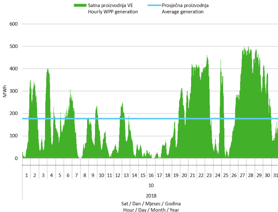
Slika 2 Satna proizvodnja svih vjetroelektrana u listopadu 2018. godine
