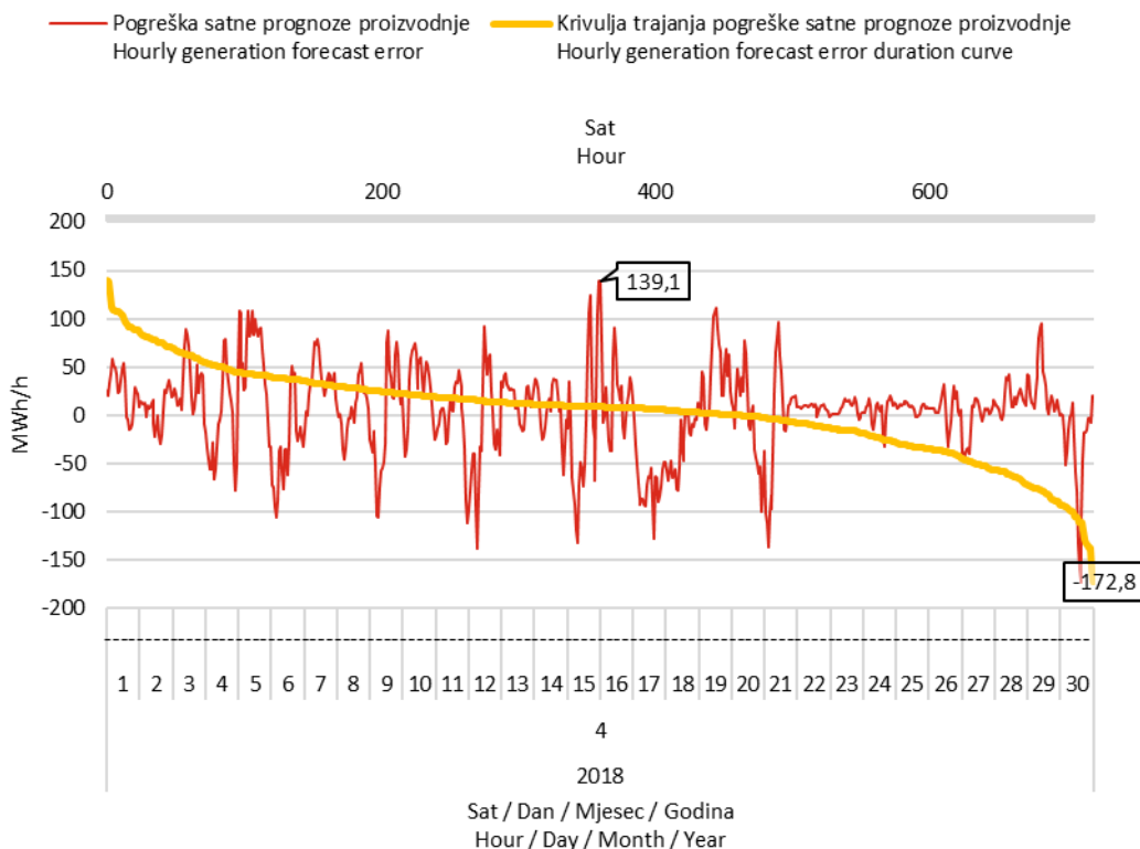
Slika 12 Razlika između prognozirane i ostvarene satne proizvodnje svih VE (pogreška prognoze) i pripadna krivulja trajanja u travnju 2018. godine
