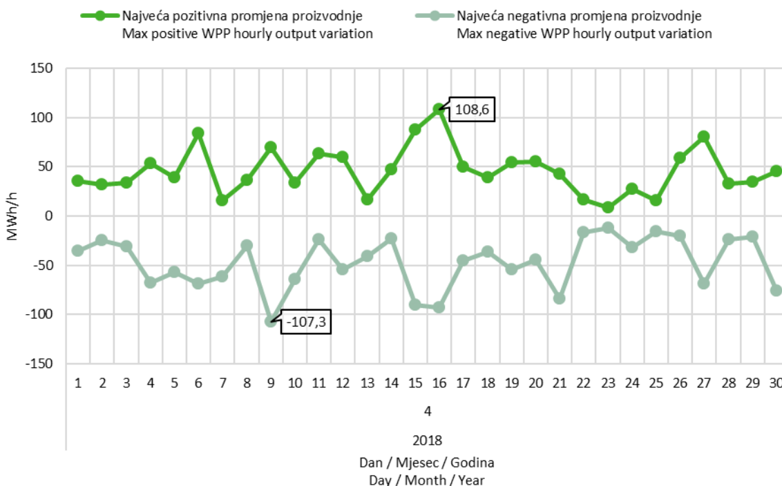
Slika 9 Maksimalna pozitivna i maksimalna negativna promjena satne proizvodnje VE u travnju 2018. godine
