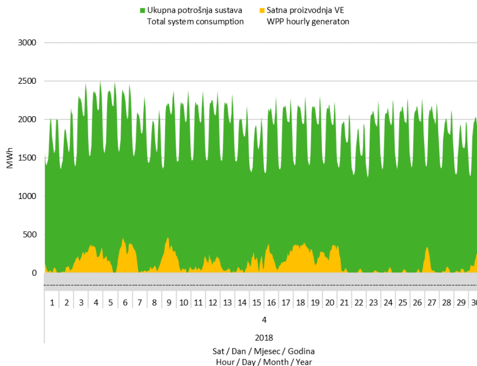
Slika 7 Usporedba satnog dijagrama opterećenja sustava i proizvodnje vjetroelektrana u travnju 2018. godine
