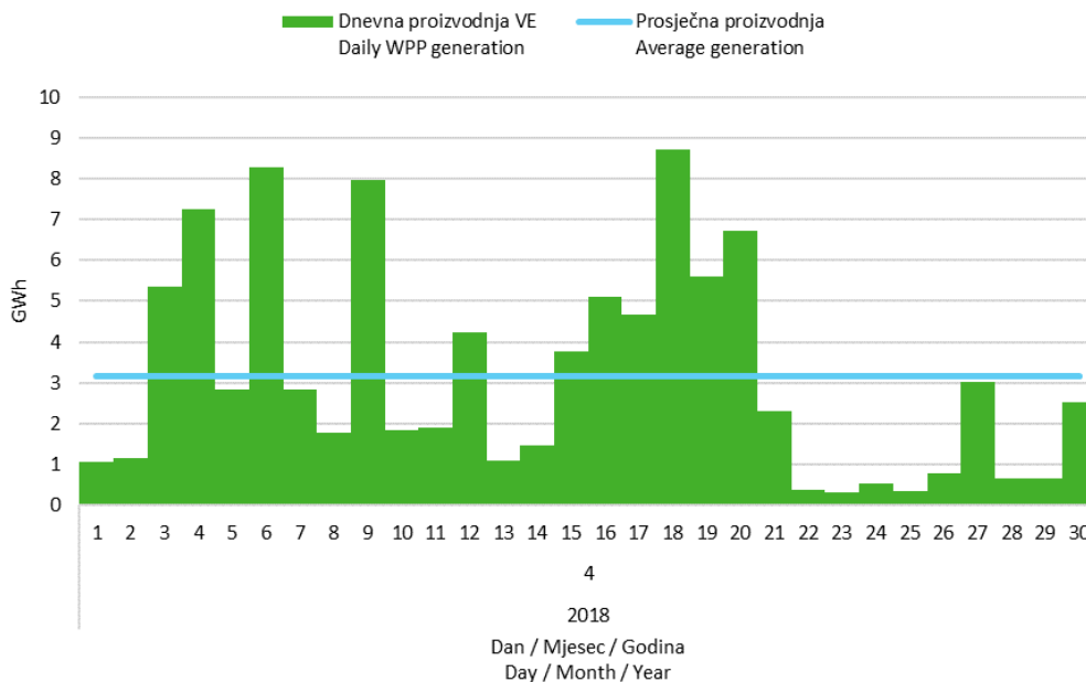
Slika 5 Dnevna proizvodnja svih vjetroelektrana u travnju 2018. godine
