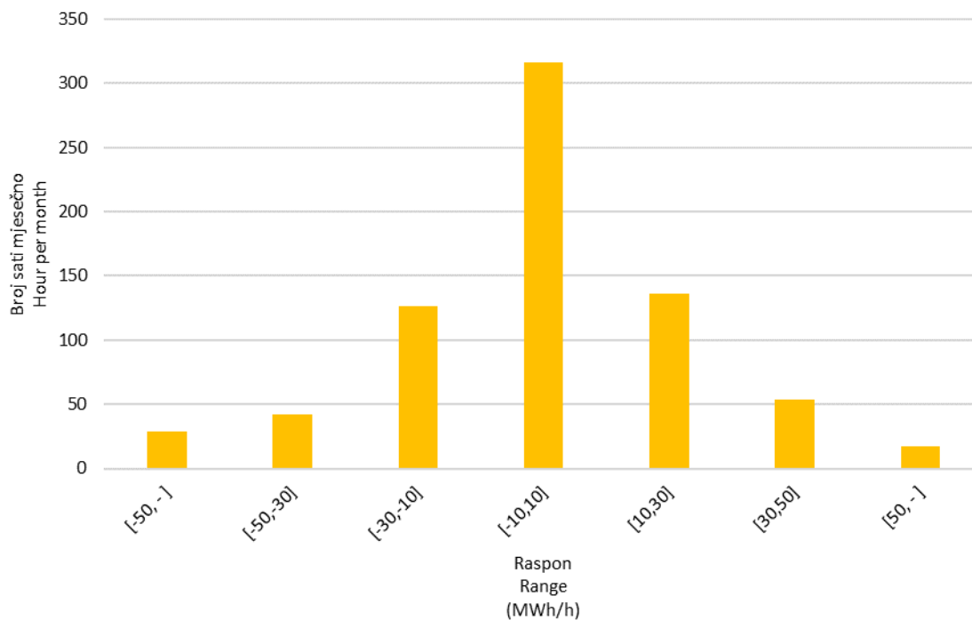
Slika 10 Statistička raspodjela satnih promjena proizvodnje VE u travnju 2018. godine
