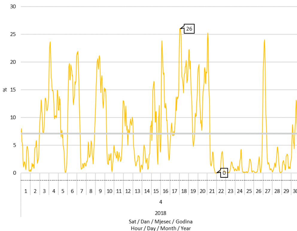
Slika 8 Udio proizvodnje vjetroelektrana u pokrivanju satnog opterećenja elektroenergetskog sustava u travnju 2018. godine
