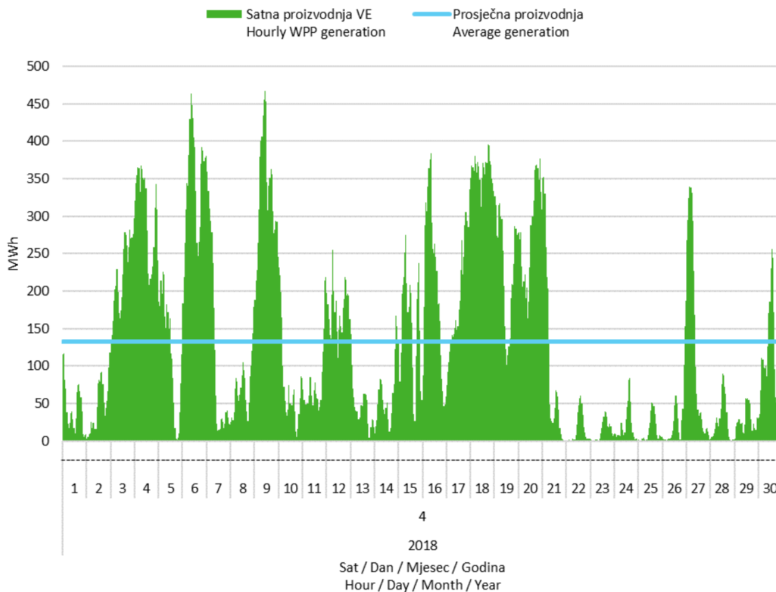
Slika 2 Satna proizvodnja svih vjetroelektrana u travnju 2018. godine
