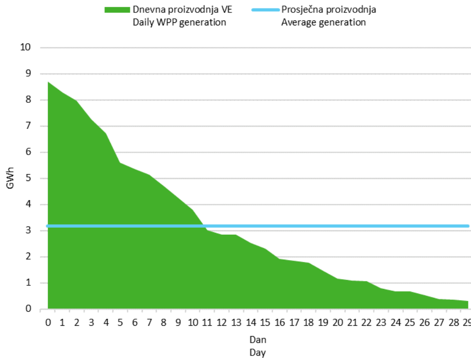
Slika 6 Krivulja trajanja dnevne proizvodnje vjetroelektrana u travnju 2018. godine
