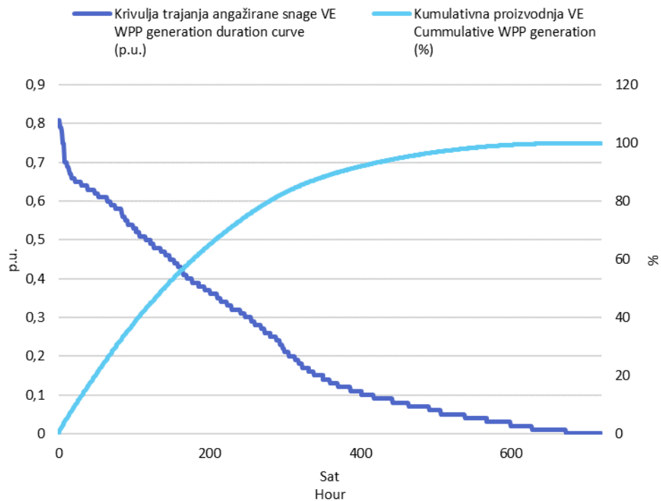
Slika 3 Krivulja trajanja angažirane snage svih VE i kumulativna proizvodnja VE u travnju 2018. godine u jediničnim vrijednostima
