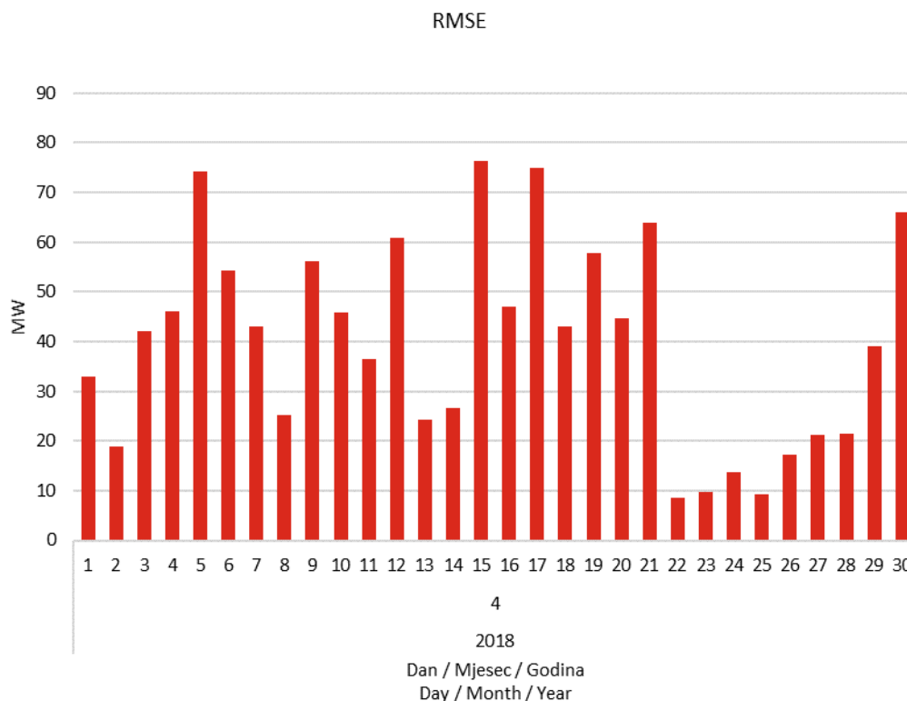
Slika 15 Korijen srednje kvadratne pogreške prognoze satne proizvodnje svih VE u travnju 2018. godine
