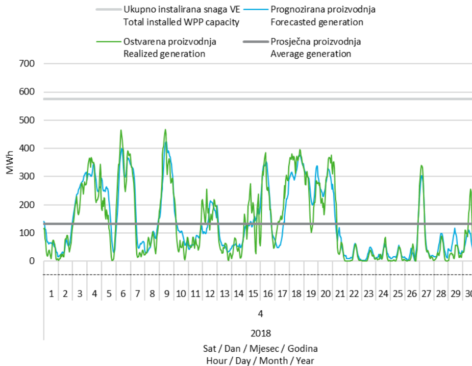
Slika 11 Prognozirana i ostvarena satna proizvodnja vjetroelektrana u travnju 2018. godine
