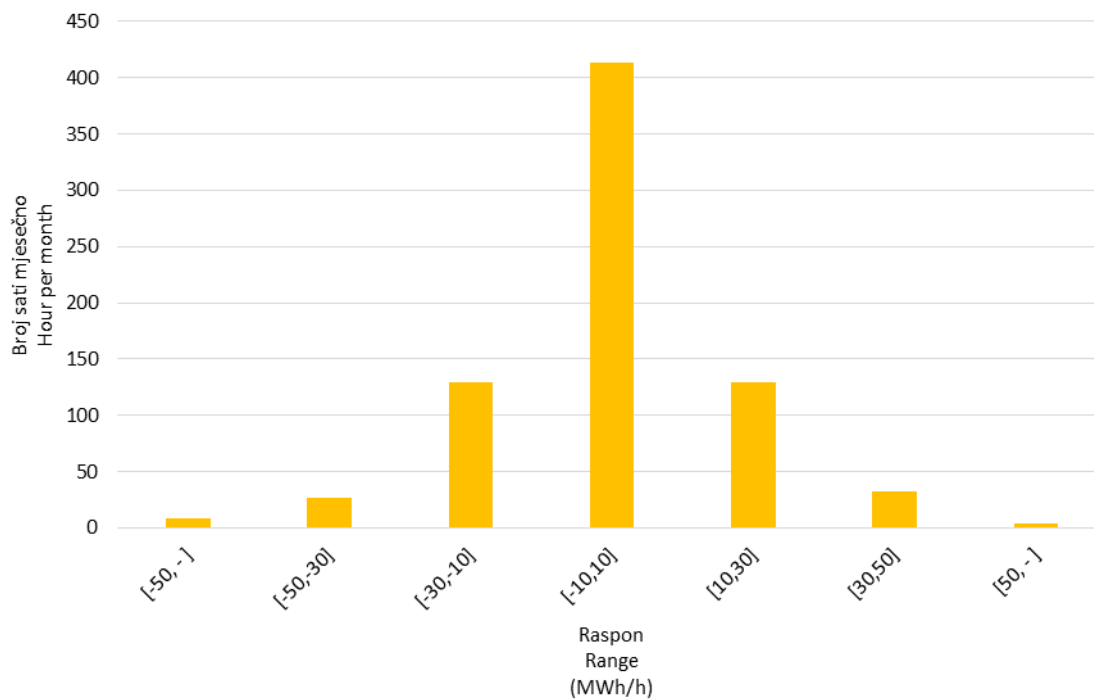
Slika 10 Statistička raspodjela satnih promjena proizvodnje VE u srpnju 2017. godine
