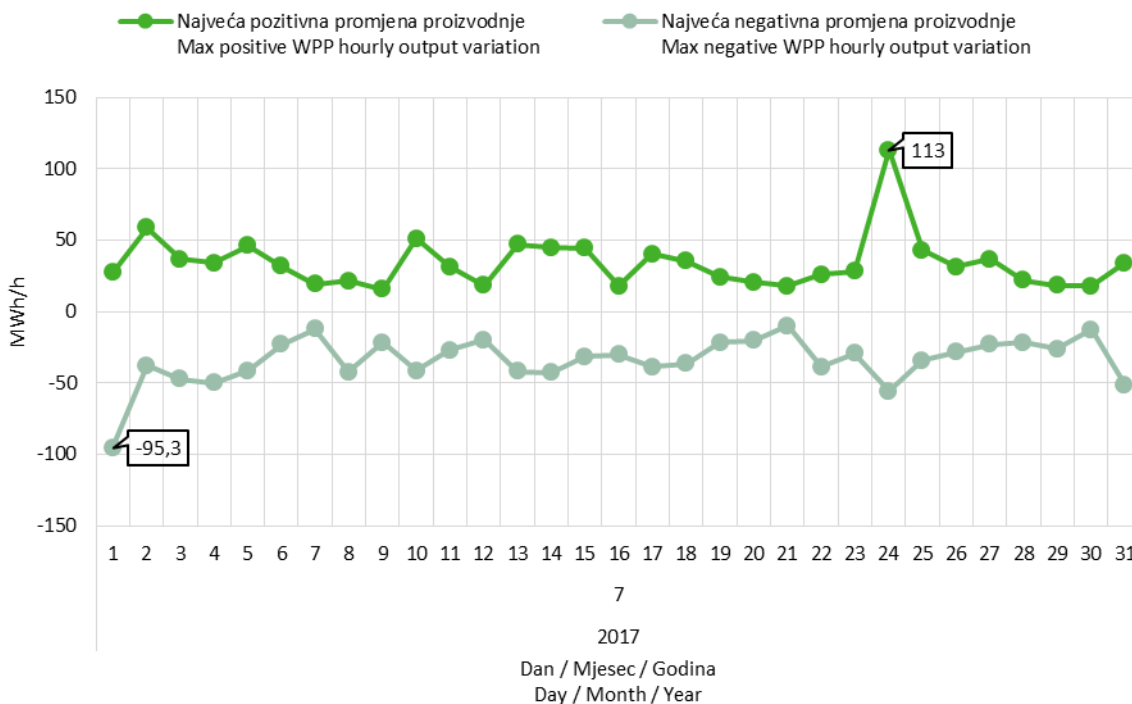
Slika 9 Maksimalna pozitivna i maksimalna negativna promjena satne proizvodnje VE u srpnju 2017. godine
