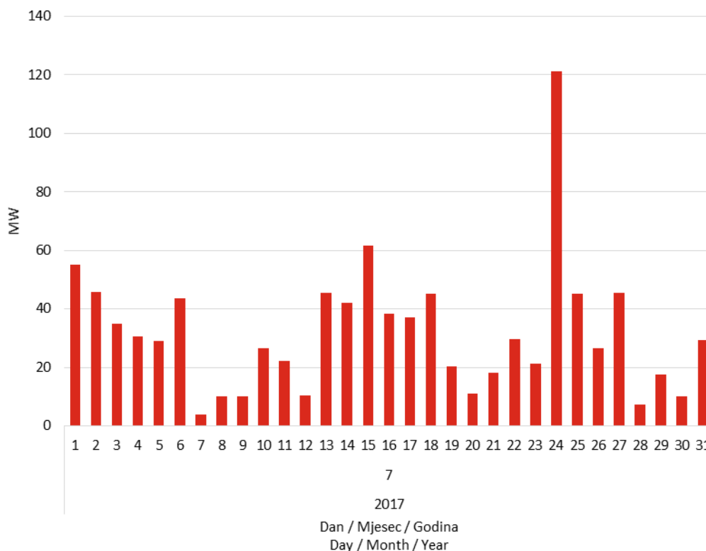
Slika 15 Korijen srednje kvadratne pogreške prognoze satne proizvodnje svih VE u srpnju 2017. godine
