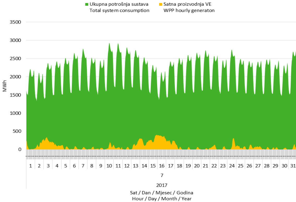
Slika 7 Usporedba satnog dijagrama opterećenja sustava i proizvodnje vjetroelektrana u srpnju 2017. godine
