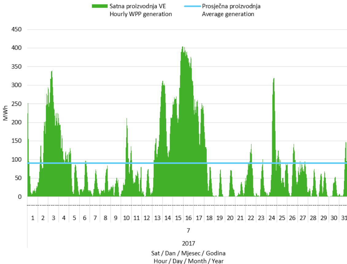
Slika 2 Satna proizvodnja svih vjetroelektrana u srpnju 2017. godine
