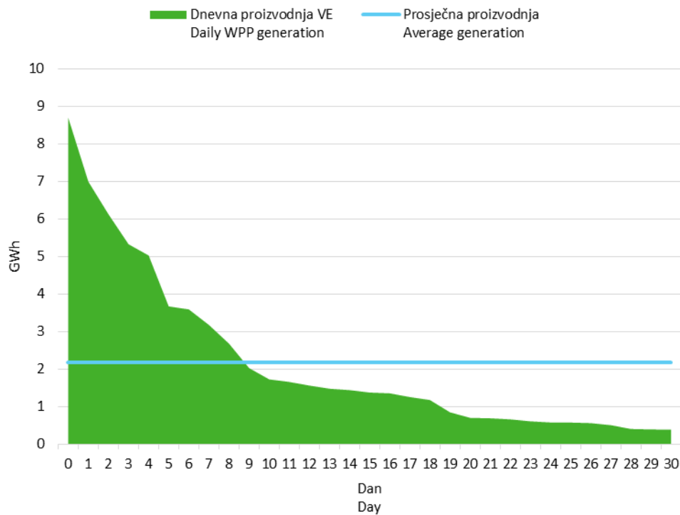
Slika 6 Krivulja trajanja dnevne proizvodnje vjetroelektrana u srpnju 2017. godine
