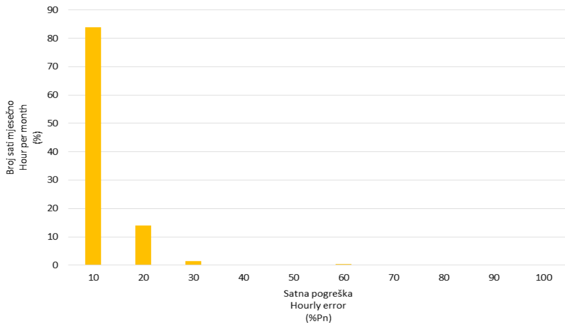
Slika 17 Frekvencija pojavljivanja pogreške prognoze satne proizvodnje svih VE u srpnju 2017. godine
