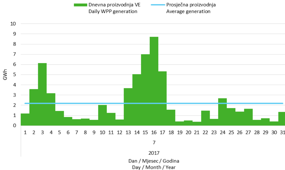
Slika 5 Dnevna proizvodnja svih vjetroelektrana u srpnju 2017. godine
