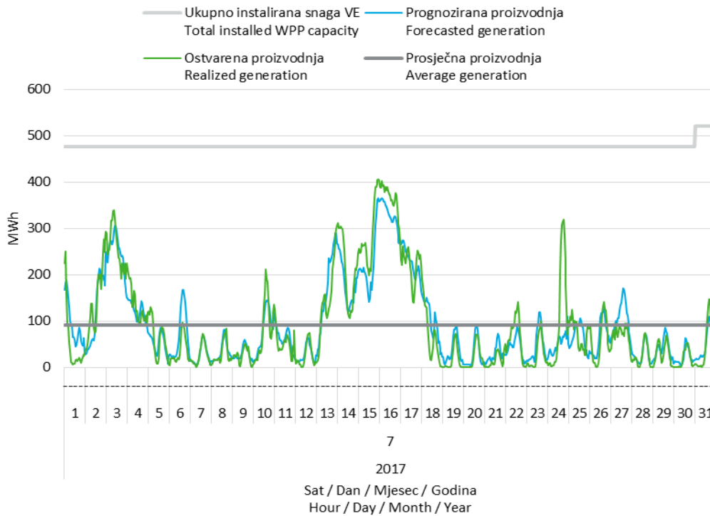
Slika 11 Prognozirana i ostvarena satna proizvodnja vjetroelektrana u srpnju 2017. godine
