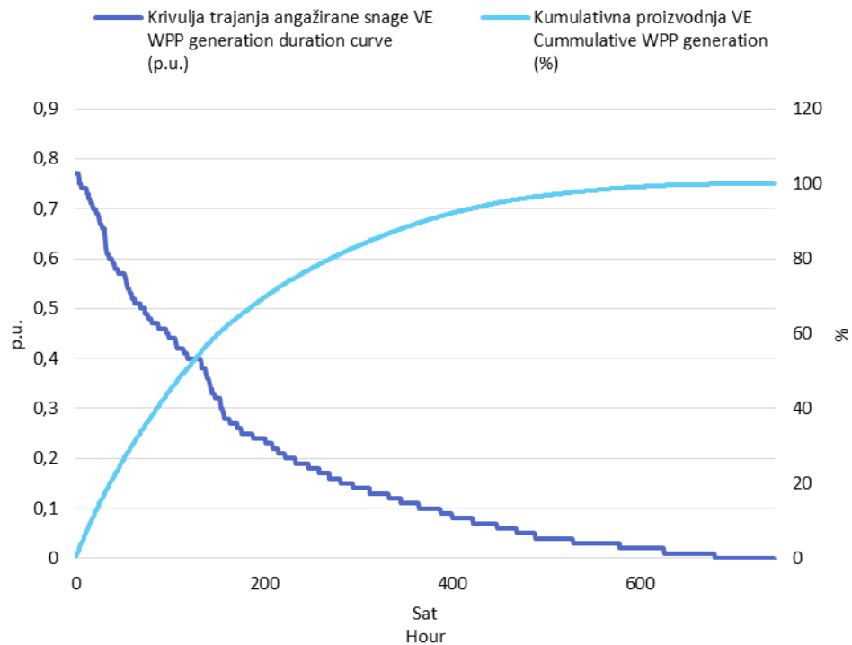
Slika 3 Krivulja trajanja angažirane snage svih VE i kumulativna proizvodnja VE u srpnju 2017. godine u jediničnim vrijednostima
