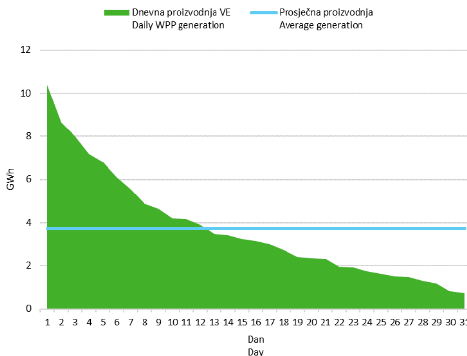
Slika 6 Krivulja trajanja dnevne proizvodnje vjetroelektrana u srpnju 2023. godine
