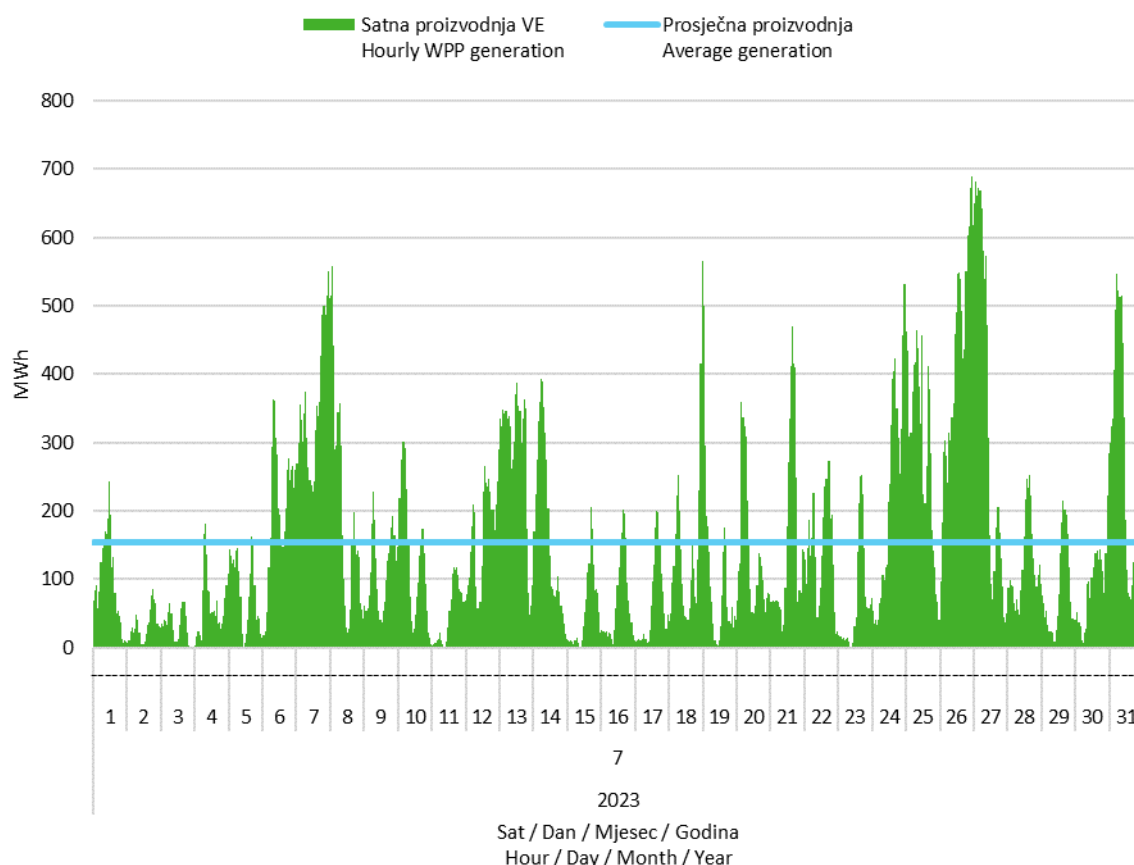
Slika 2 Satna proizvodnja svih vjetroelektrana u srpnju 2023. godine
