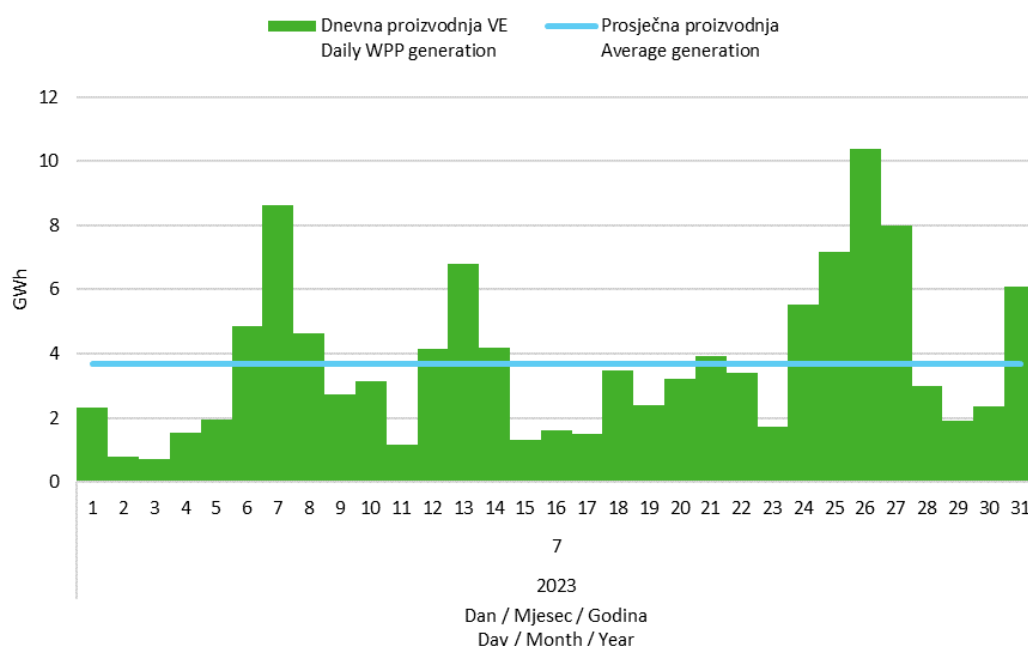
Slika 5 Dnevna proizvodnja svih vjetroelektrana u srpnju 2023. godine
