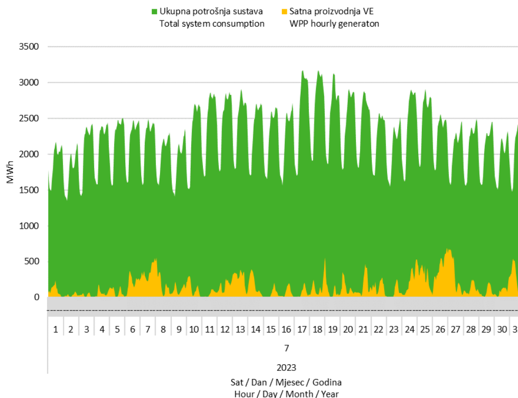
Slika 7 Usporedba satnog dijagrama opterećenja sustava i proizvodnje vjetroelektrana u srpnju 2023. godine
