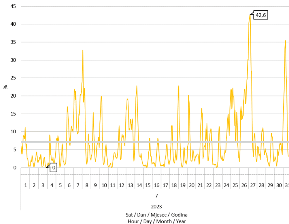
Slika 8 Udio proizvodnje vjetroelektrana u pokrivanju satnog opterećenja elektroenergetskog sustava u srpnju 2023. godine
