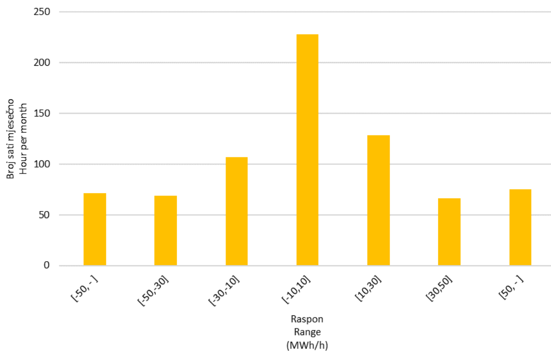
Slika 10 Statistička raspodjela satnih promjena proizvodnje VE u srpnju 2023. godine
