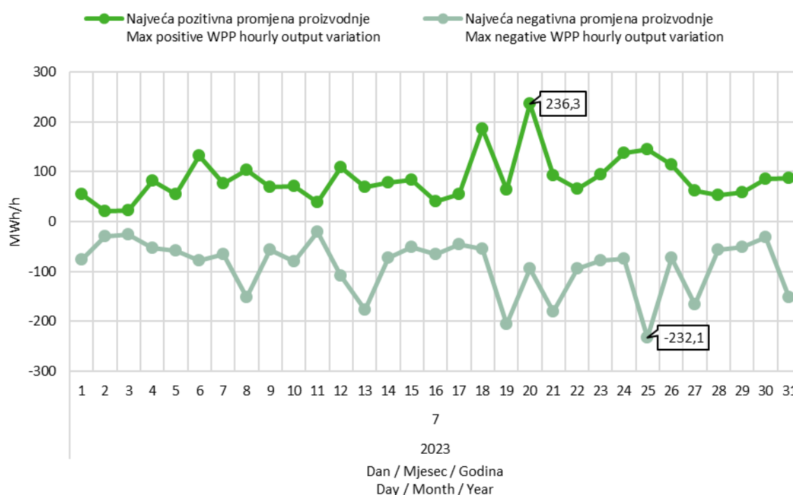
Slika 9 Maksimalna pozitivna i maksimalna negativna promjena satne proizvodnje VE u srpnju 2023. godine
