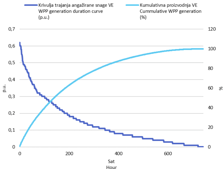
Slika 3 Krivulja trajanja angažirane snage svih VE i kumulativna proizvodnja VE u srpnju 2023. godine u jediničnim vrijednostima
