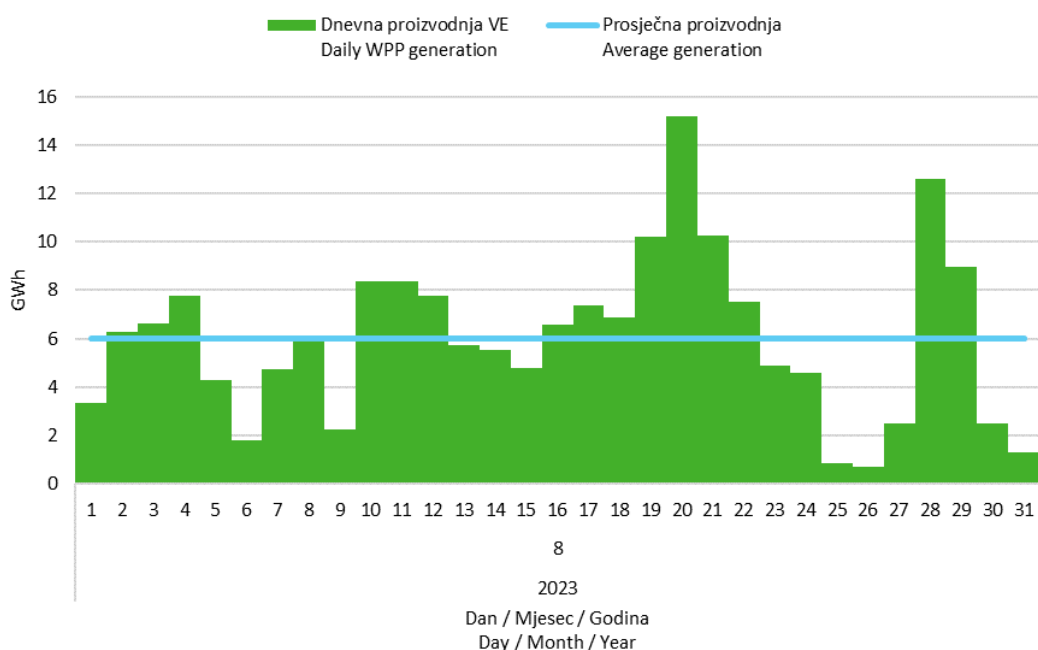
Slika 5 Dnevna proizvodnja svih vjetroelektrana u kolovozu 2023. godine
