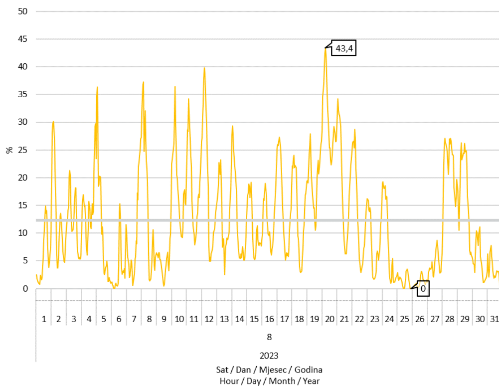
Slika 8 Udio proizvodnje vjetroelektrana u pokrivanju satnog opterećenja elektroenergetskog sustava u kolovozu 2023. godine
