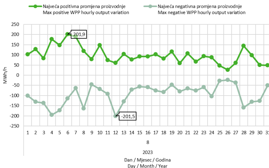
Slika 9 Maksimalna pozitivna i maksimalna negativna promjena satne proizvodnje VE u kolovozu 2023. godine
