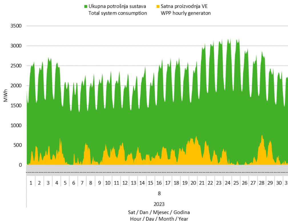
Slika 7 Usporedba satnog dijagrama opterećenja sustava i proizvodnje vjetroelektrana u kolovozu 2023. godine
