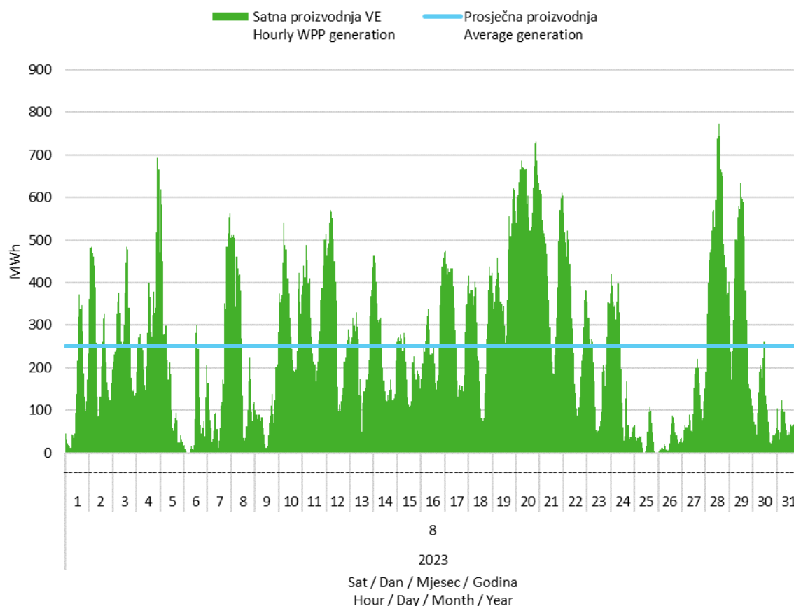
Slika 2 Satna proizvodnja svih vjetroelektrana u kolovozu 2023. godine
