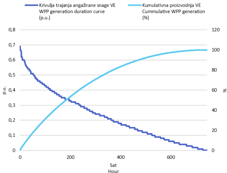
Slika 3 Krivulja trajanja angažirane snage svih VE i kumulativna proizvodnja VE u kolovozu 2023. godine u jediničnim vrijednostima
