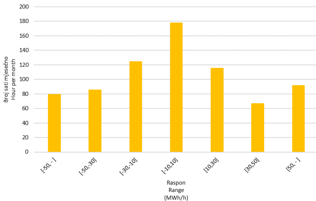
Slika 10 Statistička raspodjela satnih promjena proizvodnje VE u kolovozu 2023. godine
