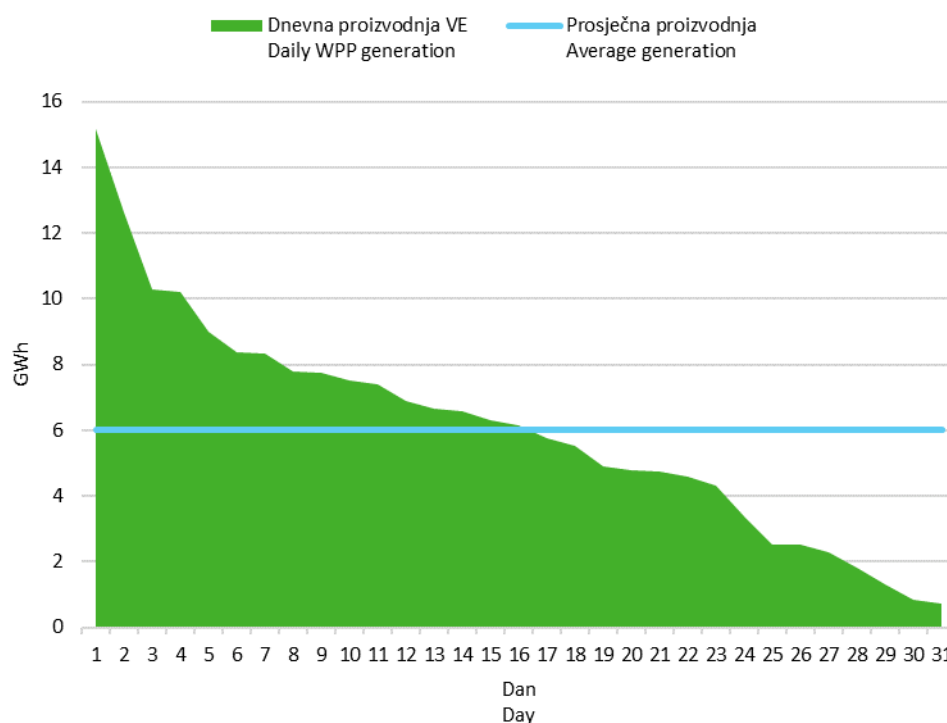
Slika 6 Krivulja trajanja dnevne proizvodnje vjetroelektrana u kolovozu 2023. godine
