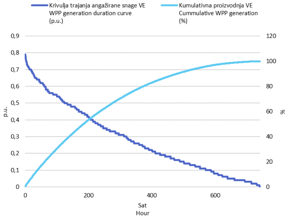
Slika 3 Krivulja trajanja angažirane snage svih VE i kumulativna proizvodnja VE u ožujku 2023. godine u jediničnim vrijednostima
