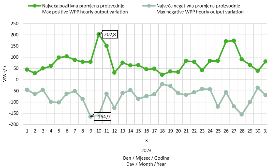
Slika 9 Maksimalna pozitivna i maksimalna negativna promjena satne proizvodnje VE u ožujku 2023. godine
