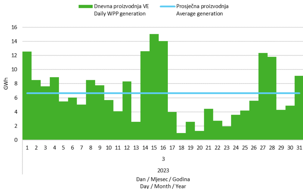
Slika 5 Dnevna proizvodnja svih vjetroelektrana u ožujku 2023. godine Figure 5 Daily generation of all wind power plants in March 2023
