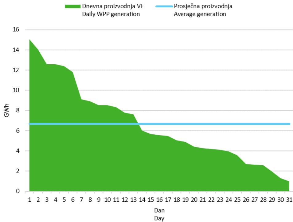
Slika 6 Krivulja trajanja dnevne proizvodnje vjetroelektrana u ožujku 2023. godine
