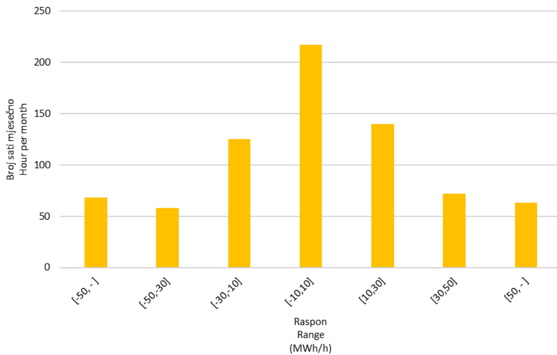
Slika 10 Statistička raspodjela satnih promjena proizvodnje VE u ožujku 2023. godine Figure 10 Statistical distribution of WPP hourly output variations in March 2023
