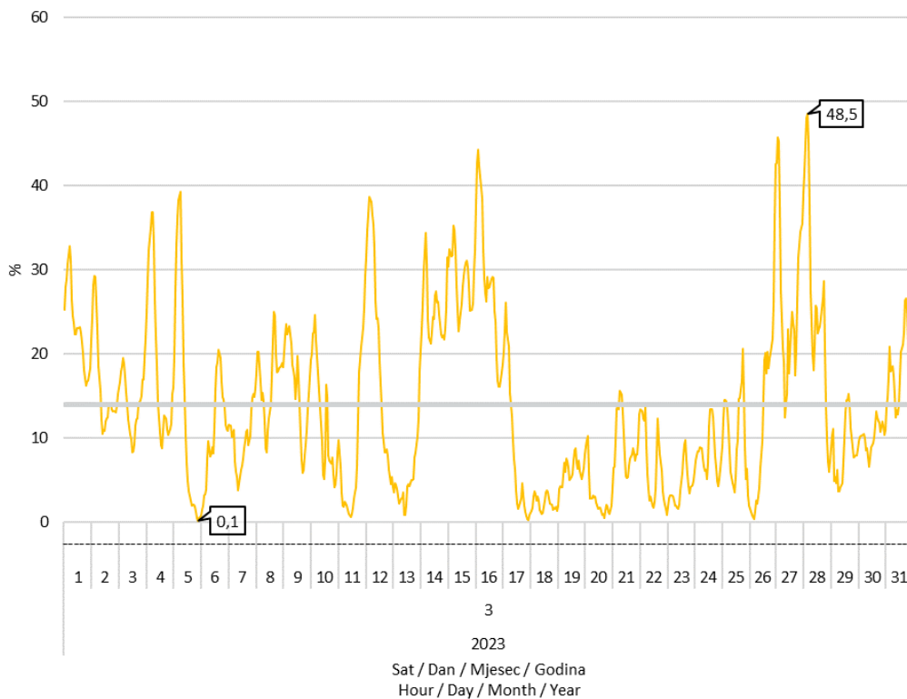
Slika 8 Udio proizvodnje vjetroelektrana u pokrivanju satnog opterećenja elektroenergetskog sustava u ožujku 2023. godine
