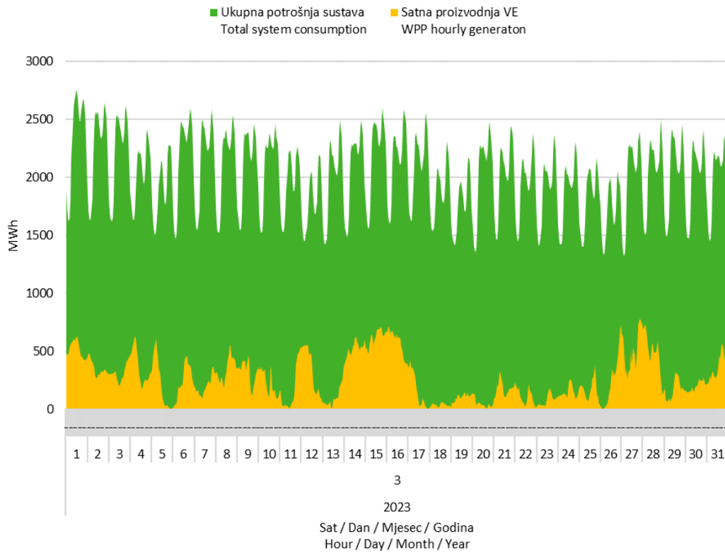
Slika 7 Usporedba satnog dijagrama opterećenja sustava i proizvodnje vjetroelektrana u ožujku 2023. godine
