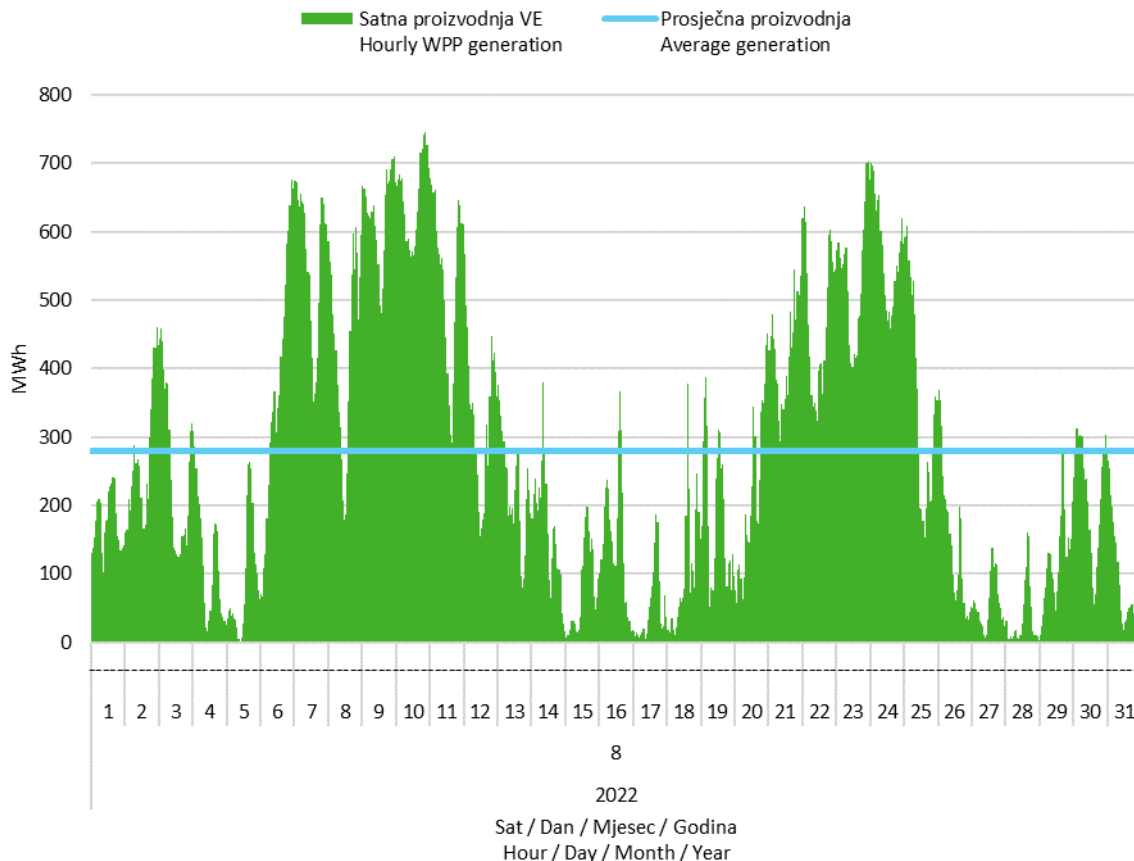
Slika 2 Satna proizvodnja svih vjetroelektrana u kolovozu 2022. godine
