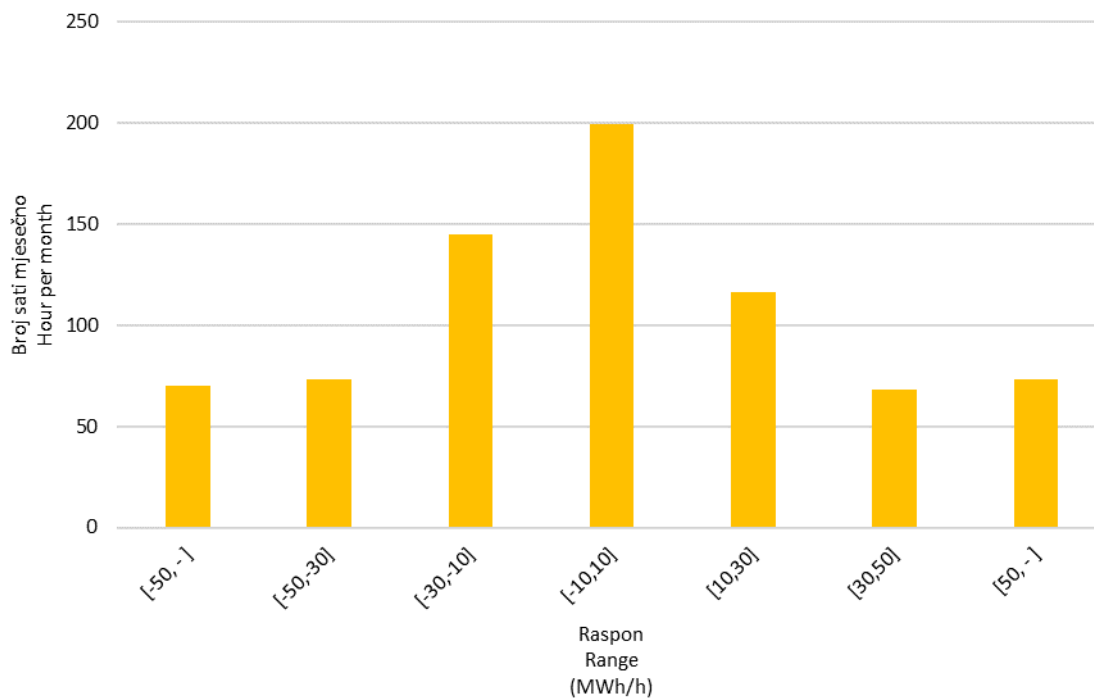
Slika 10 Statistička raspodjela satnih promjena proizvodnje VE u kolovozu 2022. godine
