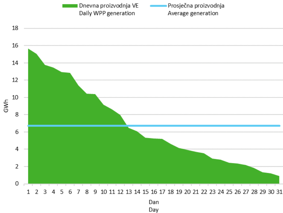
Slika 6 Krivulja trajanja dnevne proizvodnje vjetroelektrana u kolovozu 2022. godine
