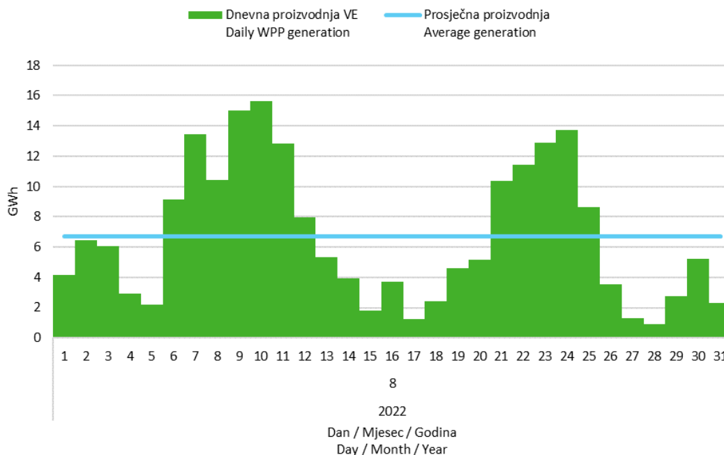
Slika 5 Dnevna proizvodnja svih vjetroelektrana u kolovozu 2022. godine
