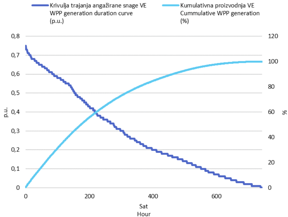
Slika 3 Krivulja trajanja angažirane snage svih VE i kumulativna proizvodnja VE u kolovozu 2022. godine u jediničnim vrijednostima
