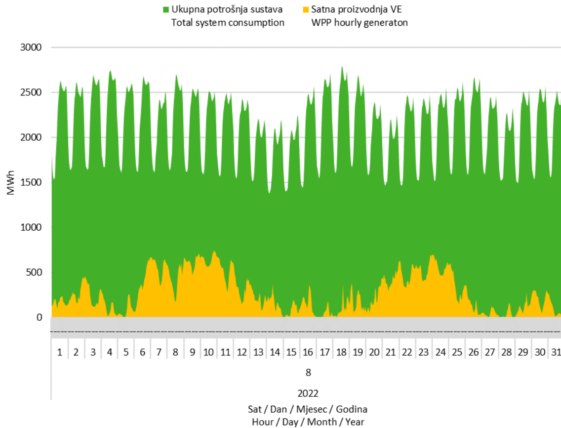
Slika 7 Usporedba satnog dijagrama opterećenja sustava i proizvodnje vjetroelektrana u kolovozu 2022. godine
