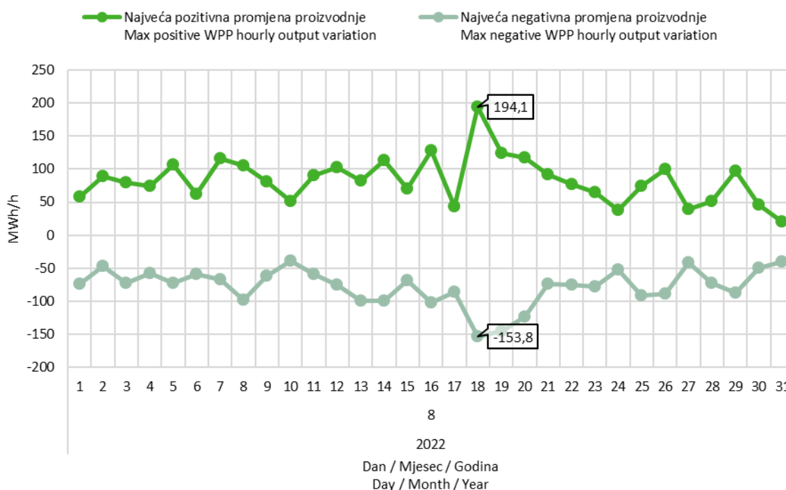
Slika 9 Maksimalna pozitivna i maksimalna negativna promjena satne proizvodnje VE u kolovozu 2022. godine
