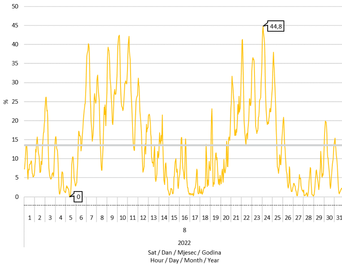
Slika 8 Udio proizvodnje vjetroelektrana u pokrivanju satnog opterećenja elektroenergetskog sustava u kolovozu 2022. godine
