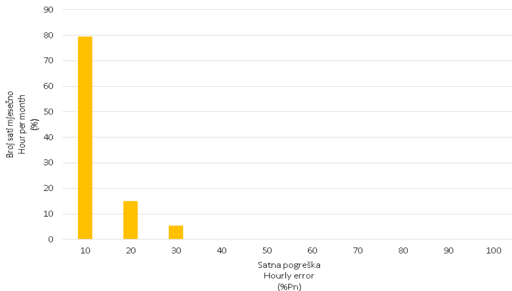
Slika 17 Frekvencija pojavljivanja pogreške prognoze satne proizvodnje svih VE u srpnju 2016. godine
