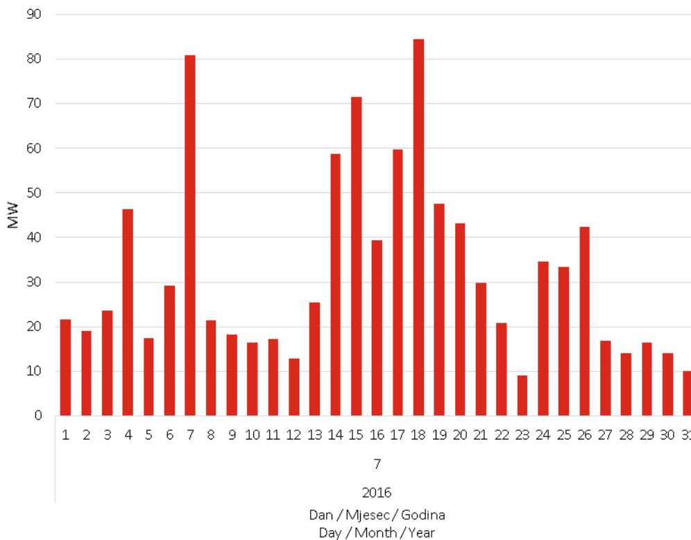
Slika 15 Korijen srednje kvadratne pogreške prognoze satne proizvodnje svih VE u srpnju 2016. godine
