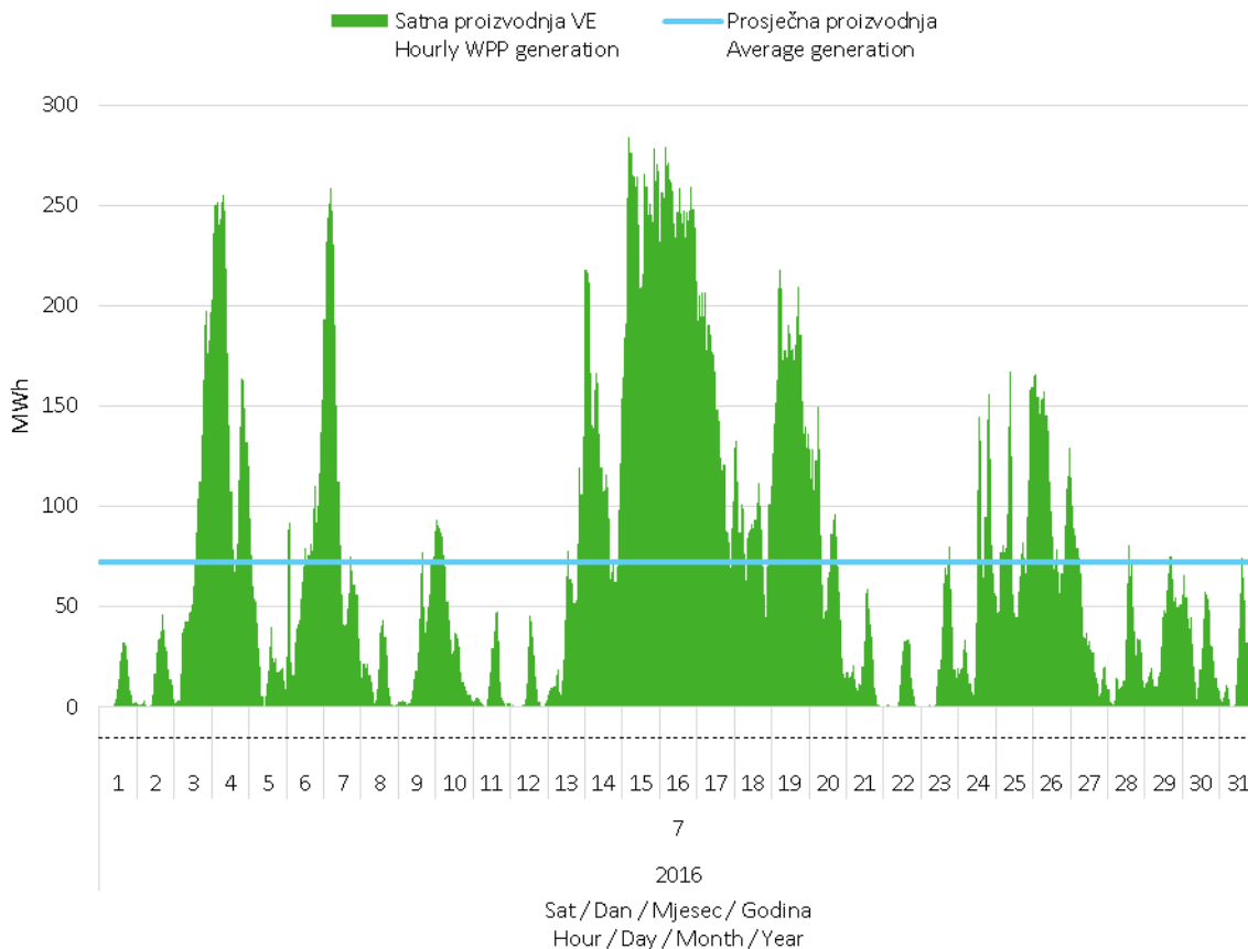
Slika 2 Satna proizvodnja svih vjetroelektrana u srpnju 2016. godine
