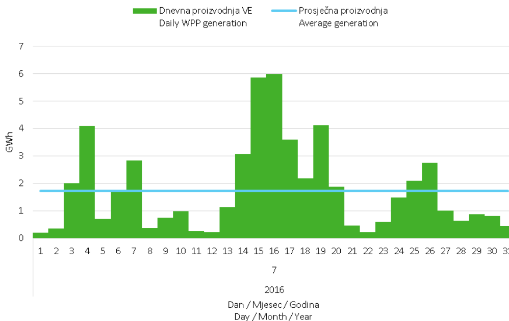
Slika 5 Dnevna proizvodnja svih vjetroelektrana u srpnju 2016. godine
