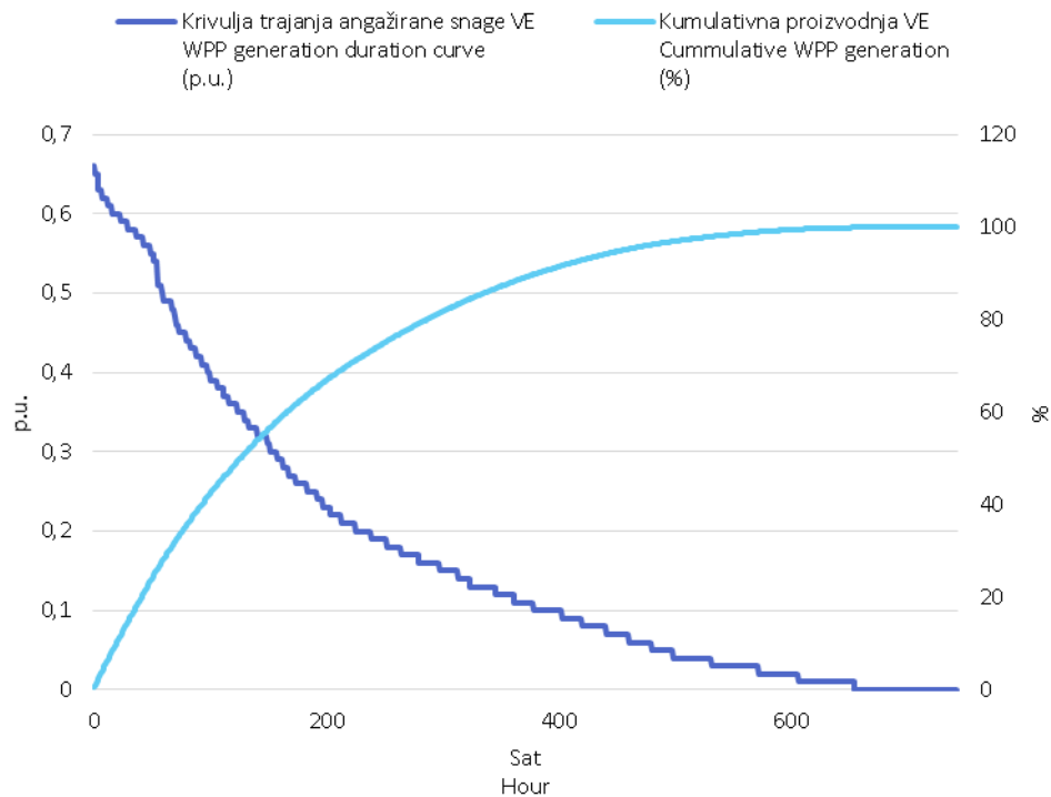
Slika 3 Krivulja trajanja angažirane snage svih VE i kumulativna proizvodnja VE u srpnju 2016. godine u jediničnim vrijednostima
