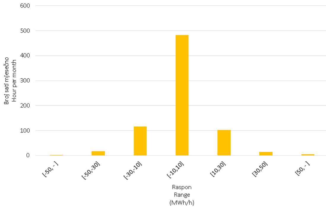
Slika 10 Statistička raspodjela satnih promjena proizvodnje VE u srpnju 2016. godine
