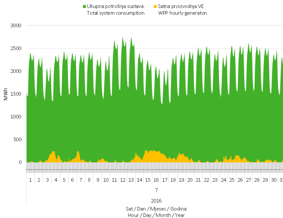
Slika 7 Usporedba satnog dijagrama opterećenja sustava i proizvodnje vjetroelektrana u srpnju 2016. godine
