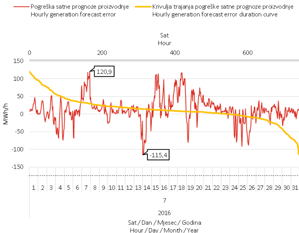
Slika 12 Razlika između prognozirane i ostvarene satne proizvodnje svih VE (pogreška prognoze) i pripadna krivulja trajanja u srpnju 2016. godine
