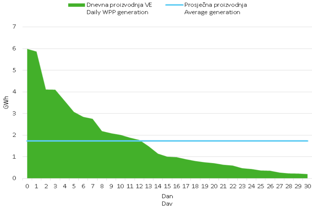
Slika 6 Krivulja trajanja dnevne proizvodnje vjetroelektrana u srpnju 2016. godine
