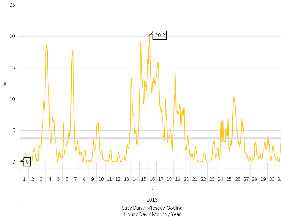
Slika 8 Udio proizvodnje vjetroelektrana u pokrivanju satnog opterećenja elektroenergetskog sustava u srpnju 2016. godine
