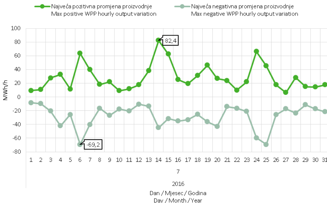
Slika 9 Maksimalna pozitivna i maksimalna negativna promjena satne proizvodnje VE u srpnju 2016. godine
